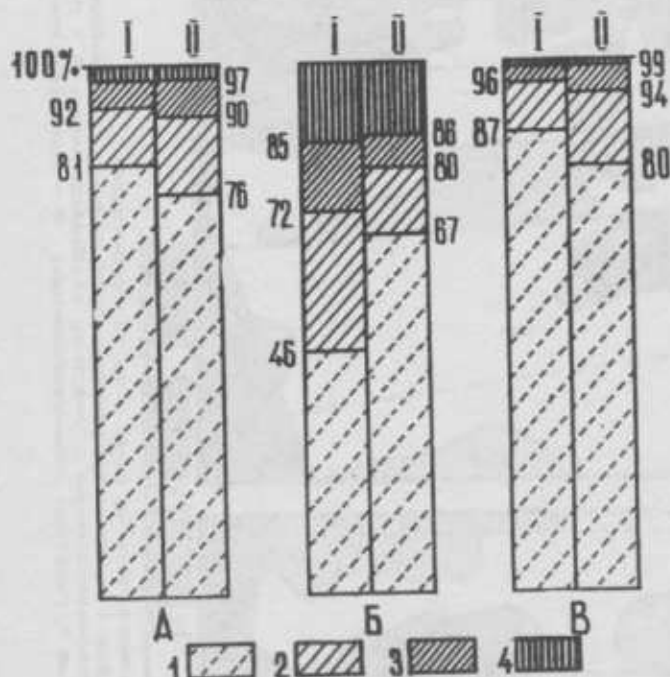
Рис. 20. Сравнение площадей почв различного засоления, подсчитанных по картам 1975 и 1986 гг. по основным почвенно-литолого-геоморфологическим районам Голодной степи:
