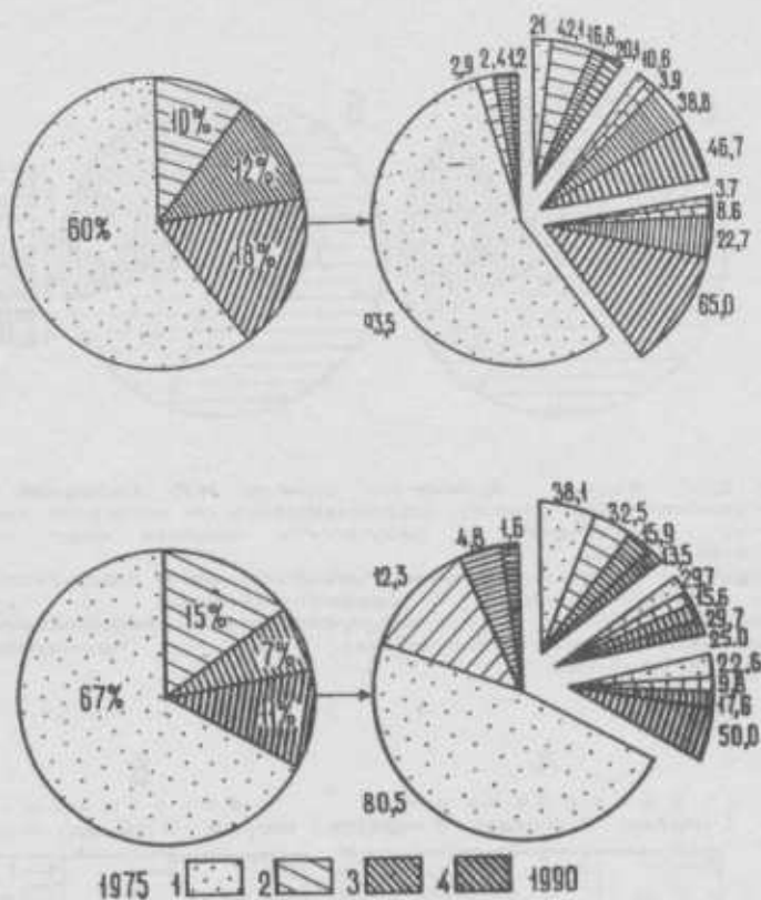
Рис. 24. Направление солевого процесса в землях НЗО Голодной (А) и Джизакской (Б) степей при различном исходном засолении почвы.
