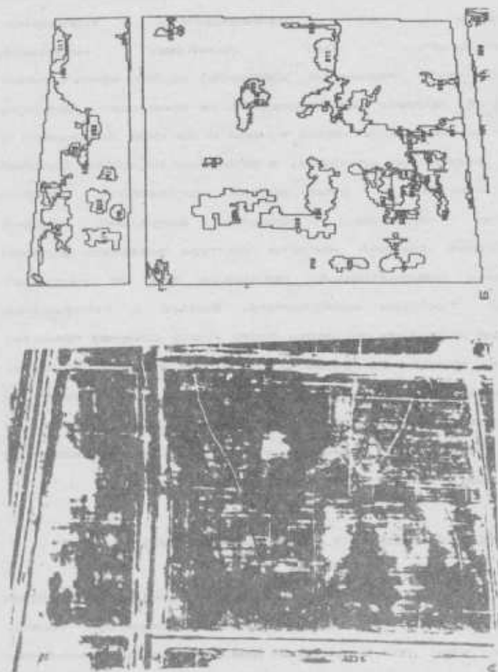
Рис. 34. Фрагмент панораматического аэрофотоснимка масштаба 1:110000 (А) и результат его лазерного дешифрирования в интерактивном режиме (Б)
