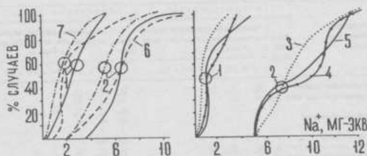
Рис. 10. Характеристика засоления почв неоднородных по фото-изображению контуров: 1 - тенные компоненты контуров; 2 - светлые.
