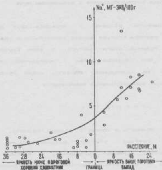
Рис. 29. Зависимость средневзвешенного засоления почвы в слое 0–100 см от расстояния до границы ближайшего выппада (после корректировки фотонизображения и включения скважин, заложённых в контурах выпадов)
