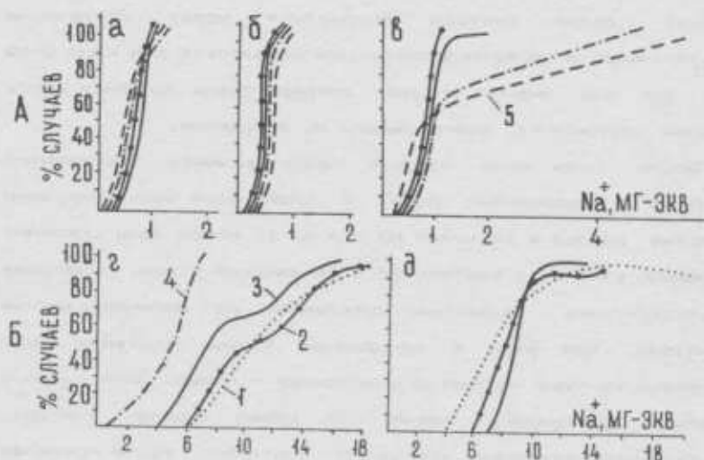
Рис.9. Характеристика засоления почв однородных (однотонных) по фотонизображению темных (А) и светлых (Б) контуров по слоям: 1 - 0-25см; 2 - 0-50см; 3 - 0-100см; 4 - 100-200см; 5 - 200-300см. Участки: а - 5м; б - 6м; в - 8м; г - 29м; д - 30м
