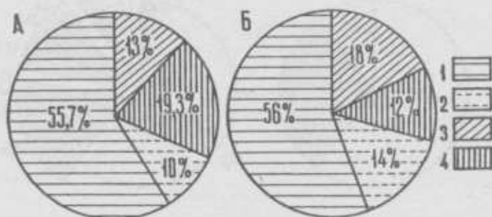
Рис. 22. Баланс орошаемых земель НЗЗ Голодной (А) и Движаской (Б) степей, различавшихся по динамике засоления почв, полученный в результате анализа карт динамики засоления почв.
