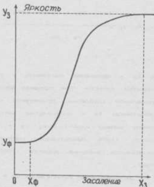
Рис. 2В. Принципиальный вид зависимости яркости фотонизображения от засоления почвы: X_f — минимальное засоление, приводящее к угнетению хлопчатника; X_z — максимальное засоление, при котором происходит полный выпад растений; Y_f — яркость при 100%-ном проективном покрытии хлопчатника; Y_z — яркость при полном отсутствии растений (100% открытой поверхности почвы)
