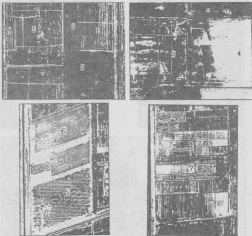
Рис. 12. Фотоизображение различных сельскохозяйственных культур на раннеосенних аэрофотоснимках масштаба 1:100000: 1 - хлопчатник; 2 - кукуруза; 3 - лецерна; 4 - лецерна скошенная; 5 - сады; 6 - виноградники; 7 - бакчи, огороды
