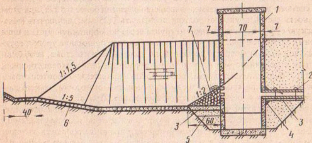
Рис. 1. Дренажный фильтр конструкции I:
