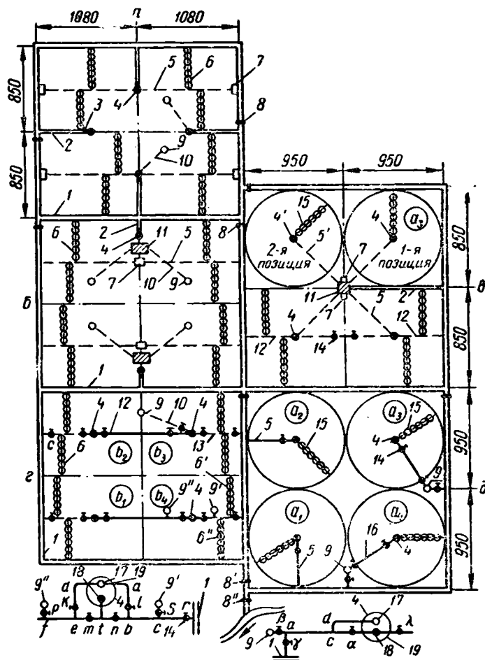
Рис. 63. Схемы осушительно-оросительных систем вертикального дренажа:
