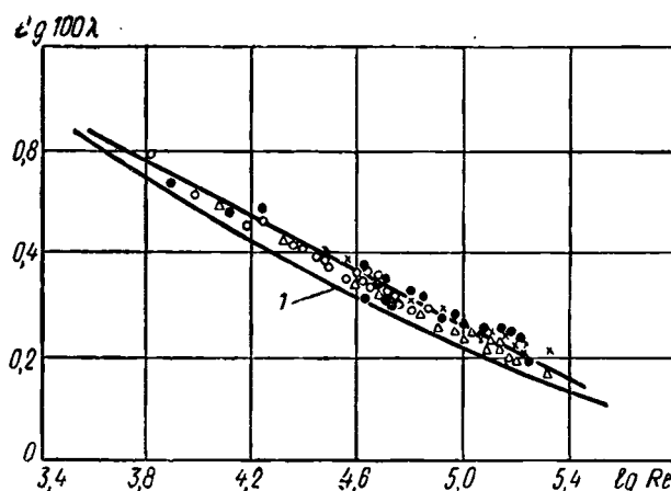
Рис. 34. Зависимость \lg 100\lambda = f(\lg Re) для гладкостенных труб из НПВХ:
