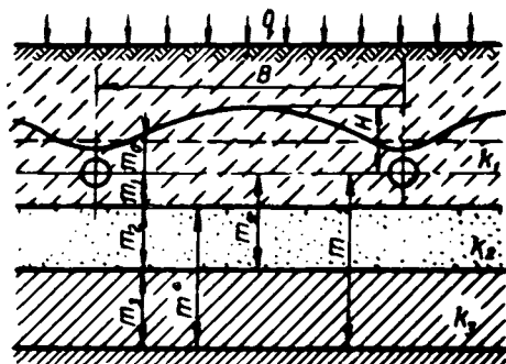
Рис. 24. Расчетная фильтрационная схема дренажа в трехслойном грунте.
