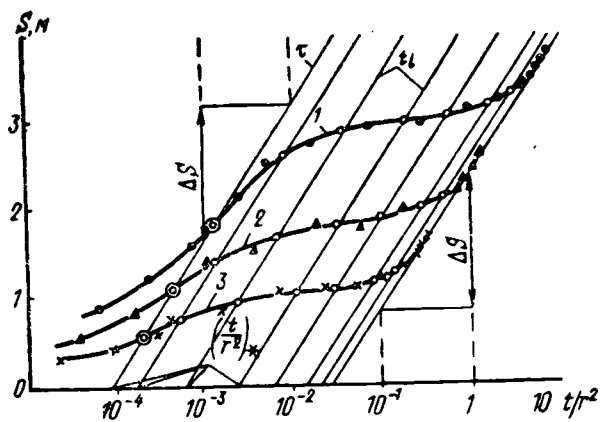
Рис. 73. Способ определения коэффициента расчетной водоотдачи по графику комбинированного прослеживания понижения уровня.
