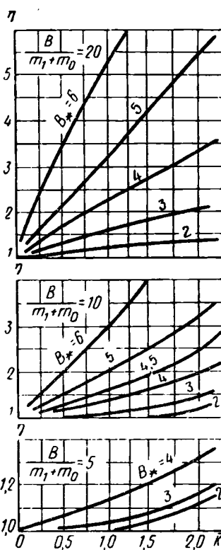
Рис. 30. Зависимость \eta = f(B/m_*, \bar{k}, B_*) .
