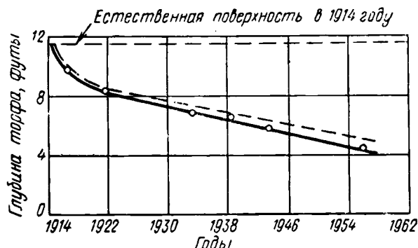
Рис. 55. Зависимость осадки торфа от времени (по Р. Эллисону).
