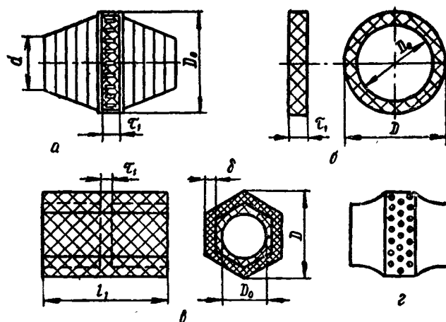
Рис. 54. Схемы соединительных деталей фильтров для керамического дренажа:
