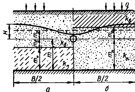
Рис. 25. Расчетная фильтрационная схема дренажа в двухслойном грунте: а — при колебании УГВ в верхнем слое; б — то же, преимущественно в нижнем.
