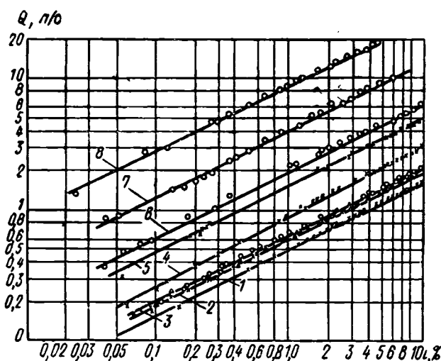
Рис. 36. Зависимость Q=f(100i) гофрирования труб из ПЭВП конструкции БелНИИМВиХ (○) НИИПМ(х) (по А. И. Митраховичу): 1 — D=42,2 мм; 2 — D=45,4 и 46,7 мм; 3 — D=44,6 мм; 4 — D=54 мм; 5 — D=65 мм; 6 — D=73,9 мм; 7 — D=91 мм; 8 — D=119 мм.
