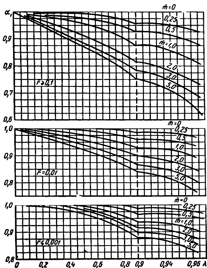
Рис. 27. Зависимость \alpha_1 = f(\lambda, \bar{r}, \bar{m}) .
