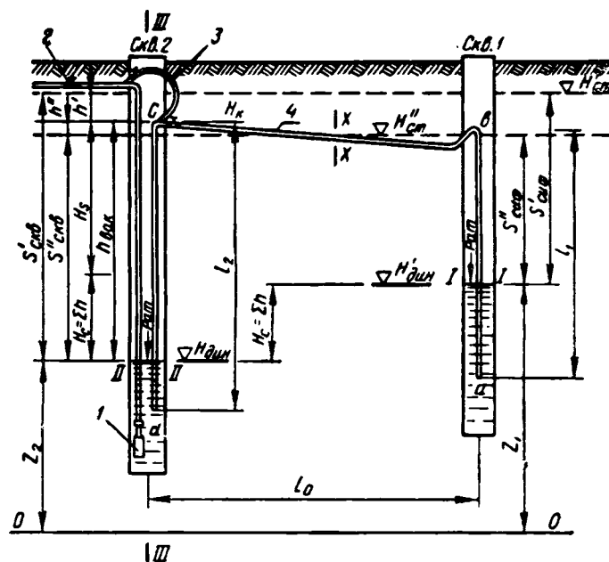
Рис. 75. Схема сифонного устройства:
