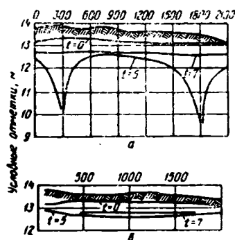
Рис. 80. Положение УГВ по створам В—В (а) и А—А (б) до откачки ( t=0 ), в конце пятистрочной откачки из четырех скважин ( t=5 ) и спустя двое суток после прекращения откачки ( t=7 ).
