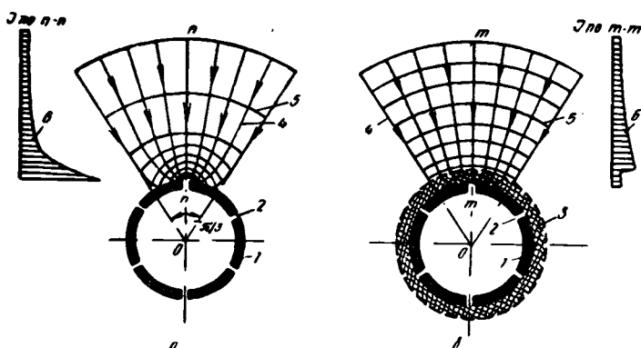
Рис. 16. Схемы движения воды к дренажным пластмассовым трубам:
