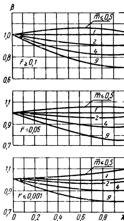
Рис. 26. Зависимость \beta=f(\lambda, \bar{r}, \bar{m}) .
