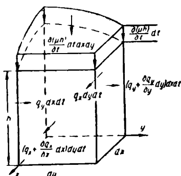
Рис. 21. Балансовая модель элементарного объема.
