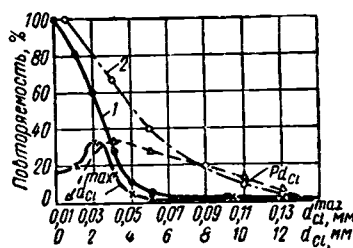
Рис. 45. Распределение суффозионных частиц в несвязных осушаемых грунтах в БССР:
