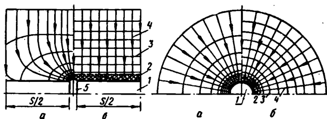
Рис. 5. Схемы движения воды к дрене из керамических труб: а — без фильтра; б — с фильтром; 1 — труба; 2 — фильтр; 3 — линии равных напоров; 4 — линии тока; 5 — стыковой зазор между трубами.
