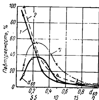
Рис. 44. Распределение сводообразующих ( d_{60} ) частиц и коэффициентов неоднородности ( \eta ) осушаемых несвязных грунтов в БССР:
