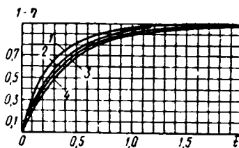
Рис. 32. Зависимость \bar{t}=f(\eta, \eta_m) : 1 — при \eta_m=0.5 ; 2 — при \eta_m=1 ; 3 — при \eta_m=2 ; 4 — при \eta_m \geq 3 (по С. Ф. Аверьянову).
