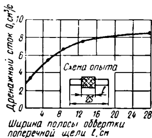
Рис. 49. Влияние на сток ширины защитной полосы стеклохолста, уложенного над поперечной щелью в дрене.
