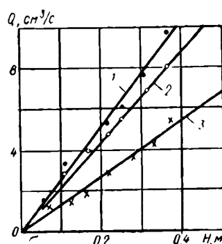
Рис. 48. Зависимость Q=f(H) для керамической дрены (одностыковой зазор \tau_1=2 мм): 1 — с фильтром из стеклохолста толщиной 1 мм; 2 — с фильтром из песчано-гравийной смеси толщиной 25 мм; 3 — без фильтра.
