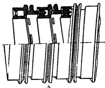
Рис. 11. Схема спиральнонавитой дренажной трубы из НПВХ.
