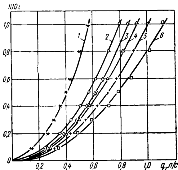
Рис. 39. Зависимость q=f(100i) для различных труб: 1, 2, 4 — гончарных по формулам (185), (190), (192); 3 — гофрированных по формуле (216); 5 — спиральнонавитых по формуле (227); 6 — гладкостенных по формуле (213).
