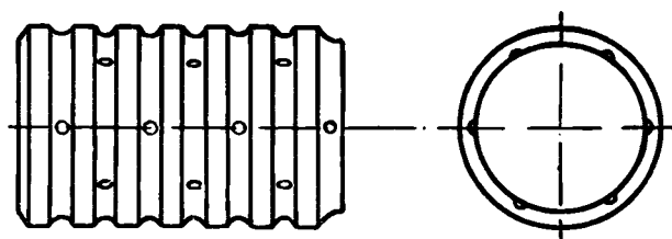
Рис. 10. Схема гофрированной дренажной трубы из ПЭВП.
