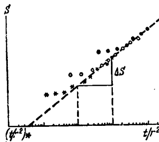
Рис. 71. График комбинированного прослеживания понижения уровня S=f(t/r^2) .
