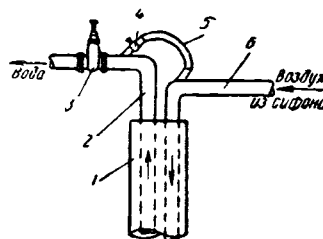
Рис. 76. Схема зарядного устройства сифона конструкции БелНИИМиВХ:
