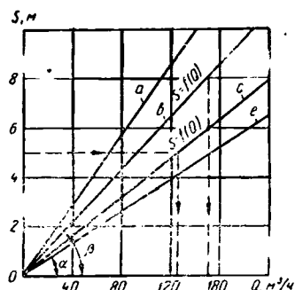
Рис. 77. Индикаторные кривые скважин S=f(Q) .
