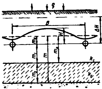
Рис. 29. Расчетная схема фильтрации при напорном питании.
