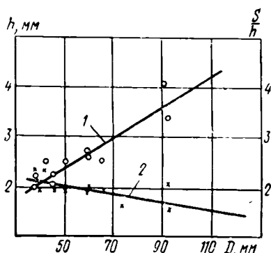
Рис. 37. Зависимость h=f(D) (1) и S/h=\varphi(D) (2) для гофрированных дренажных труб.
