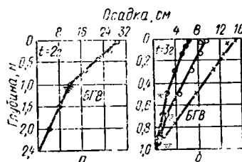
Рис. 57. Зависимость осадки торфа от его глубины и бытовых УГВ (эпюры осадки): а — объект «Поня»; б — монолиты №№ 2...4; (t — длительность осушения; БГВ — бытовой горизонт воды в торфе).
