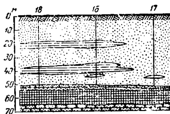
Рис. 78. Геологический разрез по створу В—В ПОМС.
