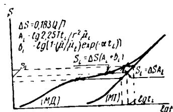
Рис. 64. График связи решения модели Довнара (МД) с решением модели Тейса (МТ).
