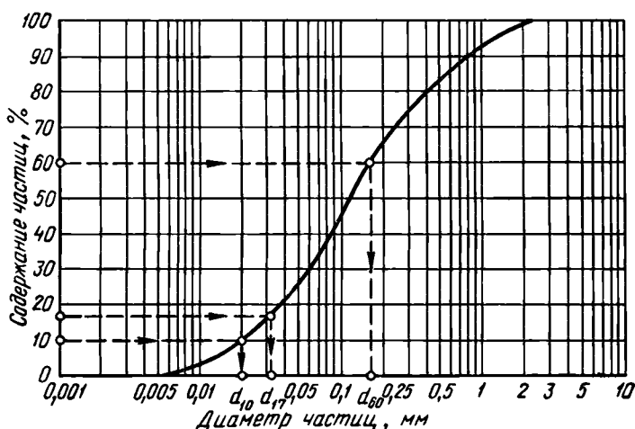
Рис. 40. График гранулометрического состава грунта.
