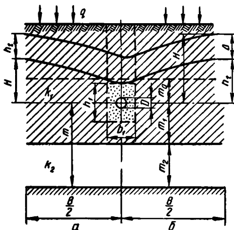
Рис. 33. Расчетная фильтрационная схема: а — по допустимому подъему УГВ; б — по заданному понижению.
