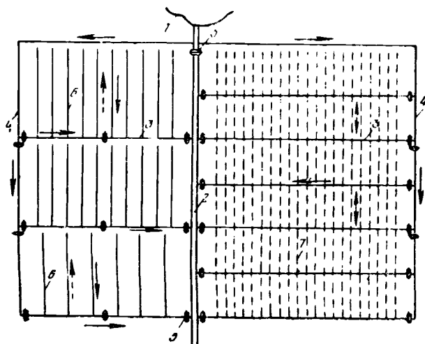
Рис. 2. Схема открытой осушительно-увлажнительной системы: 1 — водохранилище; 2 — магистральный канал; 3 — коллектор; 4 — распределитель; 5 — шлюз-регулятор; 6 — регулирующий канал; 7 — кротовые дрены.
