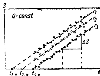
Рис. 69. График временного прослеживания понижения уровня S=f(t) .
