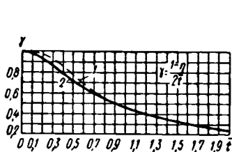
Рис. 31. Зависимость \bar{t}=f(\gamma) : 1 — при \eta=1 ; 2 — при \eta \geq 5 .
