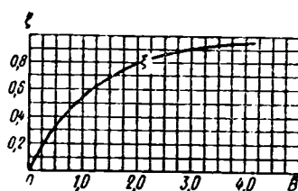
Рис. 28. Зависимость \xi = f(B) .
