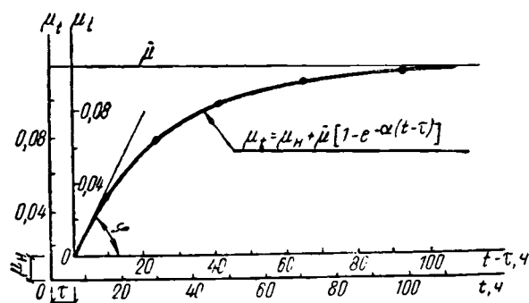
Рис. 74. График расчетной водоотдачи по данным кустовой откачки.
