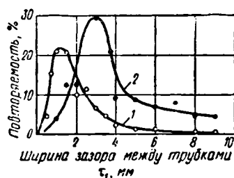
Рис. 42. Распределение величин стыковых зазоров между трубками керамического дренажа:
