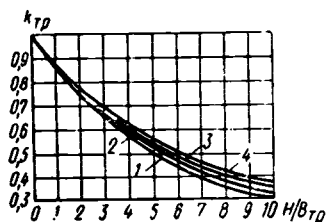
Рис. 14. Зависимость K_{тр} = \eta(H/B_{тр}) :
