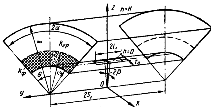
Рис. 17. Расчетная область фильтрации.
