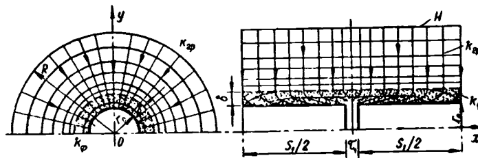
Рис. 8. Расчетная схема притока воды к дрене из керамических труб, уложенных с фильтром.
