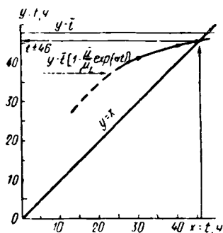
Рис. 65. Геометрическая интерпретация решения итерационного уравнения.
