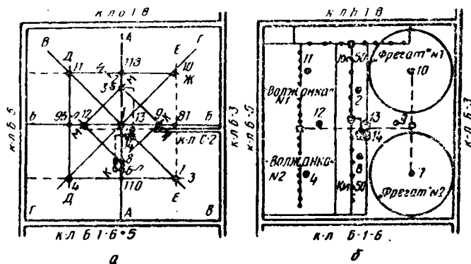
Рис. 79. Схема опытно-производственной осушительно-оросительной системы вертикального дренажа на ПОМС:
