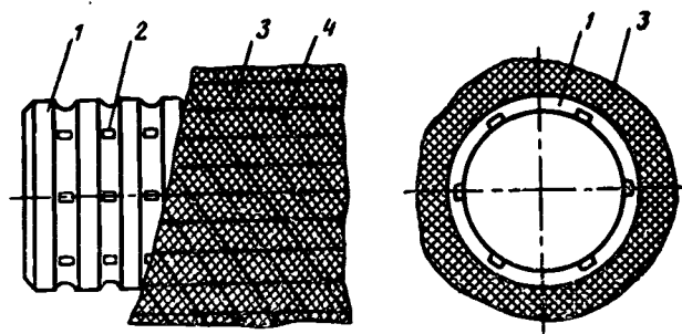
Рис. 9. Пластмассовая дренажная труба с объемным фильтром-оболочкой:
