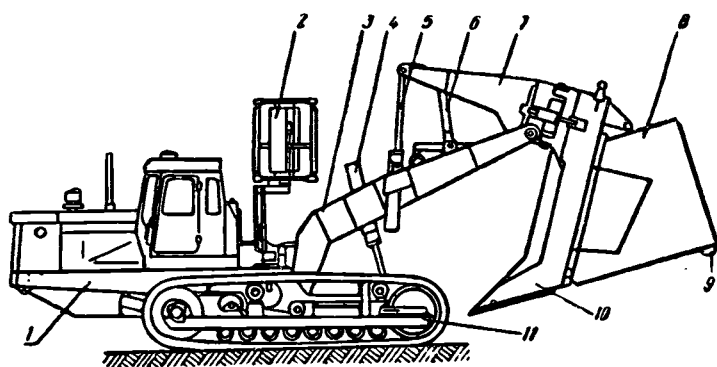
Рис. 19. Схема бестраншейного дренаукладчика МД-4:
