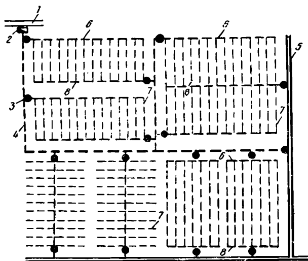
Рис. 3. Схема закрытой осушительно-увлажнительной системы: 1 — водоисточник; 2 — насосная станция; 3 — колодец с задвижкой; 4 — закрытый распределитель; 5 — магистральный канал; 6 — закрытый ороситель; 7 — дрены-увлажнители; 8 — сбросной коллектор.
