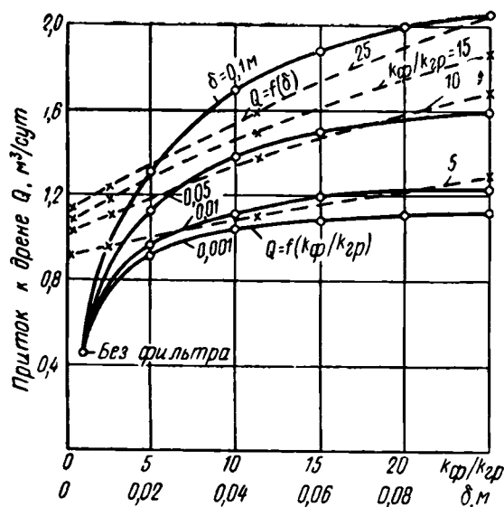
Рис. 50. Зависимости Q = f(k_\phi/k_{гр}, \delta = \text{const}) и Q = f(\delta, k_\phi/k_{гр} = \text{const}) для керамической дрены: S_1 = 0,33 м; \tau_1 = 0,002 м; r_0 = 0,036 м; k_{гр} = 1 м/сут; H = 0,5 м; R = 0,5 м; L = 1 м.
