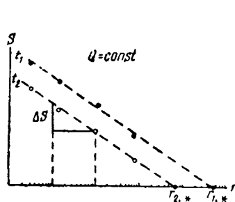
Рис. 70. График площадью прослеживания понижения уровня S=f(r) .
