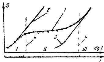
Рис. 68. Полулогарифмический график прослеживания уровней при откачках с безнапорных горизонтов:
