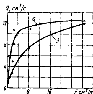
Рис. 47. Зависимость дренажного стока от площади перфорации полиэтиленовой дрены D=40 мм (по Е. Г. Сапожникову): а — с фильтром из стеклохолста; б — без фильтра.
