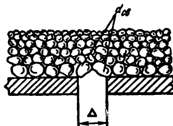
Рис. 43. Схема контактной области песчаного грунта и дренажной трубы:
