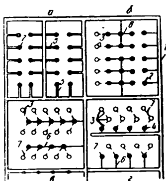
Рис. 61. Схемы систематического вертикального дренажа: 1 — каналы; 2 — дренажные скважины; 3 — сифонные водосборы; 4 — малodeбитные скважины или колодцы; 5 — мелкие сбросные каналы с противofильтрационными экранами в оголовках; 6 — напорные закрытые трубопроводы; 7 — сифонные трубопроводы.
