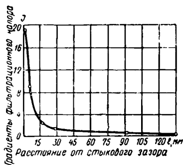
Рис. 41. Изменение градиентов фильтрационного напора вдоль керамической трубки (ширина зазора между трубками \tau = 1,1 мм, напор над дренаем H = 37 см).
