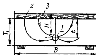
Рис. 52. Схема подрусовой дрены (лоток):
