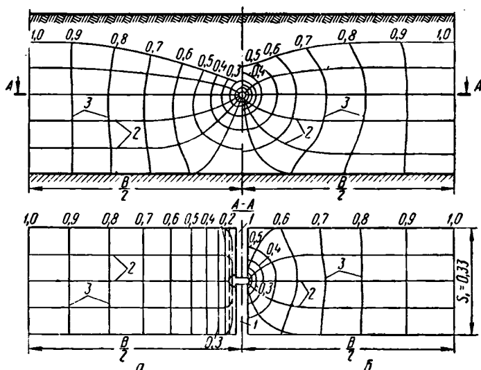
Рис. 46. Гидродинамическая сетка керамической дрены при боковом питании:
