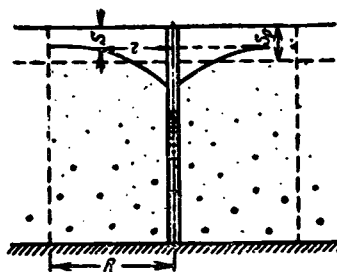
Рис. 67. Схема действия скважины в системе площадного дренажа.
