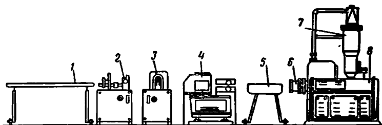
Рис. 12. Схема технологической линии для производства спиральнонавитых дренажных труб:
