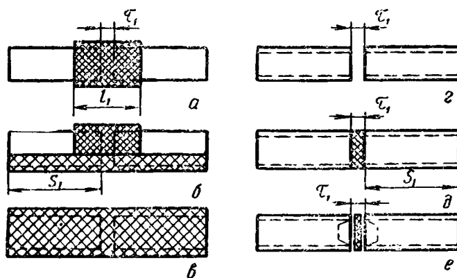
Рис. 53. Схемы укладки керамического дренажа:
