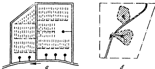
Рис. 62. Схемы комбинированного (а) и выборочного (б) вертикального дренажа.
