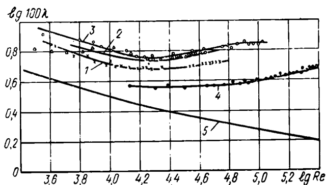
Рис. 35. Зависимость \lg 100\lambda = f(\lg Re) для гофрированных труб из ПЭВП конструкции БелНИИМиВХ (по А. И. Митраховичу):
