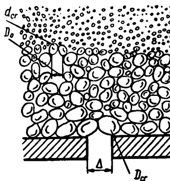
Рис. 51. Расчетная схема грунт — фильтр — дрена.
