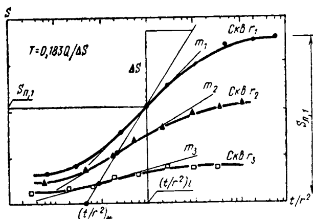
Рис. 72. График построения расчетной прямой для определения T по данным начального периода откачки.
