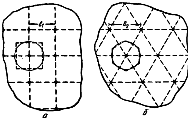
Рис. 66. Схемы расположения скважин при систематическом (площадном) вертикальном дренаже.
