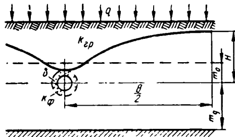
Рис. 23. Дрена в однородном грунте.
