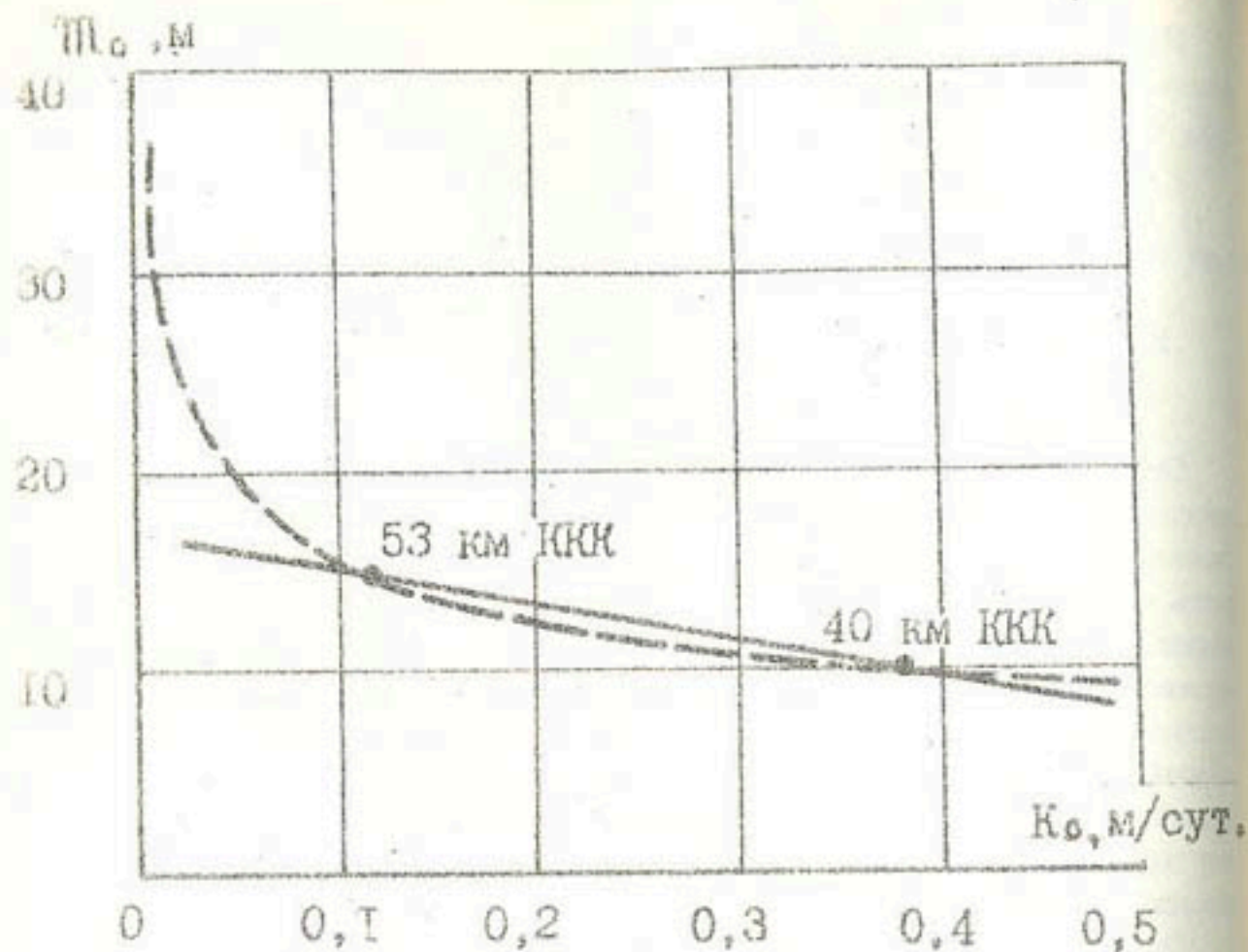
Рис. 3. Зависимость суммарной водопроницаемости песистой толщи от её мощности K_0 = f(m_0) .
