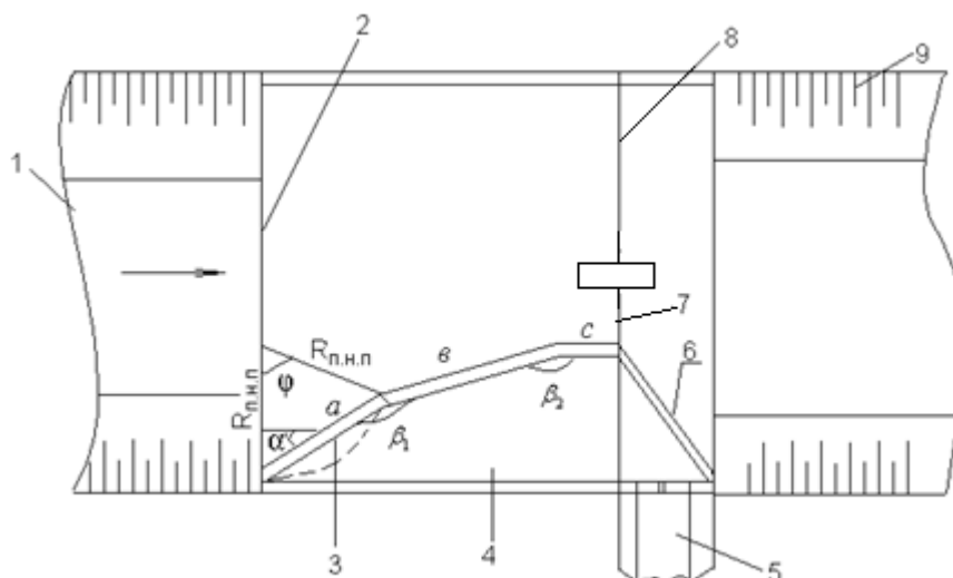
Рисунок 2.17 – Расчетная схема ломаного в плане наносазащитного порога: 1 – подводящее русло; 2 – входной створ; 3 – порог; 4 – водоприемная камера; 5 – отводящий канал; 6 – автоводослив; 7 – затвор промывника; 8 – затвор речного пролета; 9 – отводящее русло; а, в, с – секции порога; \alpha – угол между секцией а и динамической осью потока; \beta_1 и \beta_2 – углы между отдельными секциями
