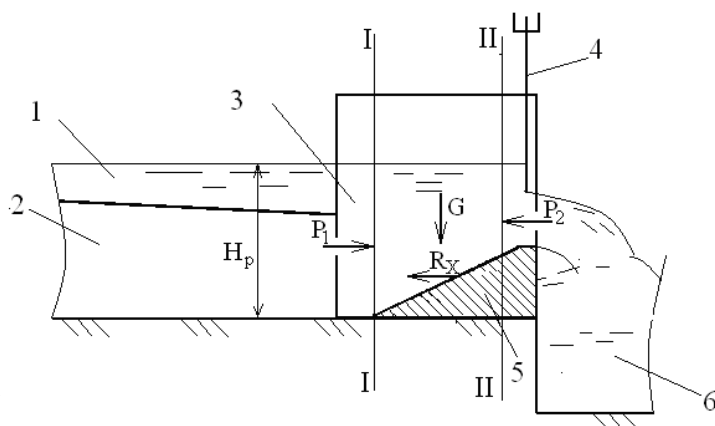
Рисунок 2.26 – Схема размещения донной вставки в промывном тракте: 1 – верхний бьеф; 2 – наносозащитный порог; 3 – промывной тракт; 4 – затвор промывного тракта; 5 – донная вставка; 6 – отводящее русло
