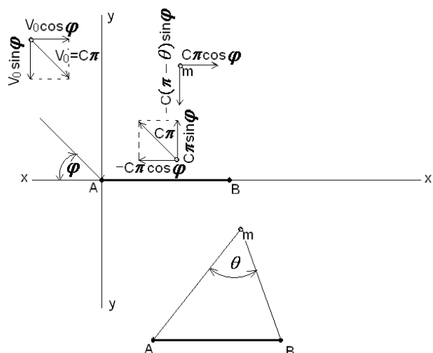
Рисунок 2.18 – Расчетная схема А.Я. Миловича к определению величин и направлений векторов скоростей жидкости в вихревых поверхностях, проявляющихся при косом набегающем потоке на плоскую пластинку. АВ – плоская пластинка; \varphi – угол набегающего потока; V_0 – скорость набегающей жидкости; C\pi – скорость распространения вихревых поверхностей; m – точка рассмотрения пластинки АВ; \theta – угол, под которым рассматривается пластинка
