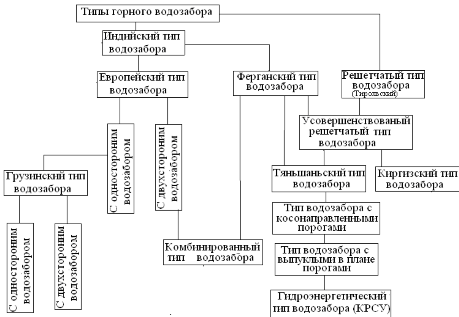
Рисунок 1.32 – Классификация типов низконапорных плотинных водозаборных сооружений на горных реках
