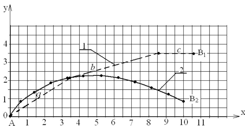
Рисунок 2.23 – Контур внешнх поверхностей наносозащитных порогов: 1 – исследуемый трехсекционный ломаный в плане наносозащитный порог; 2 – контур наносозащитного порога, построенный с использованием уравнений (2.68)
