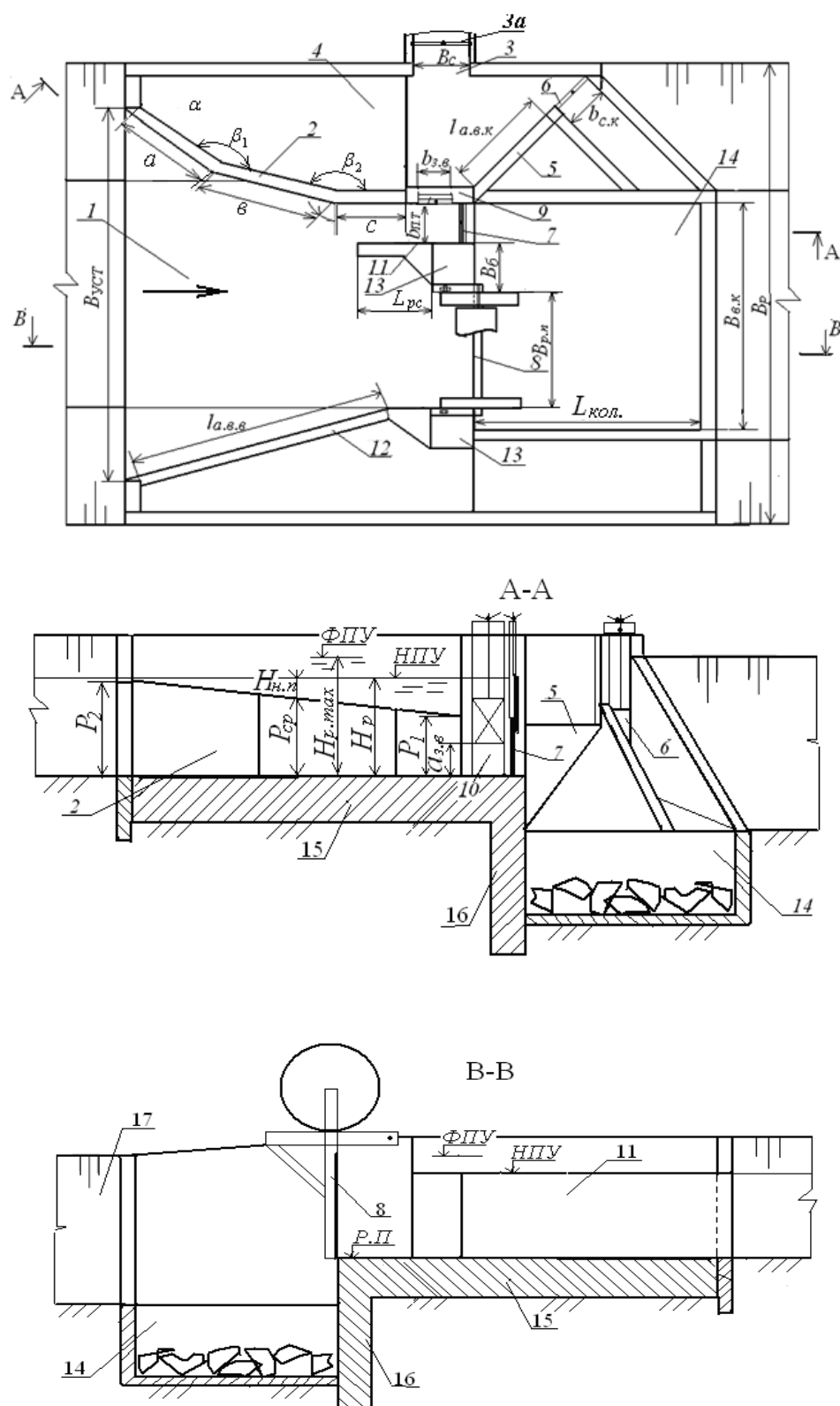
Рисунок 4.1 – Схема модели ВСДГ: 1 – верхний бьеф; 2 – наносозащитный порог; 3 – водоприемник; 3а – регулятор расхода отводящего канала; 4 – водоприемная камера; 5, 12 – автоводослив; 6 – сбросное отверстие; 7 – сдвоенный затвор промывника; 8 – затвор речного пролета; 9 – разделительная стенка; 10 – затвор зимнего водозабора; 11 – промывной тракт; 13 – быки; 14 – водобойный колодец; 15 – понур; 16 – зуб флютбета; 17 – отводящее русло
