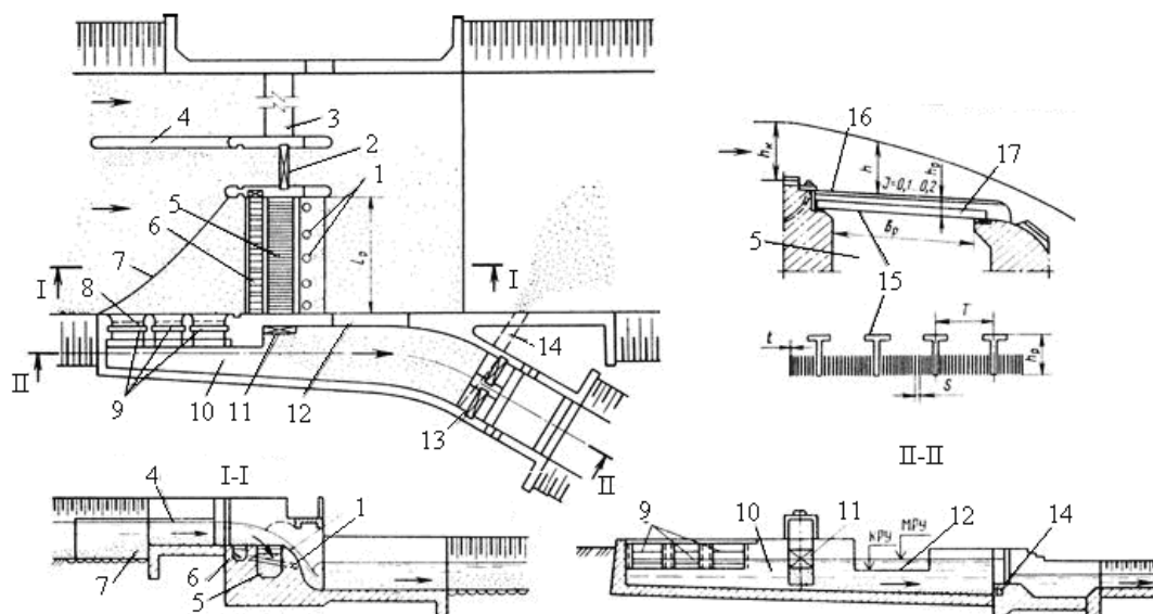
Рисунок 1.25 – Водозаборное сооружение решетчатого типа: 1 – пульповоды, 2 – щитовое отверстие; 3 – паводочная плотина; 4 – разделяющая стенка; 5 – водозаборная галерея; 6 – наносоперехватывающая траншея; 7 – криволинейный порог; 8 – сороудерживающие решетки; 9 – шандоры зимних водоприемников; 10 – аванкамера; 11 – отверстие водозаборной галереи; 12 – автоводослив; 13 – затворы головного регулятора; 14 – промывная галерея; 15 – решетка водозаборной галереи; 16 – верхняя решетка; 17 – мелкая решетка
