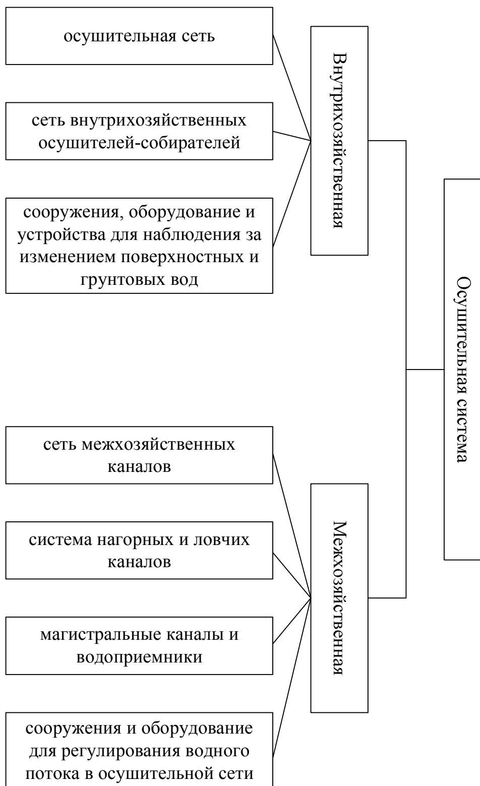
Рисунок 28 – Состав осушительной системы согласно В. А. Шаумяну
