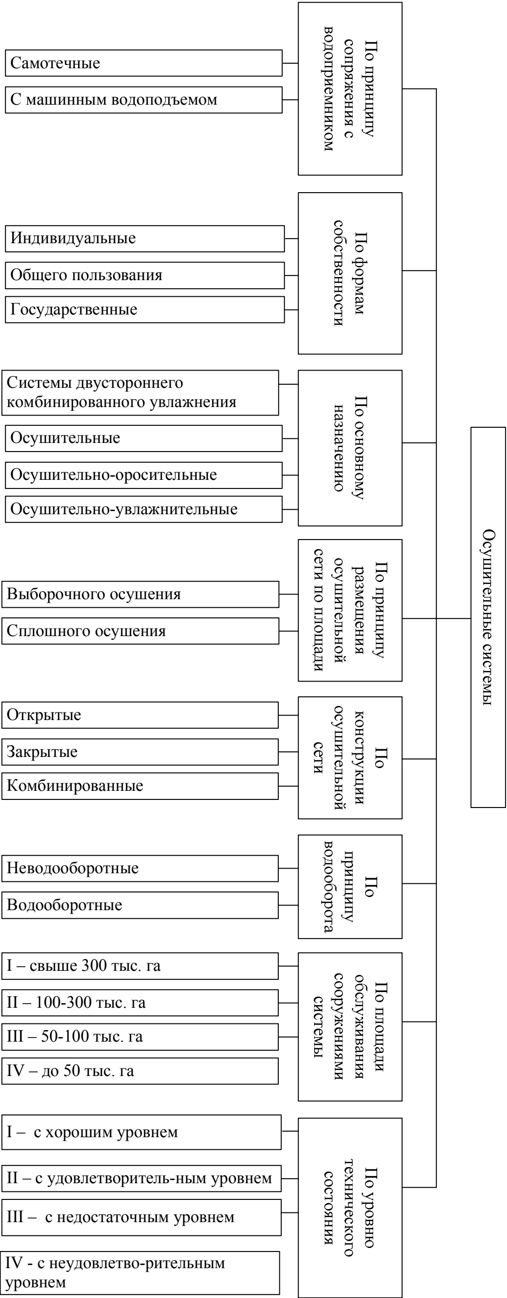
Рисунок 37 – Классификация осушительных систем
