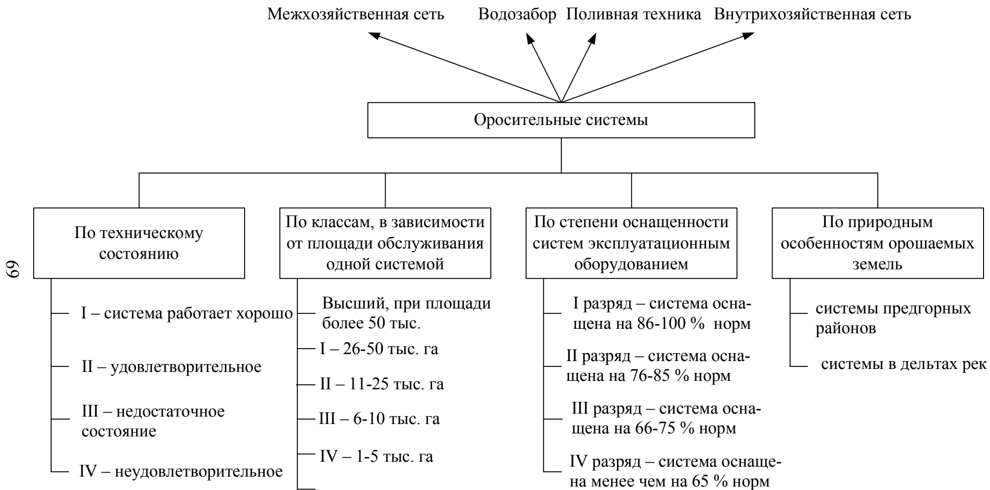
Рисунок 14 – Классификация и элементы оросительных систем согласно М. Ф. Натальчук
