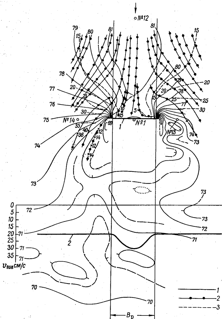
Рис. 1.2. Горизонталы поверхности воды (1), траектории (2) и плановые изотахи (3) потока при Q=15,2 л/с и \frac{B_p}{B_n} = \frac{1}{7,8} .
