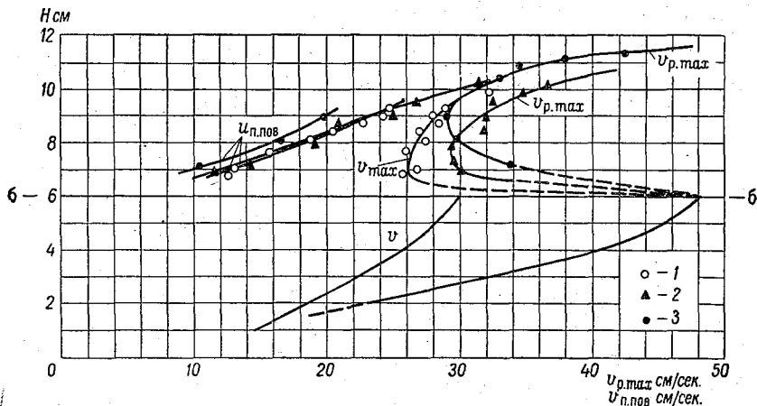
Рис. 10-12. Зависимость скоростей v_{p. \max} и v_{п. пов} от уровня воды (опыты 1948 г., вторая шероховатость поймы).
