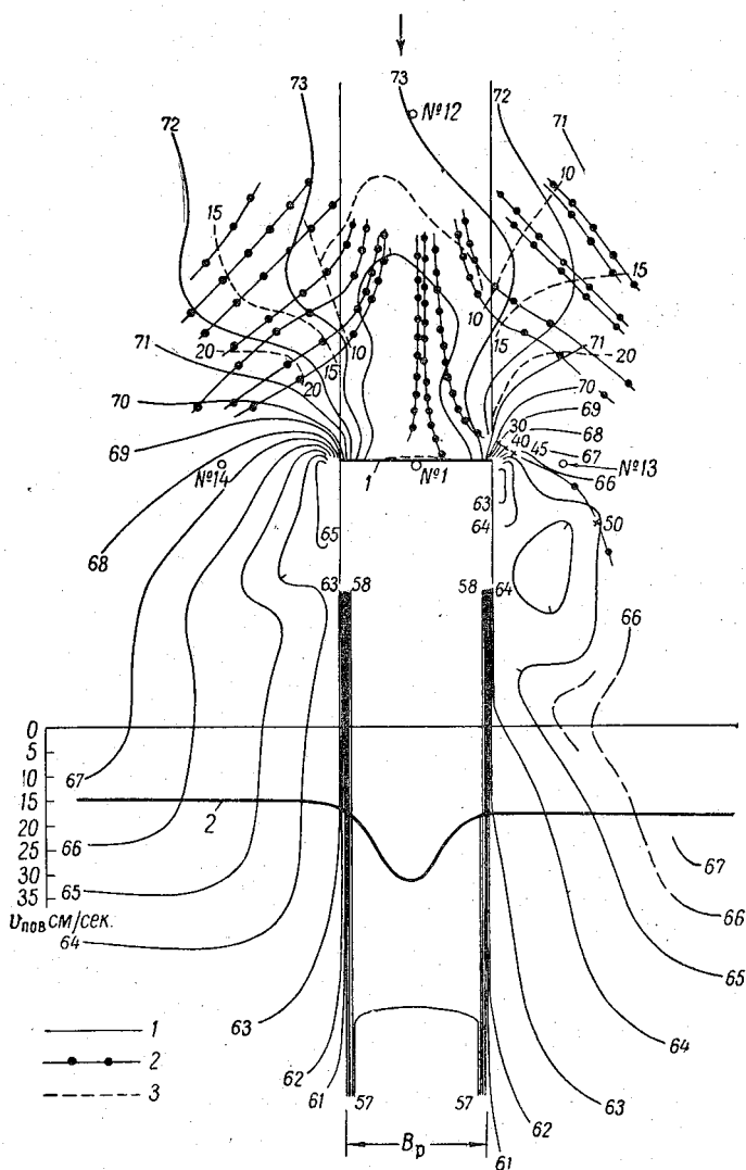
Рис. 1-2. Горизонталы поверхности воды (1), траектории (2) и плановые изотехи (3) потока при Q = 7,1 л/сек. и \frac{B_p}{B_n} = \frac{1}{7,8} .
