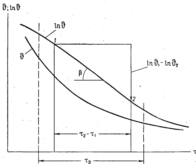
Рис. 6-10. График функции \Theta = \Theta(\tau) в обычных и полулогарифмических координатах.
