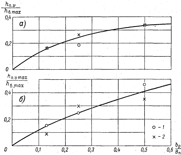
✓ Рас. 10-13. Зависимость глубины h_{п. в} (а) и h_{п. в тах} (б) от \frac{b_p}{B_p} . 1 — вторая шероховатость поймы; 2 — первая шероховатость поймы.
