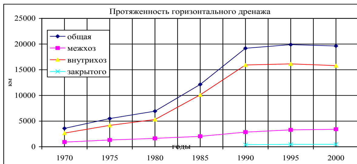
Рис. 6.5.1.3 Изменение протяженности КДС
