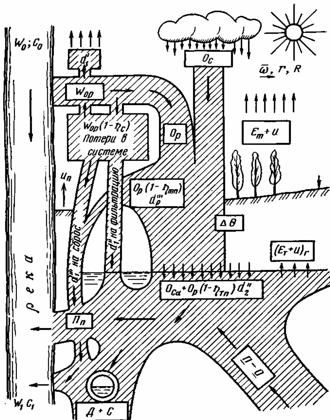
Рис.3.2. Взаимодействие оросительных вод на массиве орошения
