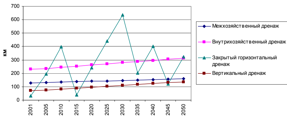
Протяженность реконструируемой дренажной сети
