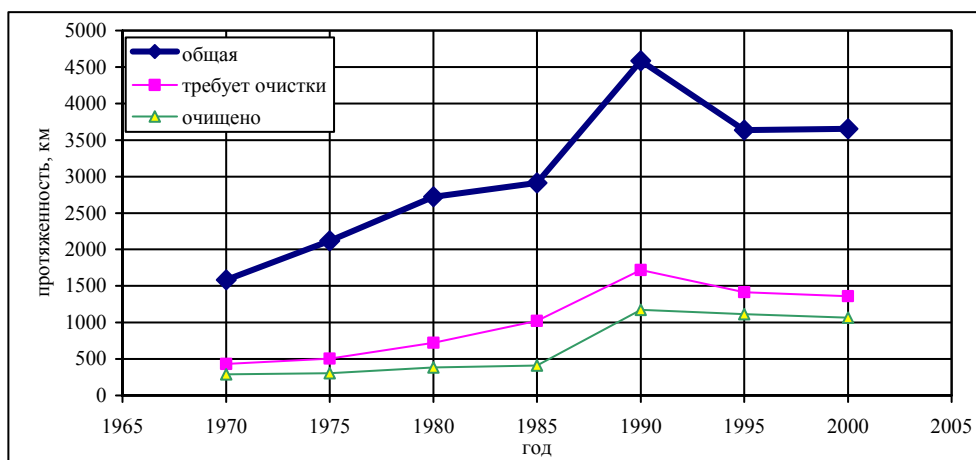
Рис. 6.2.1.6 Состояние внутрихозяйственного открытого дренажа
