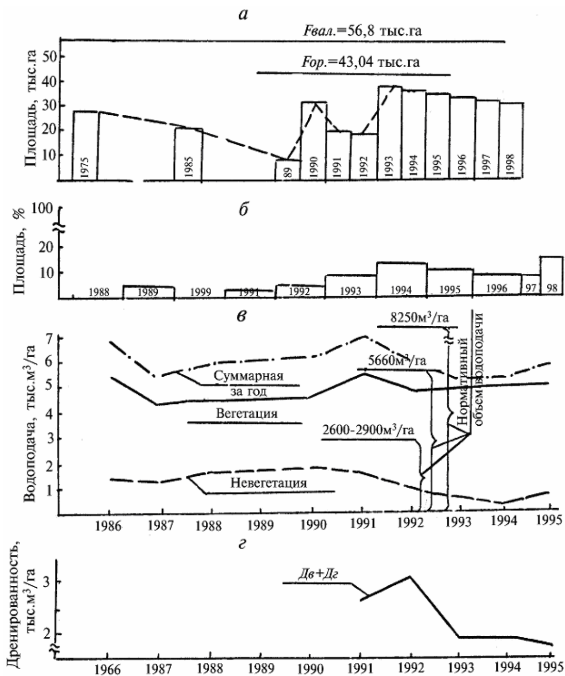
Рис. 6.4.1.4 Динамика показателей мелиоративной обстановки на Юго-Восточном массиве первой очереди а – незасоленные и слабозасоленные площади; б – площади с глубиной УГВ 0-2 м; в – водоподача «нетто-поле»; г – дренажность (на валовую площадь)
