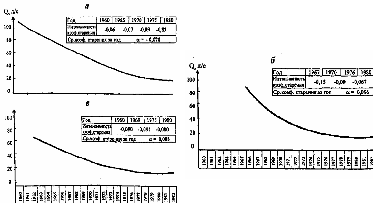
Рис.5.5. Изменение дебита скважин в процессе физико-химического колюматажа в зависимости от продолжительности их работы при: а – карбонатизации; б – коррозионных явлениях; в – смешанных процессах
