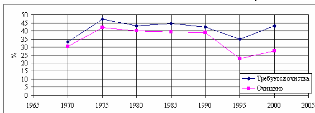
Рис. 6.3.1.6 Состояние межхозяйственных коллекторов
