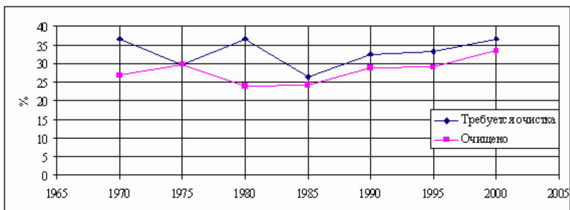
Рис. 6.3.1.4 Состояние межхозяйственных коллекторов
