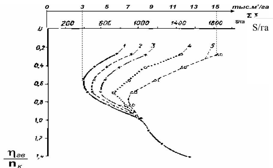
Рис.2.2. Оптимизация мелиоративного режима по сумме приведенных затрат с учетом воды и урожая:
