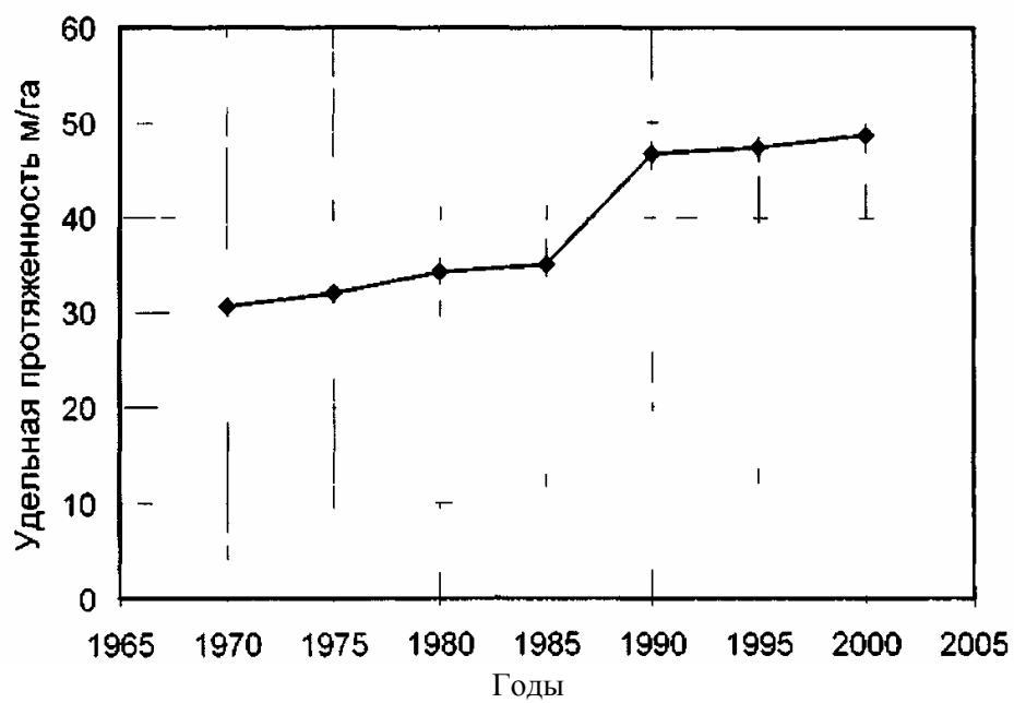
Рис.4.2. Удельная протяженность горизонтального дренажа
