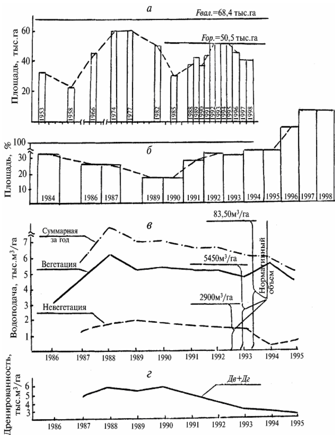
Рис. 6.4.1.3. Динамика показателей мелиоративной обстановки на Шурузьяском массиве
