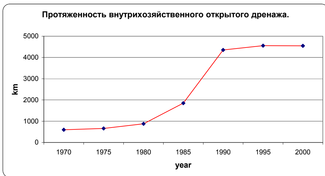
Рис.6.6.1.4.4 Протяженность внутрихозяйственного открытого дренажа
