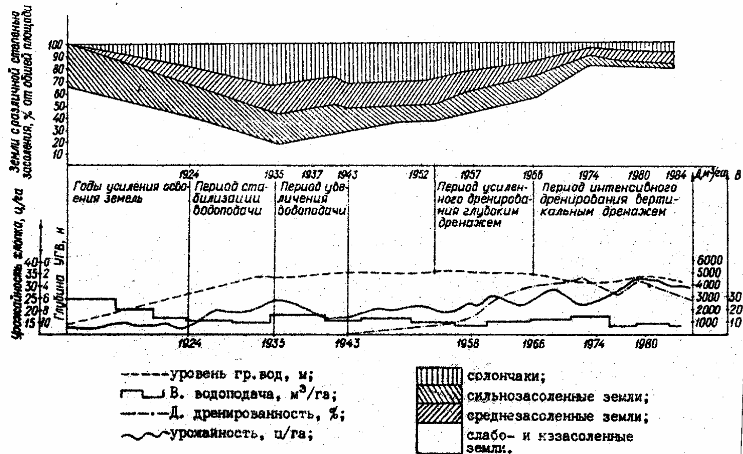
Рис.8.2. Измерение показателей мелиоративного состояния земель в зоне старого орошения Голодной степи под влиянием водохозяйственных мероприятий (площадь 102000 га)
