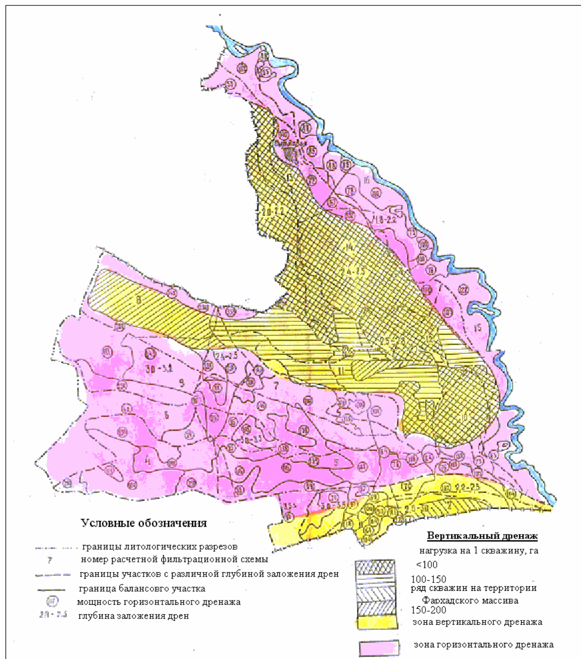
Рис. 6.4.1.2 Зоны обслуживания вертикального и горизонтального дренажа
