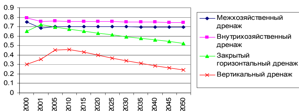
Объем ремонтно - очистительных работ. Сценарий 3.
