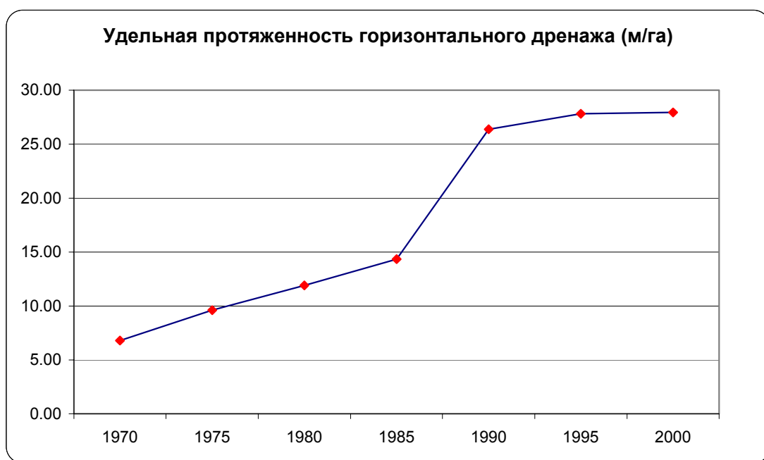
Рис.6.6.1.4.2 Удельная протяженность горизонтального дренажа Кашкадарьинской области
