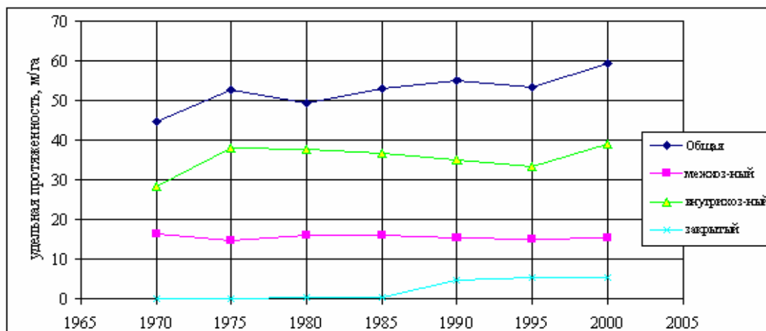
Рис. 6.3.1.3 Удельная протяженность горизонтального дренажа
