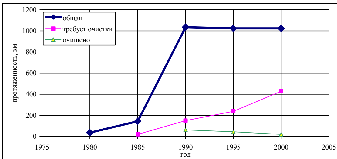
Рис. 6.2.1.7 Состояние закрытого горизонтального дренажа
