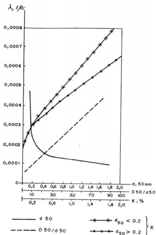
Рис.5.3. Зависимость интенсивности отказов электронасосов от литологии и состава гравийной обсыпки и пескования в момент пуска ( K )
