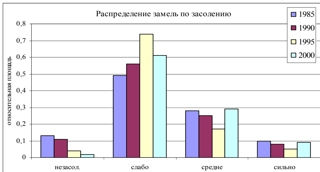
Рис. 6.4.1.7 Диаграммы засоления почв
