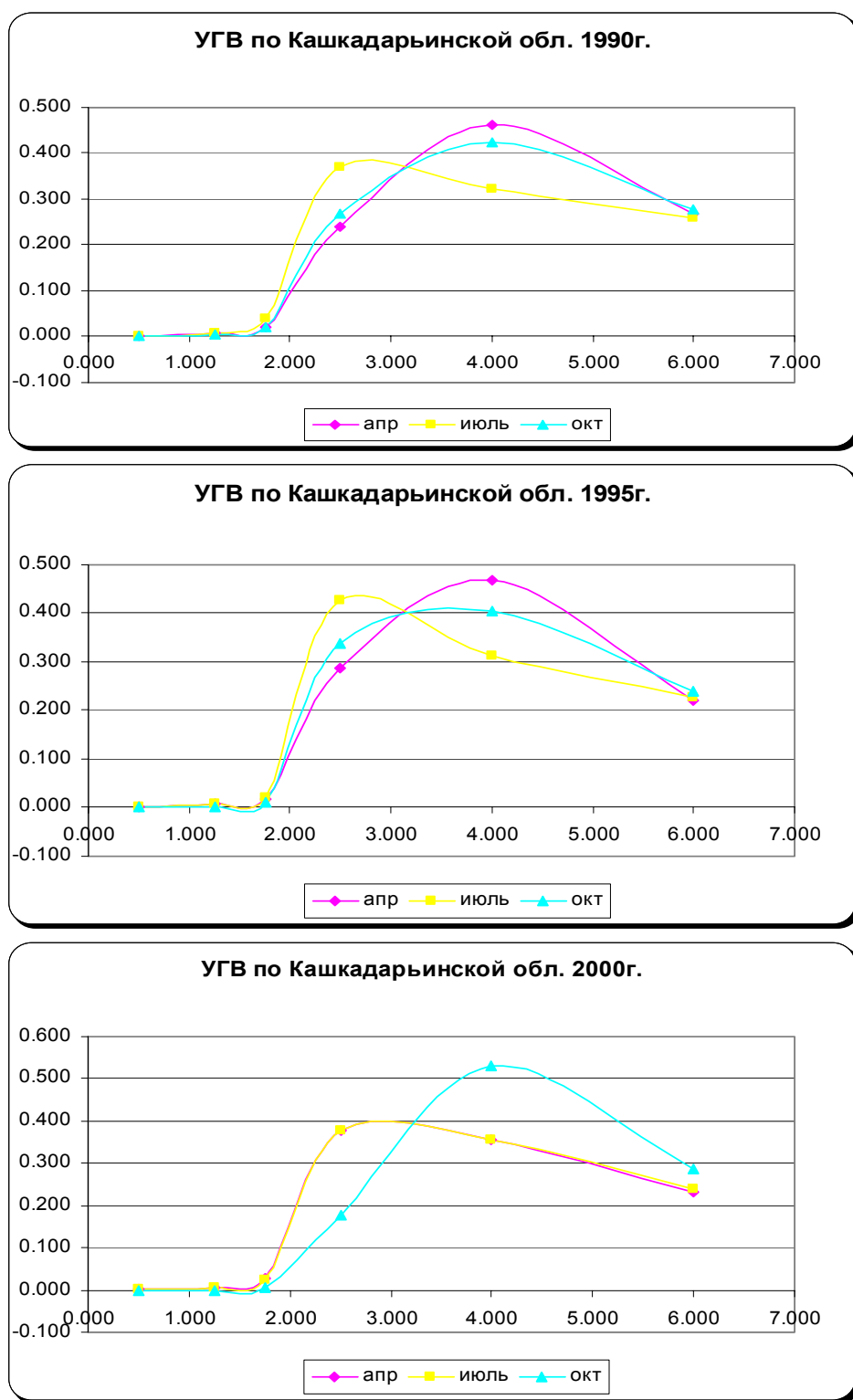
Рис. 6.6.1.5.2.1 Графики глубины залегания грунтовых вод Кашкадарьинской области (в относительных единицах).
