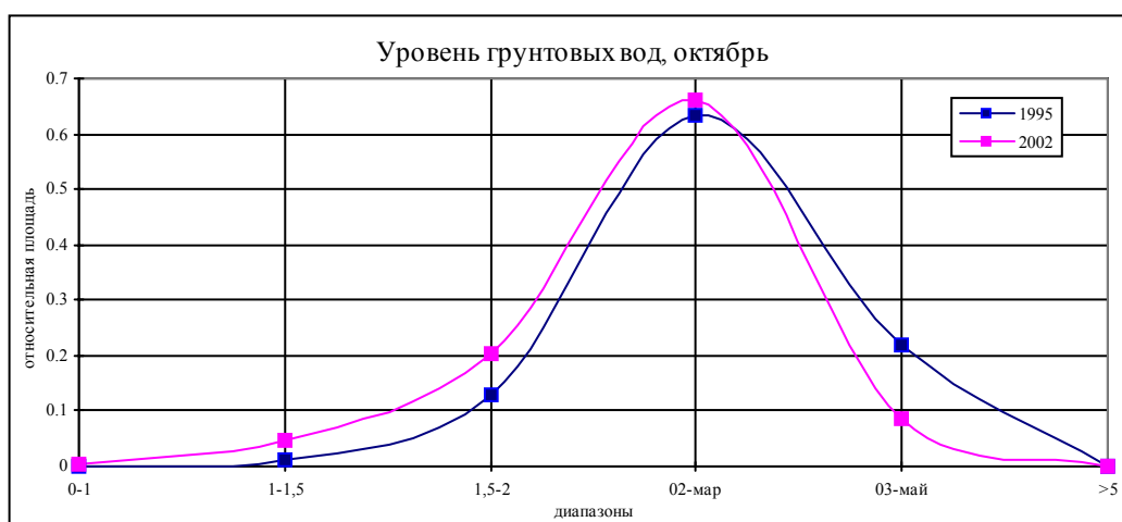
Рис. 6.1.1. Функция распределения по уровню залегания грунтовых вод
