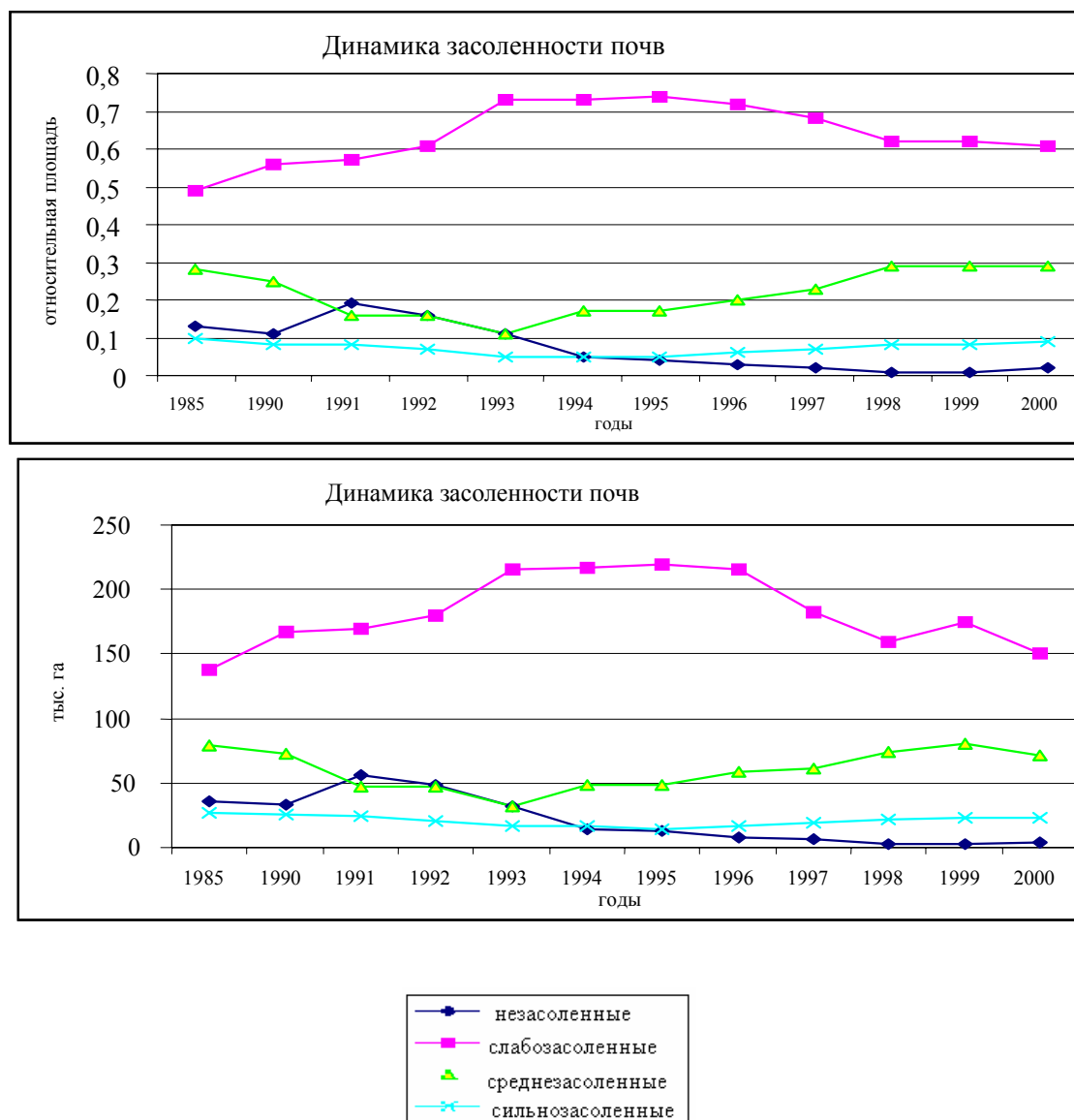
Рис 6.4.1.8 Динамика засоления почв
