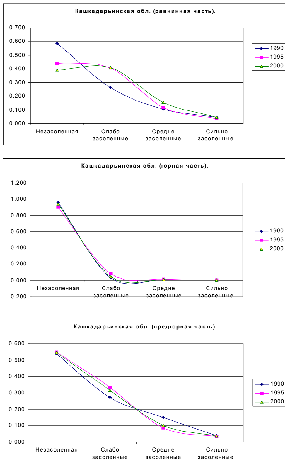
Рис. 6.6.1.5.3.1 Распределение орошаемых площадей по степени засоления (все диаграммы выполнены в относительных единицах)
