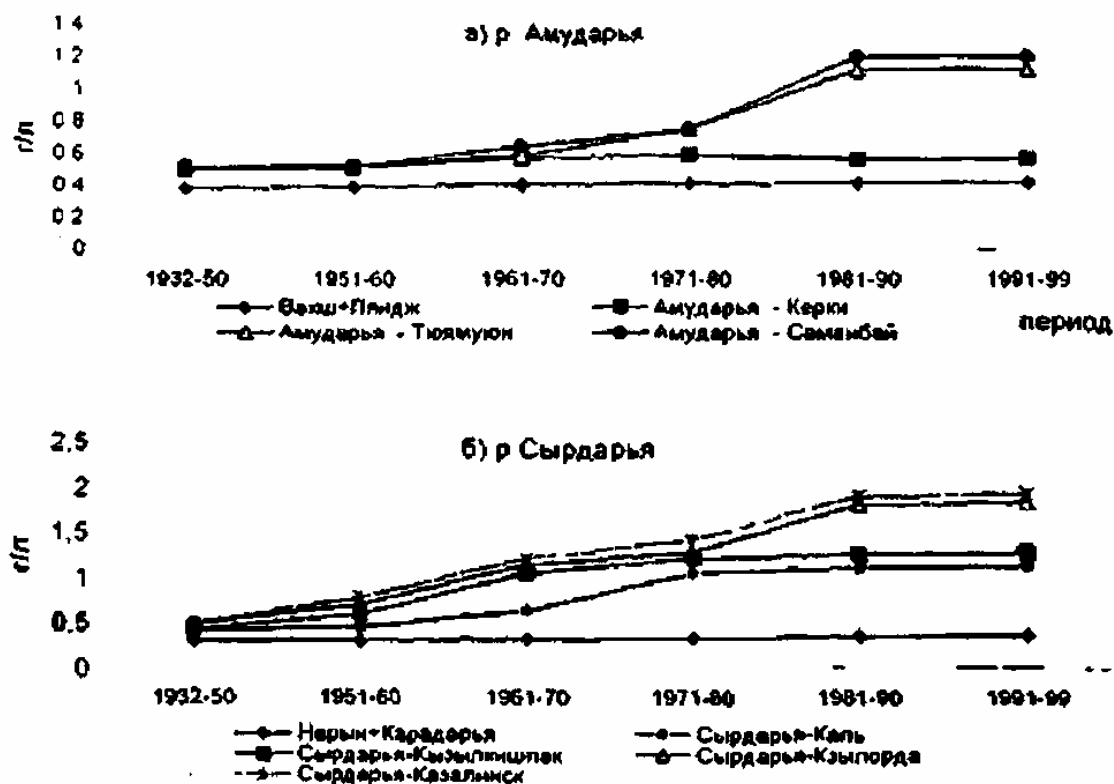
Рис. 7.1 Многолетний тренд минерализации речного стока по створам рек
