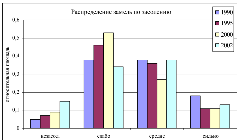
Рис. 6.5.1.10 Диаграммы засоления почв
