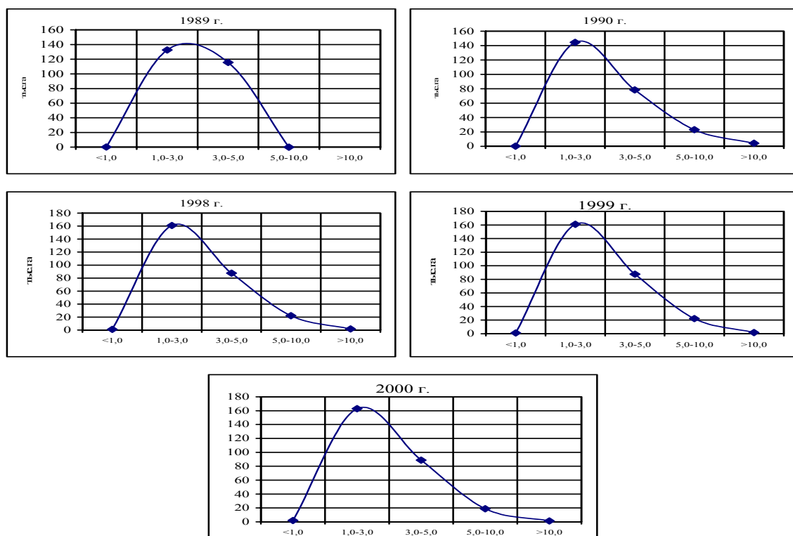
Рис. 6.2.1.16. Диаграммы распределения площадей орошения по минерализации грунтовых вод
