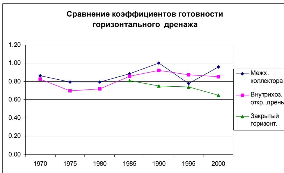
Рис. 6.6.1.4.5 Сравнение коэффициентов готовности
