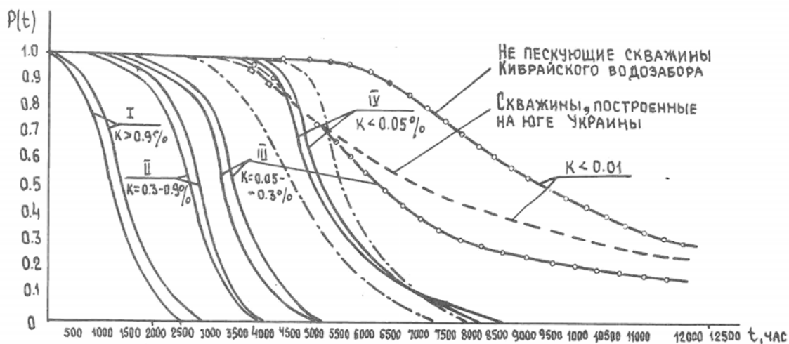
Рис.5.4. Вероятность безотказной работы электронасосов в водоносных грунтах при разной степени пескования скважин вертикального дренажа
