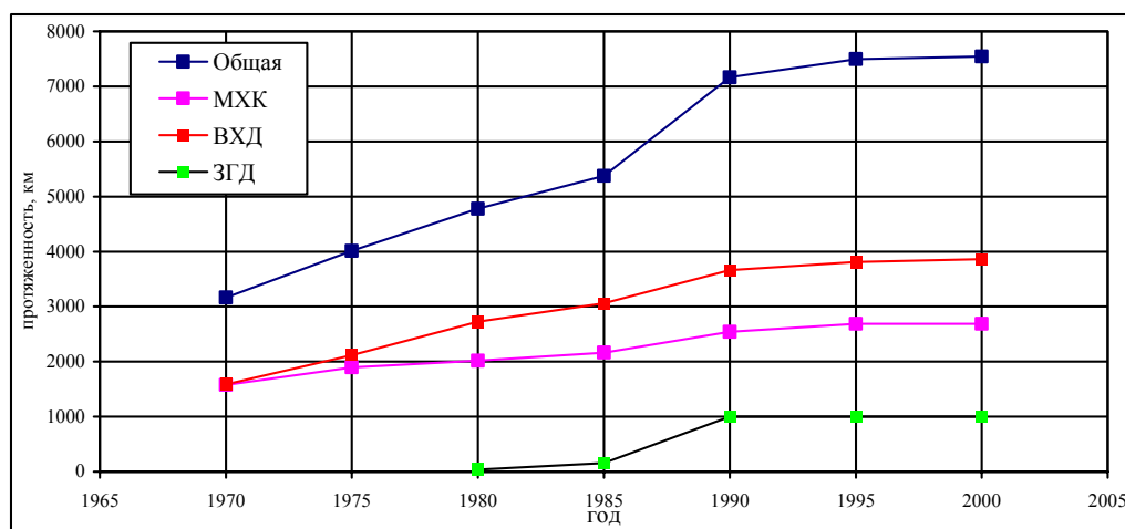
Рис. 6.2.1.4 Протяженность горизонтального дренажа Бухарской области
