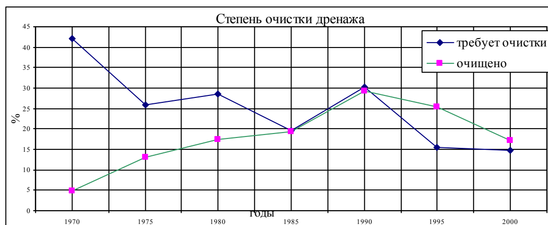
Рис. 6.5.1.6 Состояние межхозяйственного дренажа
