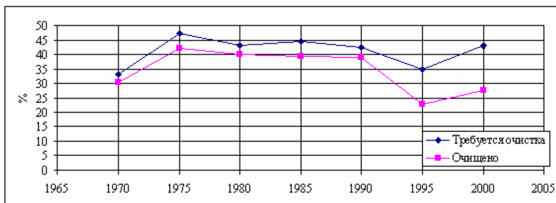
Рис. 6.3.1.4 Состояние межхозяйственных коллекторов
