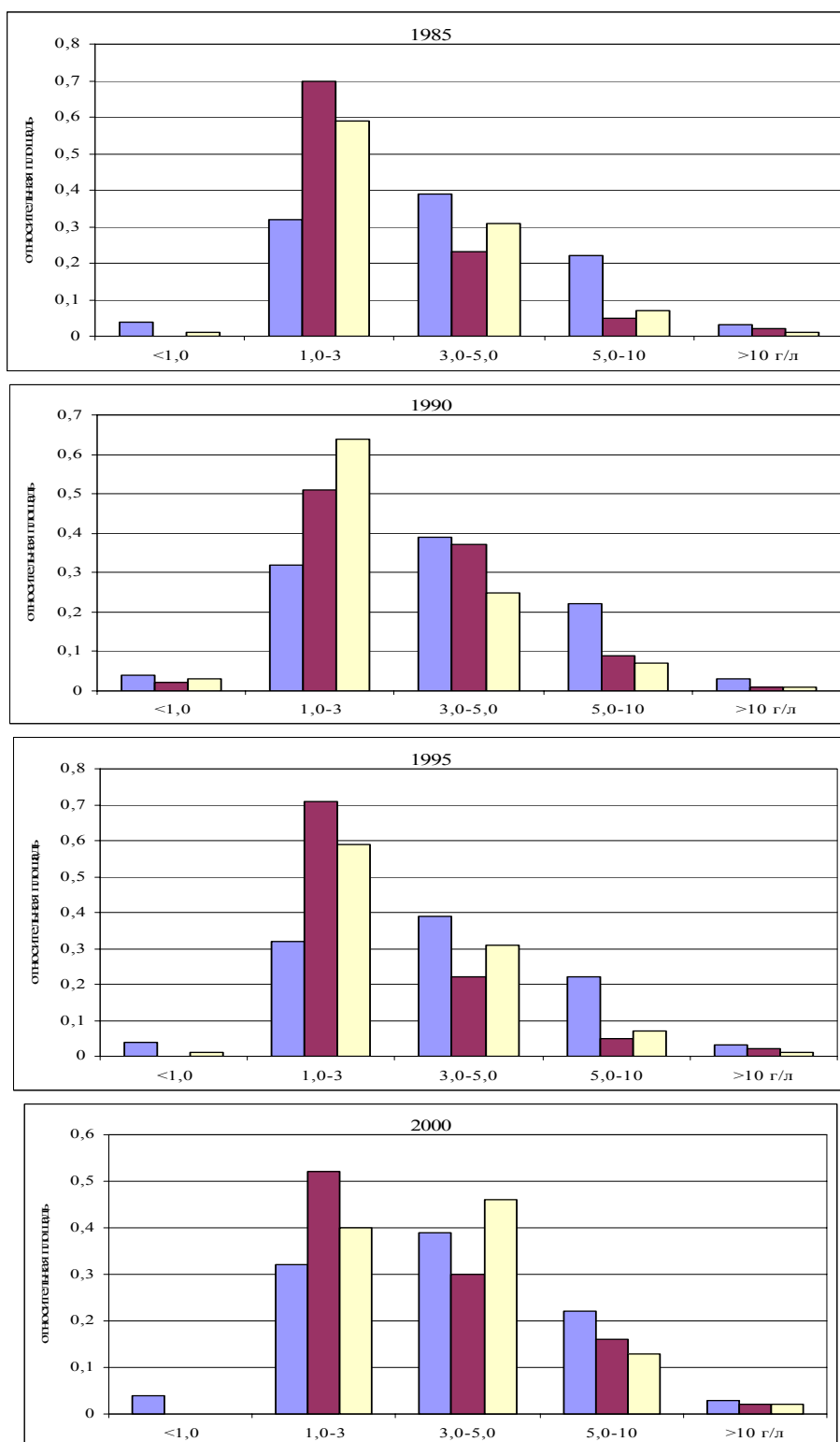
Рис. 6.5.1.9 Распределение площадей по минерализации грунтовых вод
