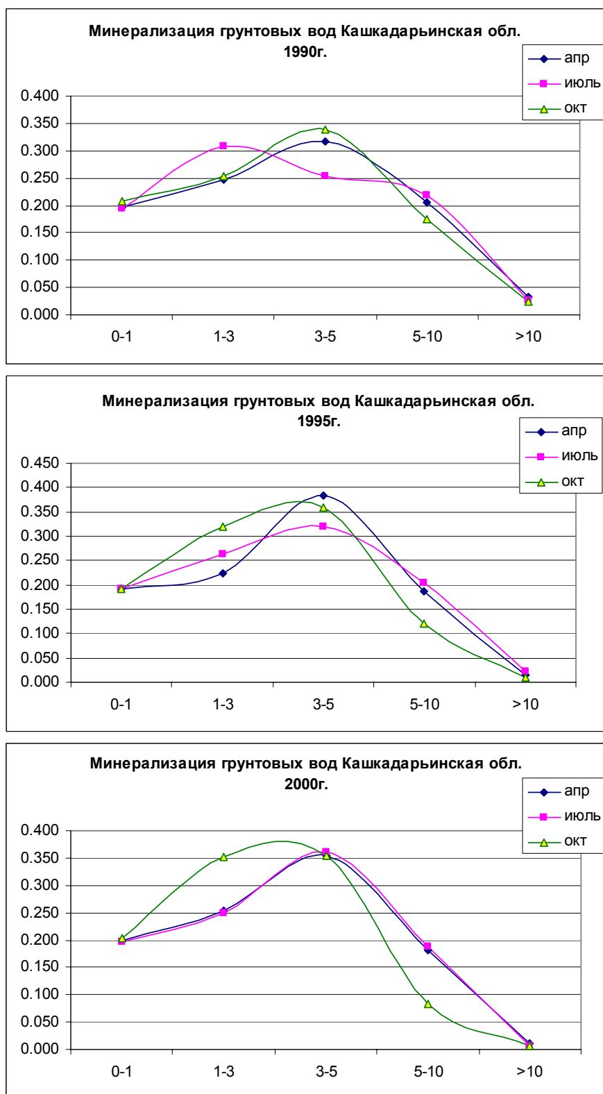
Рис. 6.6.1.5.2.2 Диаграммы минерализации грунтовых вод Кашкадарьинской области (в относительных единицах)
