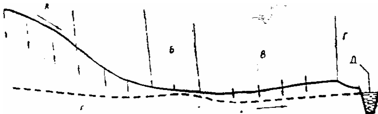
Рис 2.1. Схема гидрогеологических зон орошения территорий Центральной Азии
