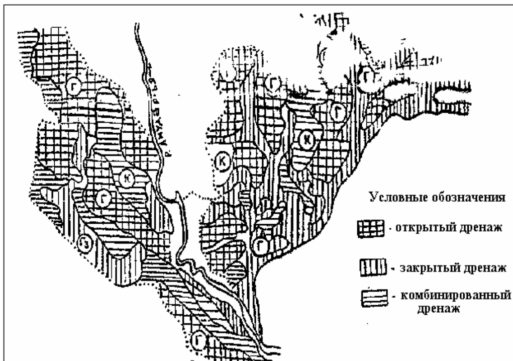
Рис. 6.5.1.7 Схема районирования северной зоны Республики Каракалпакстан
