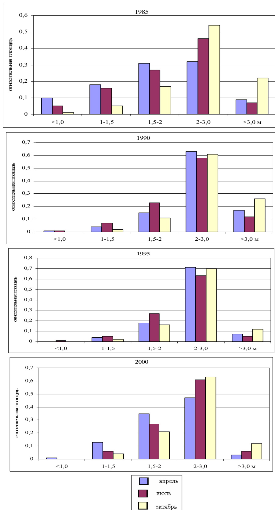
Рис. 6.4.1.5 Диаграммы уровня залегания грунтовых вод Сырдарьинской области
