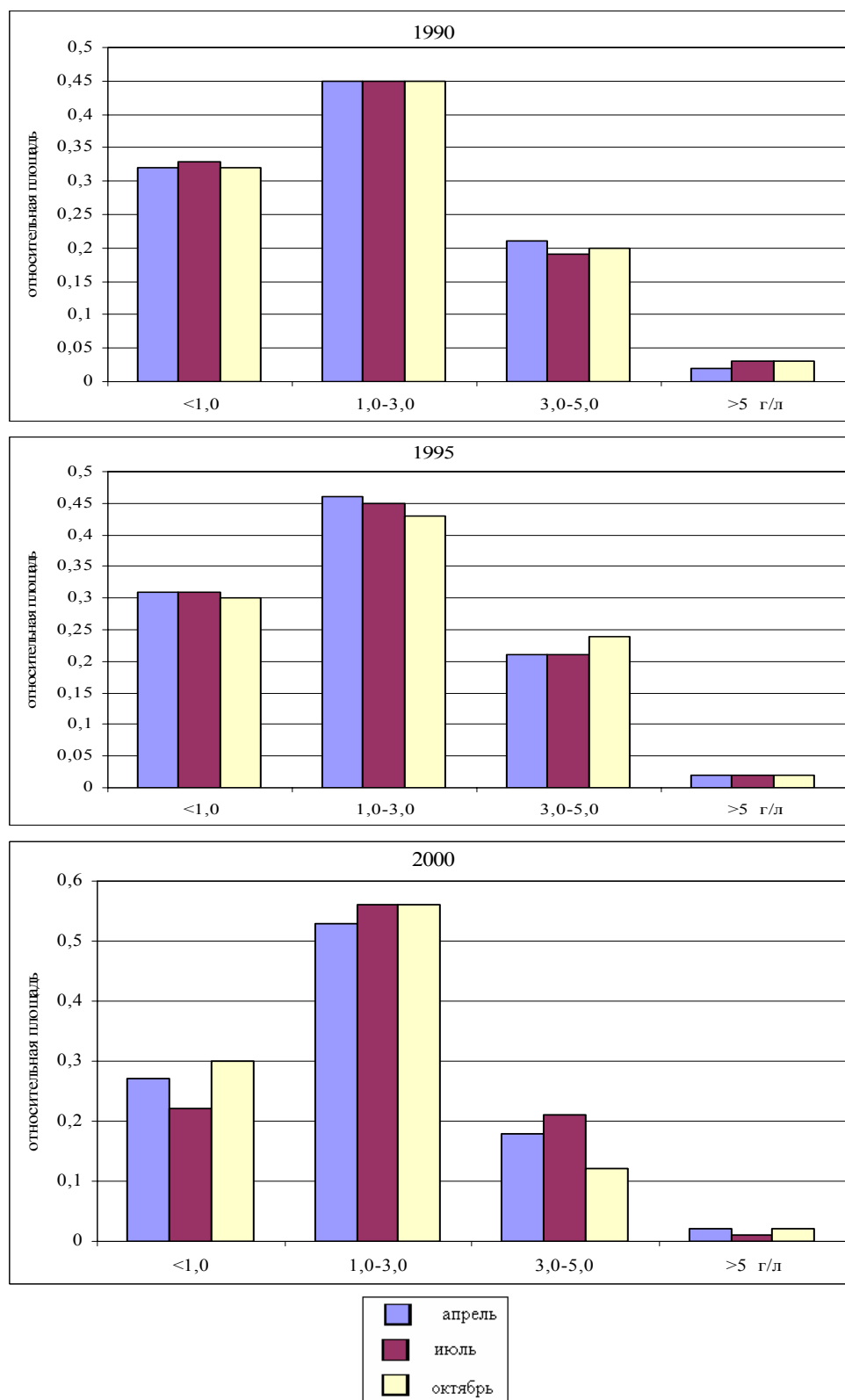
Рис. 6.3.1.11 Распределение орошаемых площадей по минерализации грунтовых вод
