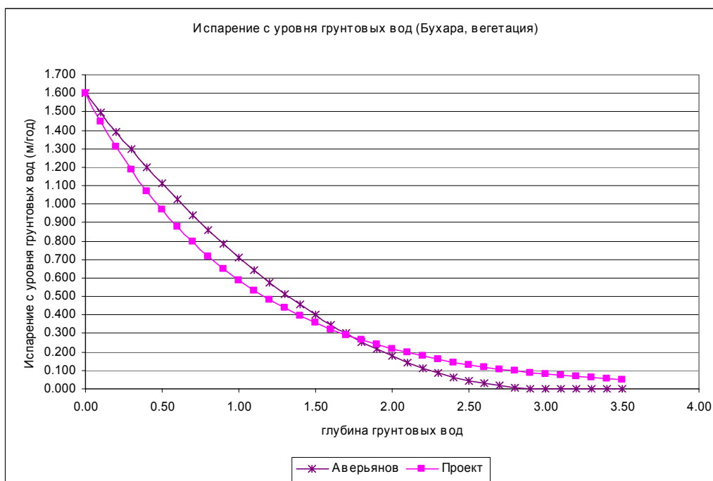
Рис 6.1.3. Испарение с уровня грунтовых вод
