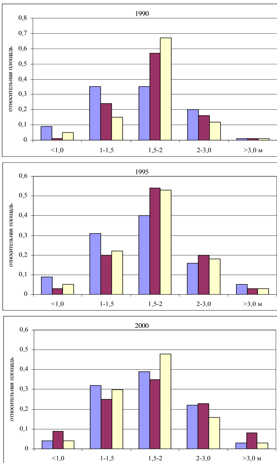
Рис. 6.5.1.8 Распределение площадей по глубине залегания грунтовых вод
