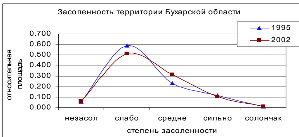
Рис. 6.1.2 Функция распределения по степени засоленности почвы
