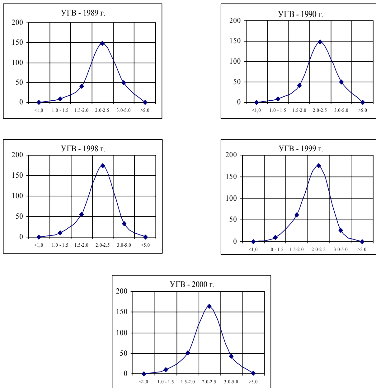
Рис. 6.2.1.15. Диаграммы распределения УГВ по площади орошения
