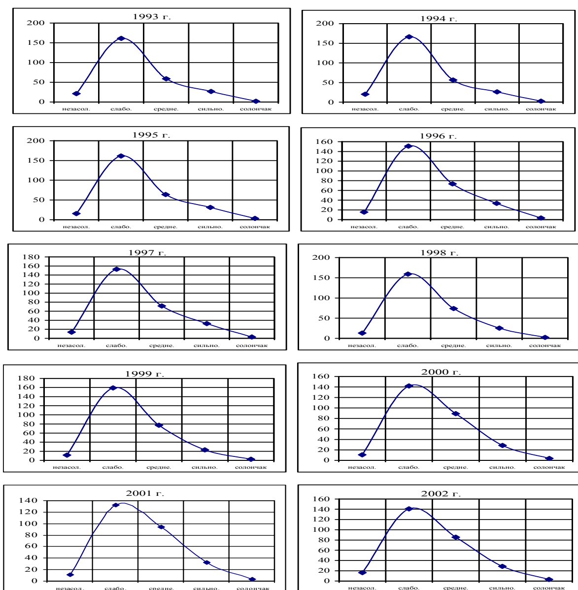
Рис. 6.2.1.18. Диаграммы распределения орошаемых земель по засолению
