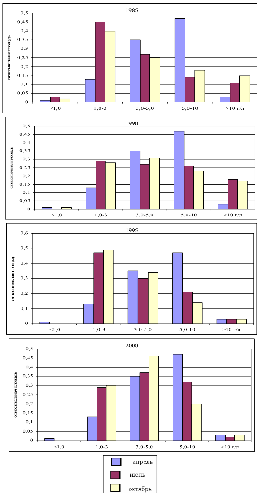
Рис. 6.4.1.6 Диаграммы минерализации грунтовых вод Сырдарьинской области
