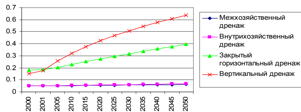
Доля дренажной сети требующей, полной реконструкции. Сценарий 3.
