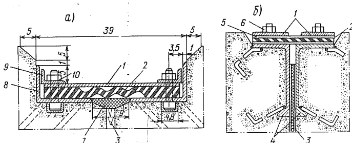
Рис. 3-18. Схемы наружных контурных уплотнений узких осадочных швов (размеры в см) с резиновой профилированной лентой: а - на камерах шлюзов Воткинской ГЭС, Волжской ГЭС имени ХХП съезда КПСС; б - на плотине Имперлэз (США)
