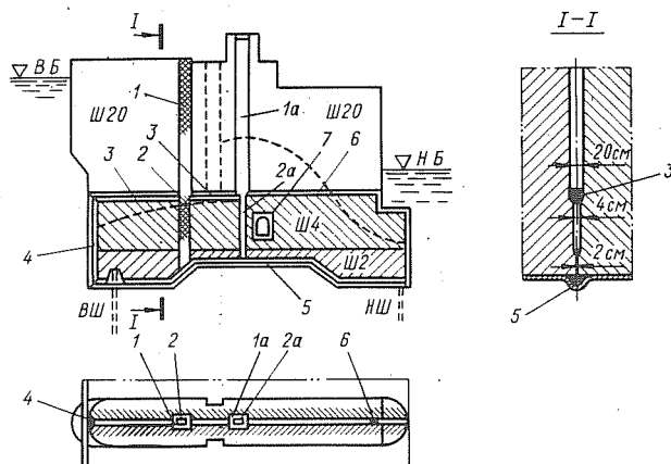
Рис. 2-5. Размещение уплотнений в деформационных швах и швах-надрезах массивного гидросооружения на сжимаемом основании (размеры в см)
