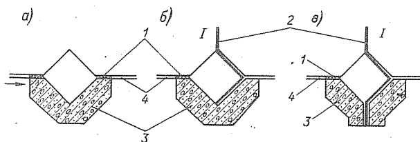
Рис. 3-13. Нерекомендуемые схемы ограждений асфальтовых шпонок в температурных швах: а - ограждение шпонок конопаткой, просмоленной паклей; б - ограждение шпонок, установленной внутри металлической диафрагмы, и одним концом заделанной в бетон I; в - ограждение шпонок металлической диафрагмой, одним концом заделанной в бетон I, вторым концом выпущенной между корытами
