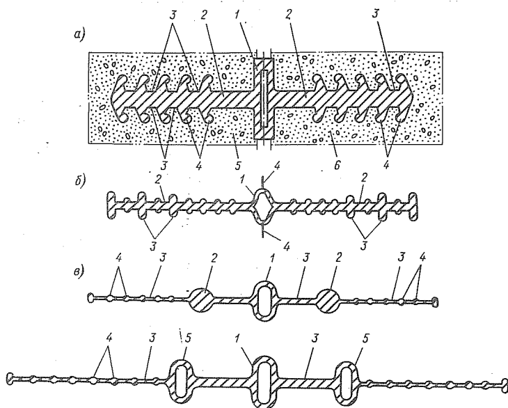
Рис. 3-2. Конструкции уплотнений из эластического синтетического материала (Швеция)
