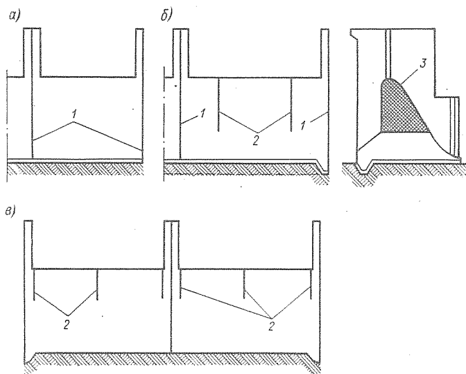
Рис. 2-1. Схема разрезки сооружения на сжимаемом основании деформационными швами: а – только сквозными швами; б – смешанной системой сквозных и несквозных швов; в – только одним несквозными швами
