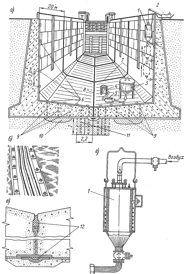
Рис. 6-32. Схема ремонта уплотнений осадочных швов камер шлюзов № 7 и 13 Волго-Донского канала имени В. И. Ленина: а - общая схема камеры шлюза; б - уплотнение продольного шва; в - шпонка продольного шва днища; г - битумный иньектор
