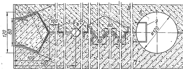
1 – железобетонный брус; 2 – окраска битумом; 3 – оклейка битумматами; 4 – металлический лист между битумматами; 5 – медный лист с компенсатором; 6 – дренаж; 7 – стальные листы с компенсаторами; 8 – смотровая шахта; 9 – лестница
