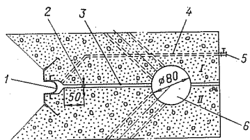
Рис. 6-1. Схема уплотнения температурного шва плотины Мерайе (Франция) (размеры в см)
