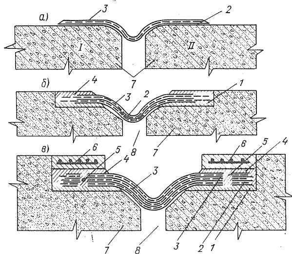
Рис. 5-16. Безанкерные поверхностные уплотнения клеечного типа: а – однослойное; б – двухслойное с пластрастровной подготовкой площадок сцепления; в – трехслойное усиленное с перфорацией
