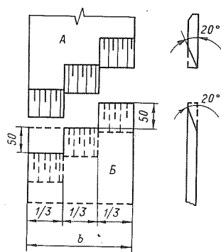
Рис. 5-10. Схема сращивания резиновых лент
