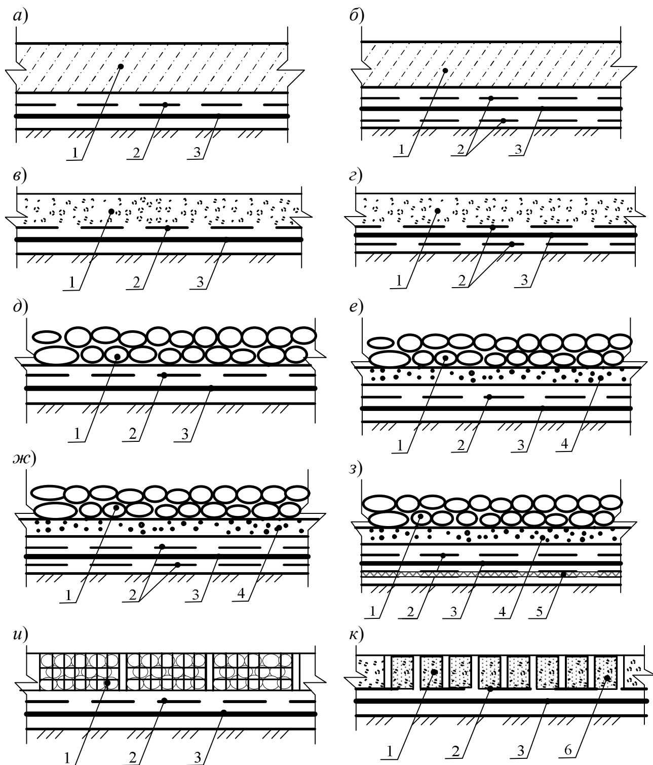
а, б – с геомембраной и защитным покрытием из бетона; в, з – с геомембраной и защитным покрытием из грунта; д, з – с геомембраной и защитным покрытием из каменной наброски; и, к – с геомембраной и защитным покрытием из габионов и георешетки; 1 – защитное покрытие; 2 – защитная прокладка из геотекстиля; 3 – противофильтрационный элемент из геомембраны; 4 – защитный слой из песка; 5 – дренажный элемент из геокомпозита; 6 – георешетка; 7 – габионы
