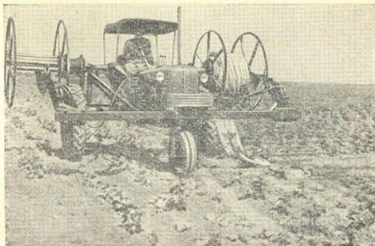
Рис. 46. Прямая сборка гибкого трубопровода после полива при движении трактора задним ходом.
