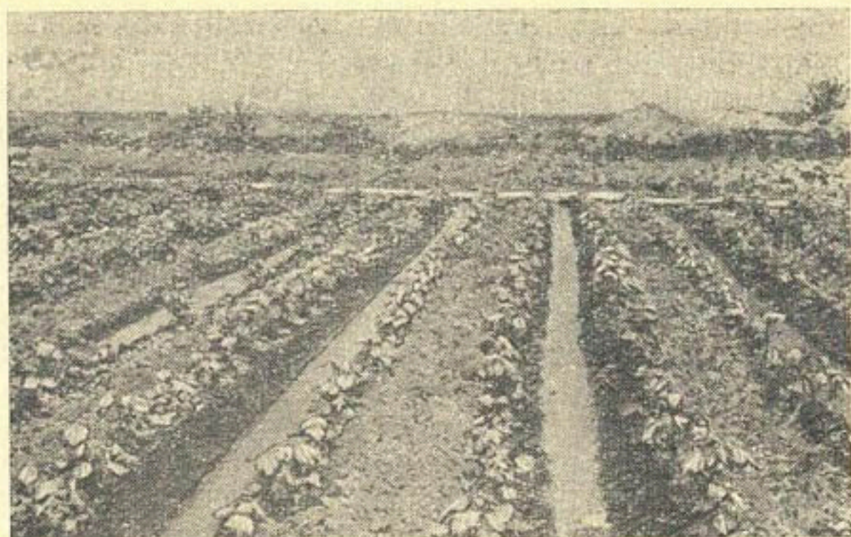
Рис. 35. Полив хлопчатника через борозду с помощью гибкого трубопровода.
