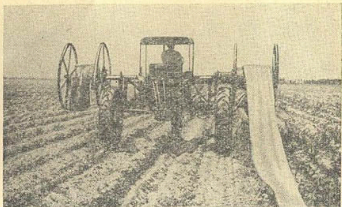
Рис. 4. Укладка и сборка гибких трубопроводов с помощью навесного намоточного устройства с двумя катушками.
