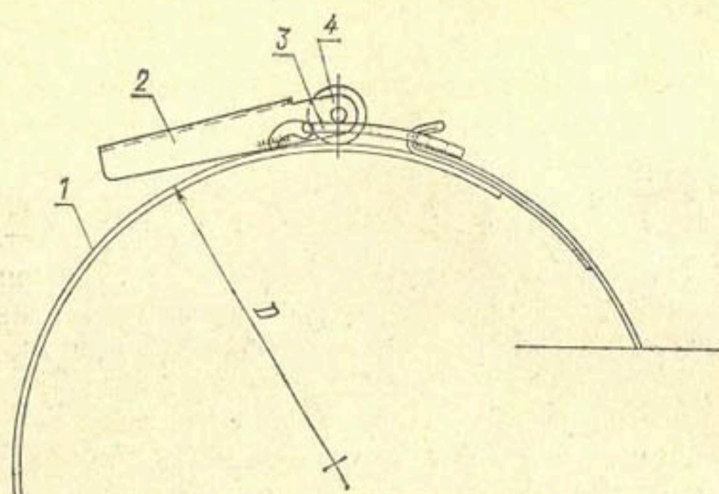
Рис. 31. Хомут с эксцентриковым замком: 1 — ленты хомута; 2 — рукоятка; 3 — планка; 4 — осевой ролик.
