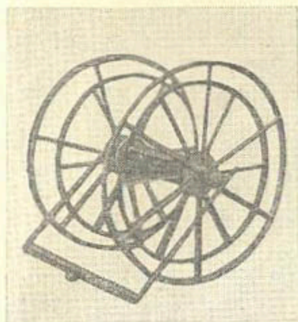
Рис. 48. Двойная катушка для полумеханизированной укладки, сборки и перемещения гибких трубопроводов со съемной тягой для буксировки.
