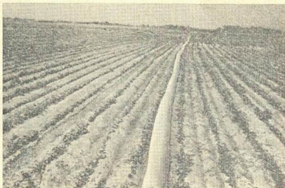
Рис. 3. Гибкий транспортирующий трубопровод, уложенный в междурядье хлопчатника.
