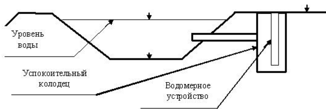
Рисунок 7 – Размещение уровнемерного устройства в успокоительном колодце
