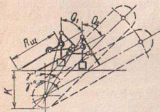
Рис. 47. Корректирование коленчатым шупом.
