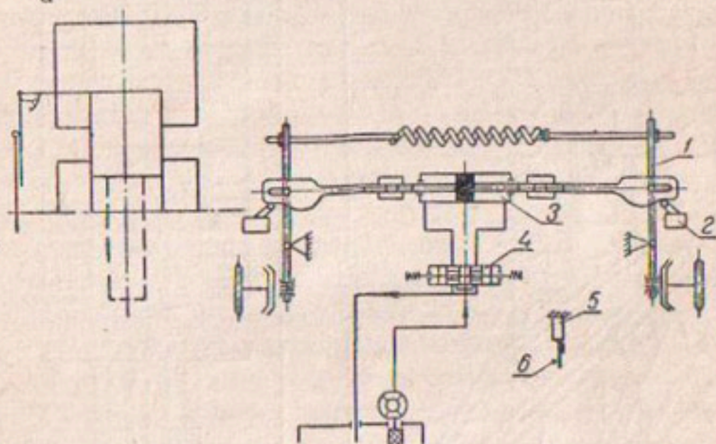
Рис. 53. Схема автоматического вождения по копиру (ВНИИЗемМаш):
