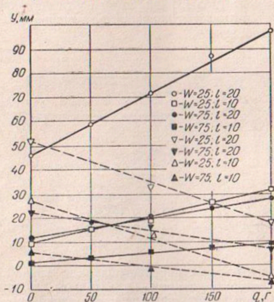
Рис. 41. Зависимость провисания копирного тросика 2 мм от натяжения ( W ), расстояния между опорами ( l ), величины и направления давления щупа на тросик ( q ) сверху (сплошная линия) или снизу (пунктирная линия).
