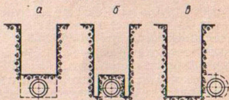
Рис. 83. Способы рытья траншей для перекладки дрен:
