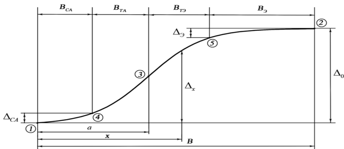
Рисунок 1 - Геоморфологическая схематизация ландшафтной катены: B – ширина ландшафтной катены; B_{ca} , B_{та} , B_{тэ} , B_э – протяженности соответственно супераквального, трансаккумулятивного, трансэлювиального и элювиального элементарных ландшафтов; \Delta_{ca} и \Delta_э – перепады высот соответственно супераквального и элювиального элементарных ландшафтов; 1, 2, 3, 4, 5 – характерные точки [2]
