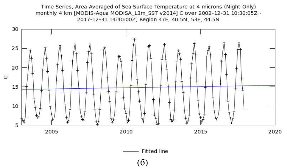
Р и с. 1 (а, б). Сезонная и межгодовая изменчивость ТПМ (среднемесячные значения), средней для Северного (а), Среднего (б) и Южного (в) Каспия и КБГ (г) (2003–2017 гг.). Прямые линии на рисунках – линейные тренды ТПМ в рассматриваемый период.
