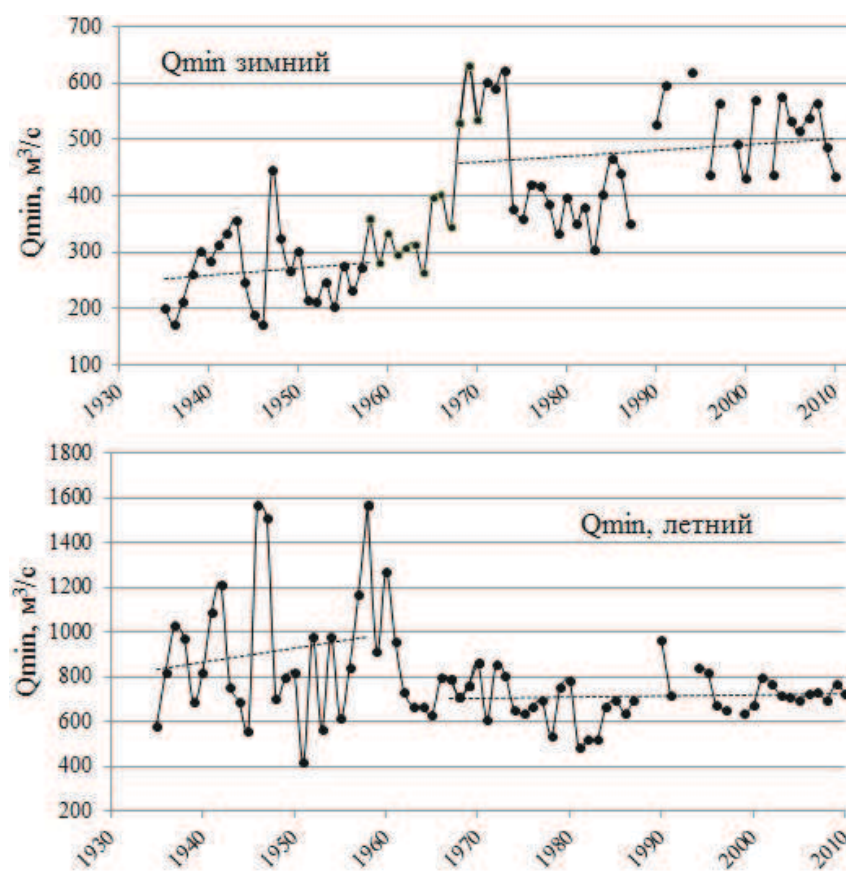
Рис. 2. Межгодовая динамика минимального среднемесячного стока р. Иртыш – п. Семиярка. Тенденции минимального стока, обозначенные пунктирной линией, статистически незначимы
