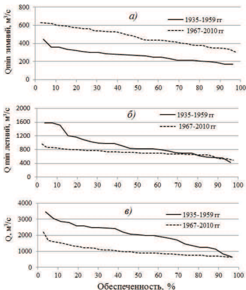
Рис. 3. Эмпирические кривые обеспеченности стока в естественных и зарегулированных условиях (р. Иртыш – п. Семиярка)
