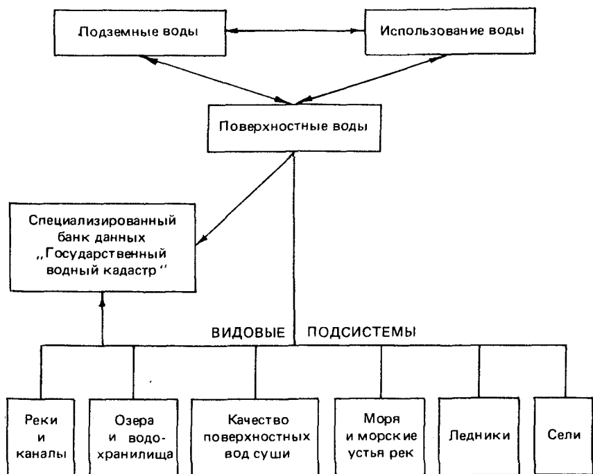
Рис. 2. Организационная структура АИС ГВК.
