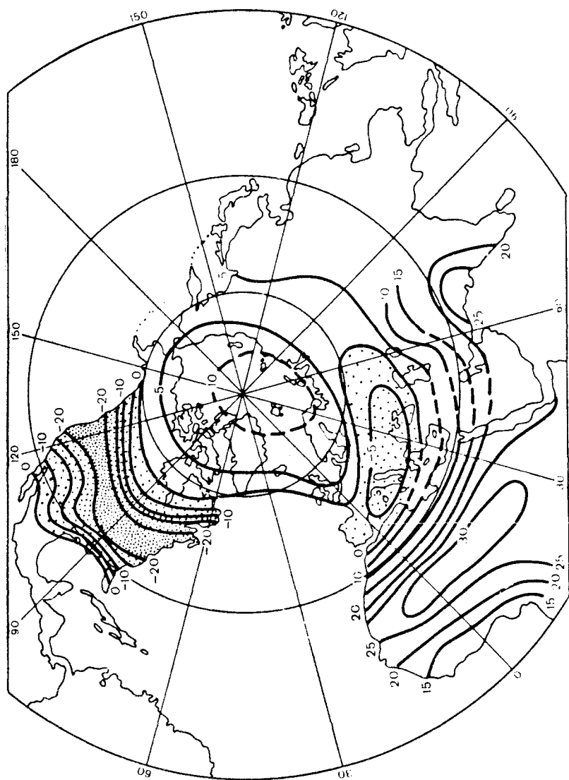
Рис. 29. Изменение годовой суммы осадков (в см слоя) в северном полушарии при повышении глобальной температуры воздуха на 1^{\circ}\text{C} (на 2000 г.).
