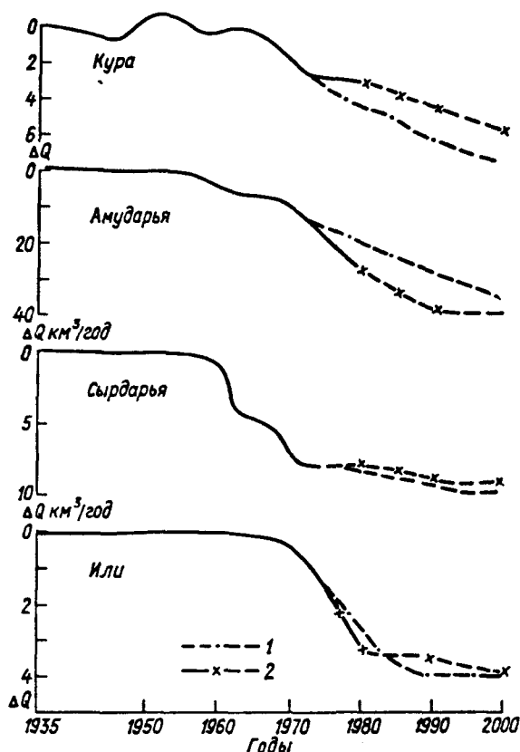
Рис. 6. Изменения годового стока рек СССР под влиянием хозяйственной деятельности для средних климатических условий (стационарная климатическая даны). 1 — расчеты и прогнозы изменений, выполненные в 1975 г., 2 — то же в 1985 г.
