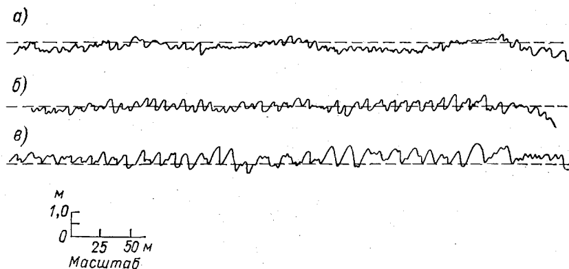
Рис. 86. Развитие гряд в дноуглубительной прорези на р. Дон (по Снищенко).
