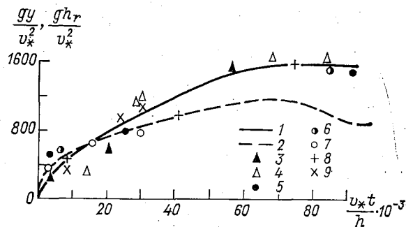
Рис. 87. График роста гряд в дноуглубительных прорезях (по Снищенко).
