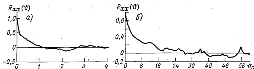
Рис. 23. Временные (одноточечные) корреляционные функции R_{xx}(\tau) . а — по измерениям Райхлена в лабораторном лотке, б — по измерениям Гринвальда на р. Турунчук.
