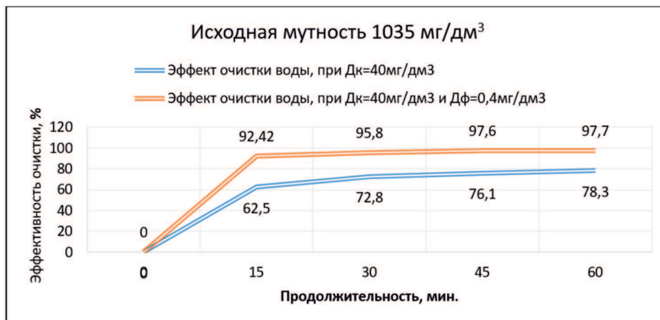
Рис. 4 – Сравнение эффекта осветления воды при применении традиционного коагулянта в сочетании с современным флокулянт
