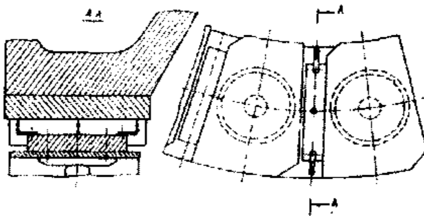
Рис. Д.1 Расположение датчиков биения зеркальной поверхности диска подпятника
