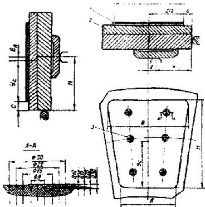
Рис. Д.5 Эластичный металлопластмассовый сегмент:
