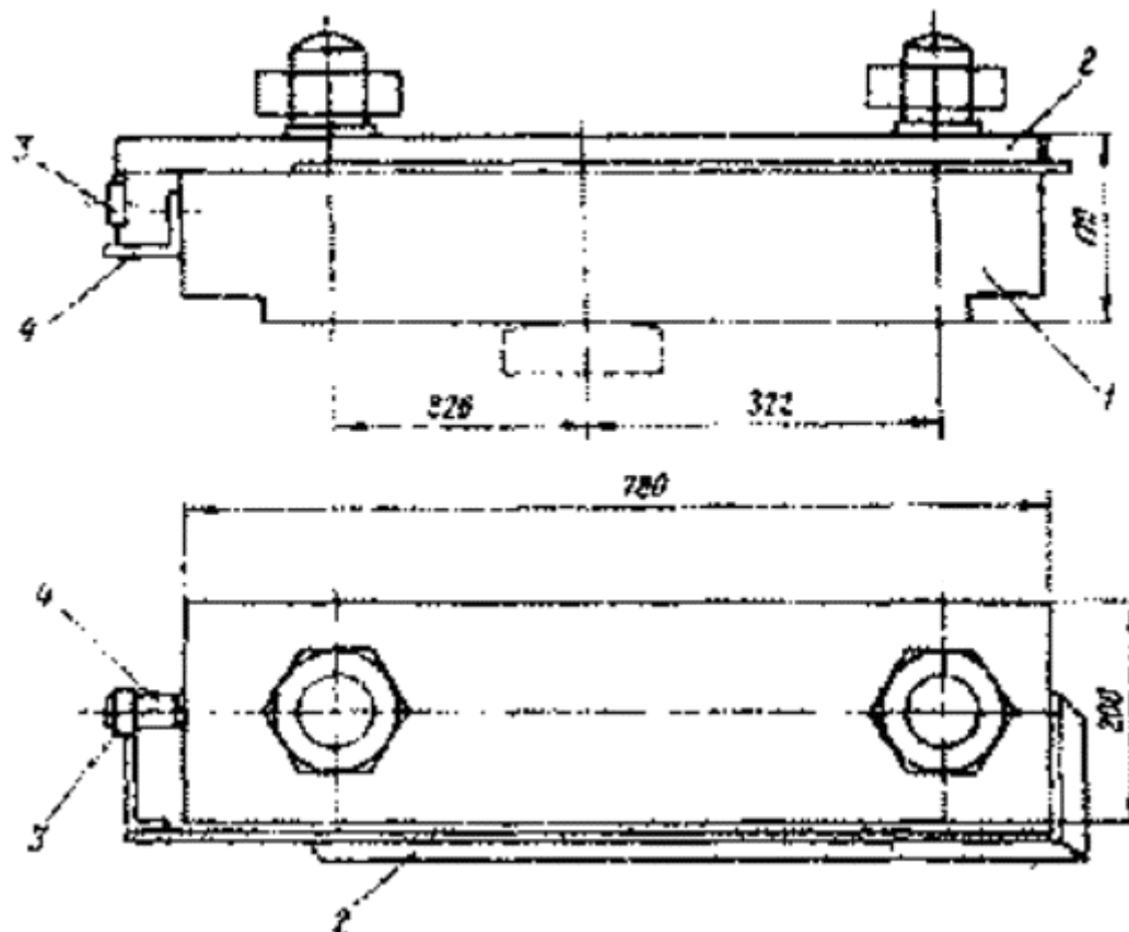
Рис. Д.3. Рычажно-индикаторное устройство для определения нагрузки на пару сегментов по прогибу балансира:
