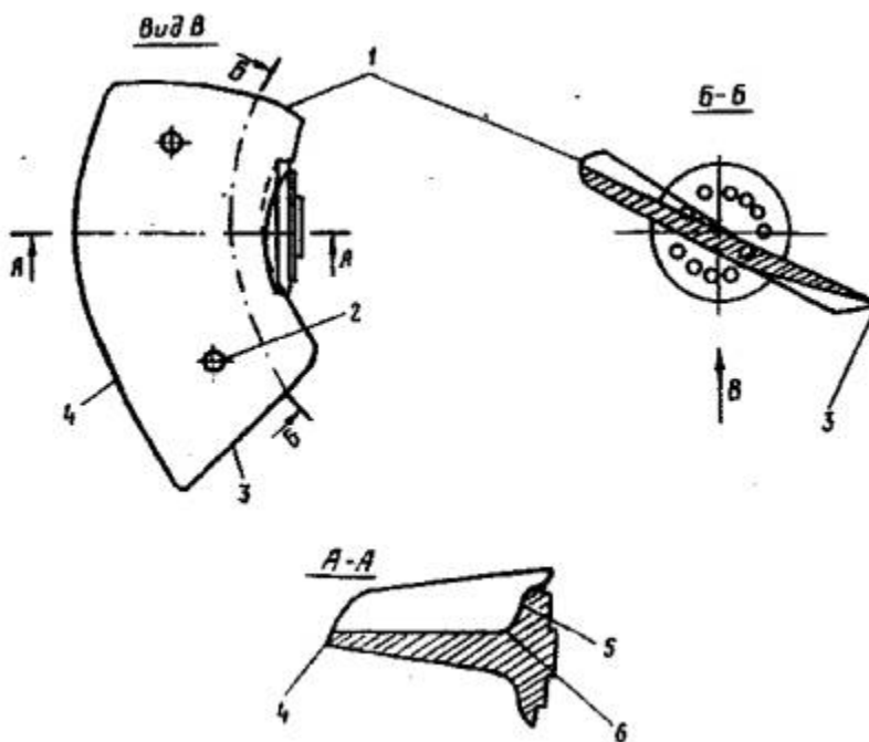
Рис. 2. Схема лопасти рабочего колеса поворотного-лопастной гидротурбины с указанием основных мест контроля.
