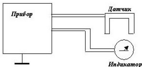
Рис. 1 Блок-схема соединений к прибору датчика-индуктора и микроамперметра-индикатора.
