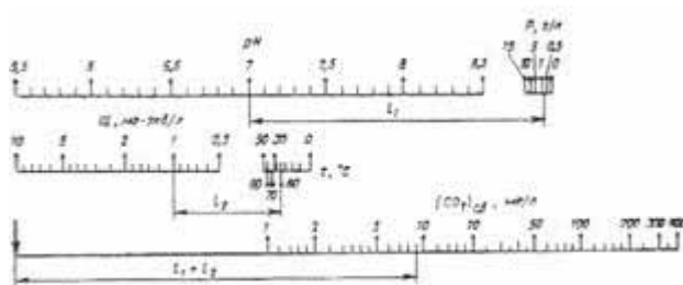
Рис. 2. Номограмма для определения концентрации свободной двуокиси углерода в природной воде (или pH)
