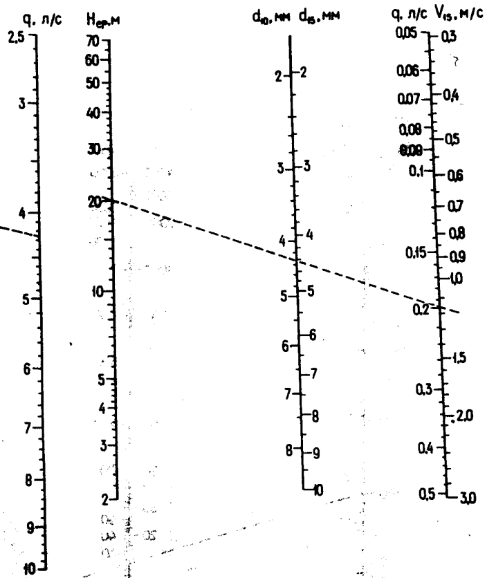
Черт. 6. Номограмма для определения диаметров отверстий диафрагм, устанавливаемых у смесителей водоразборной арматуры санитарных приборов
