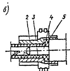
Рис. 17. Схема формирования утолщенного бурта на конце трубы
