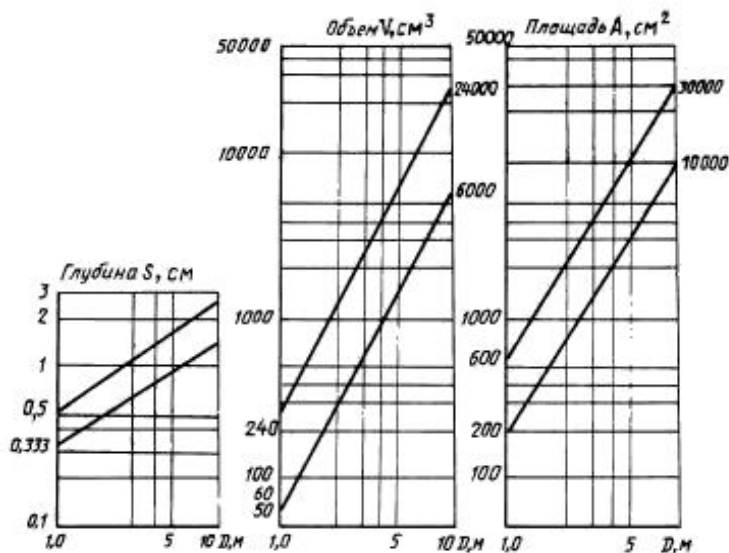
Черт. 4. Примеры количественных характеристик кавитационной эрозии
