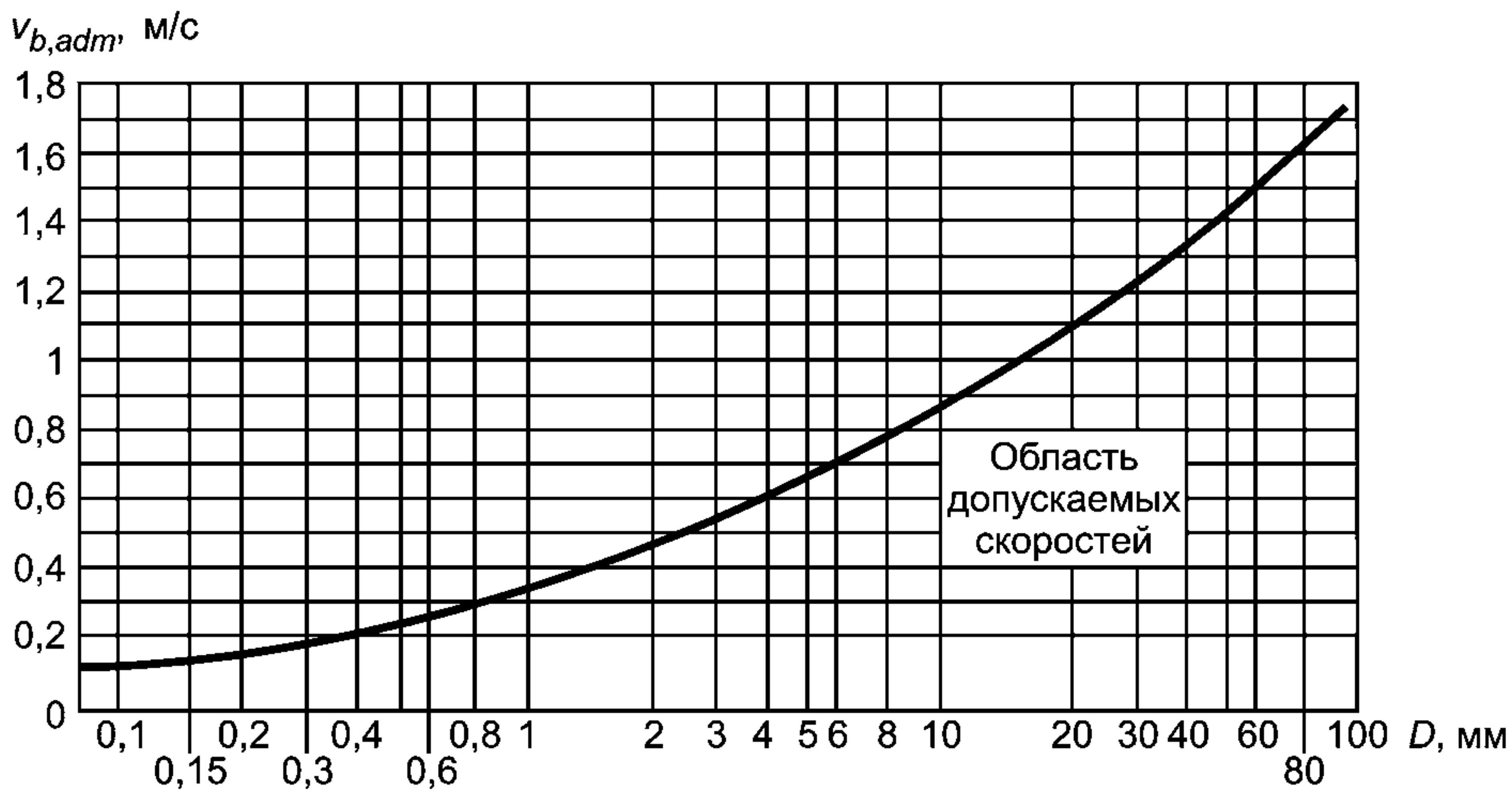
Рисунок 7 — График допускаемых значений неразрывающих донных скоростей
