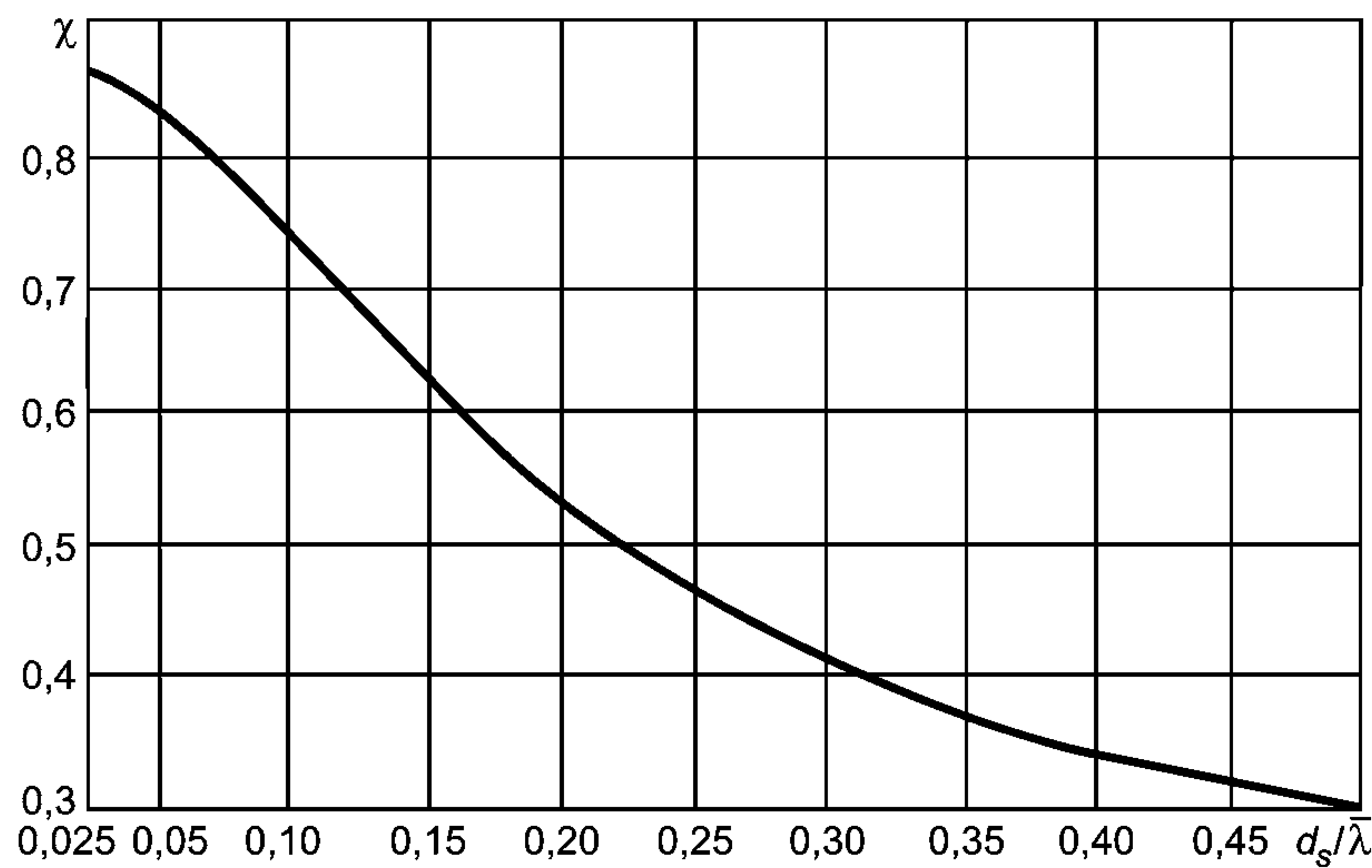
Рисунок 32 — График значений коэффициента \chi
