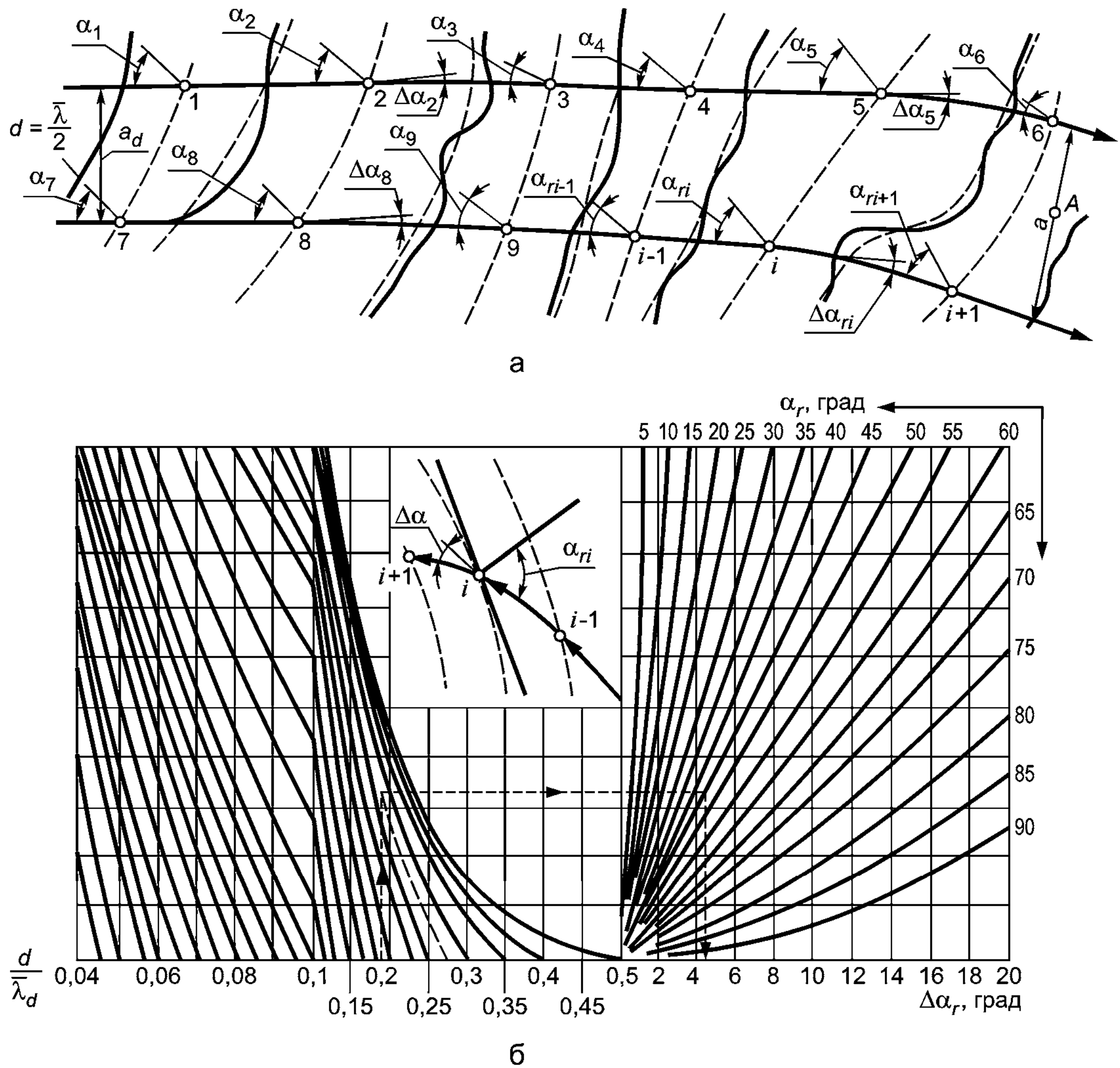
Рисунок А.6 — Схема (а) и графики (б) для построения плана рефракции
