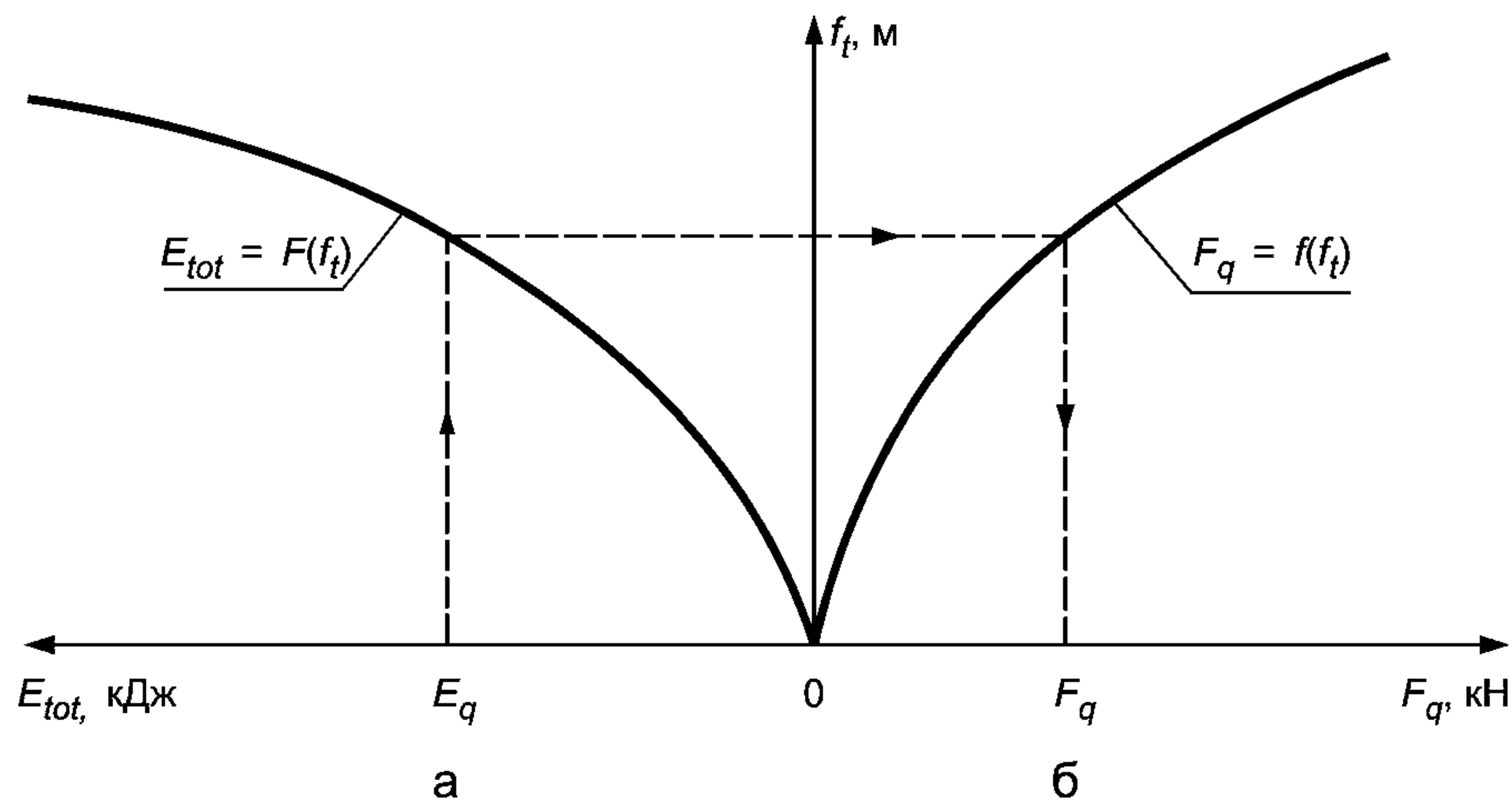
Рисунок 33 — Схема построения графиков зависимости деформаций отбойного устройства (и причального сооружения) f_t
