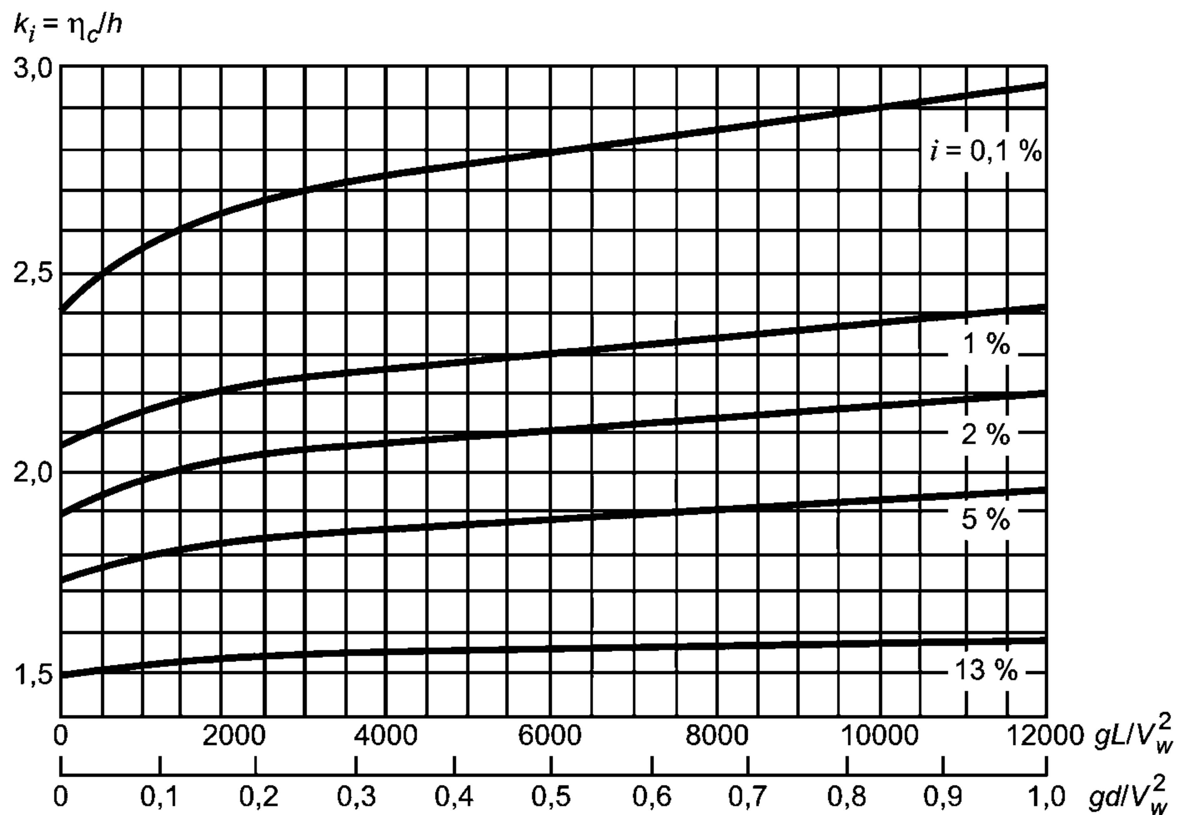
Рисунок А.2 — Графики значений коэффициента k_i
