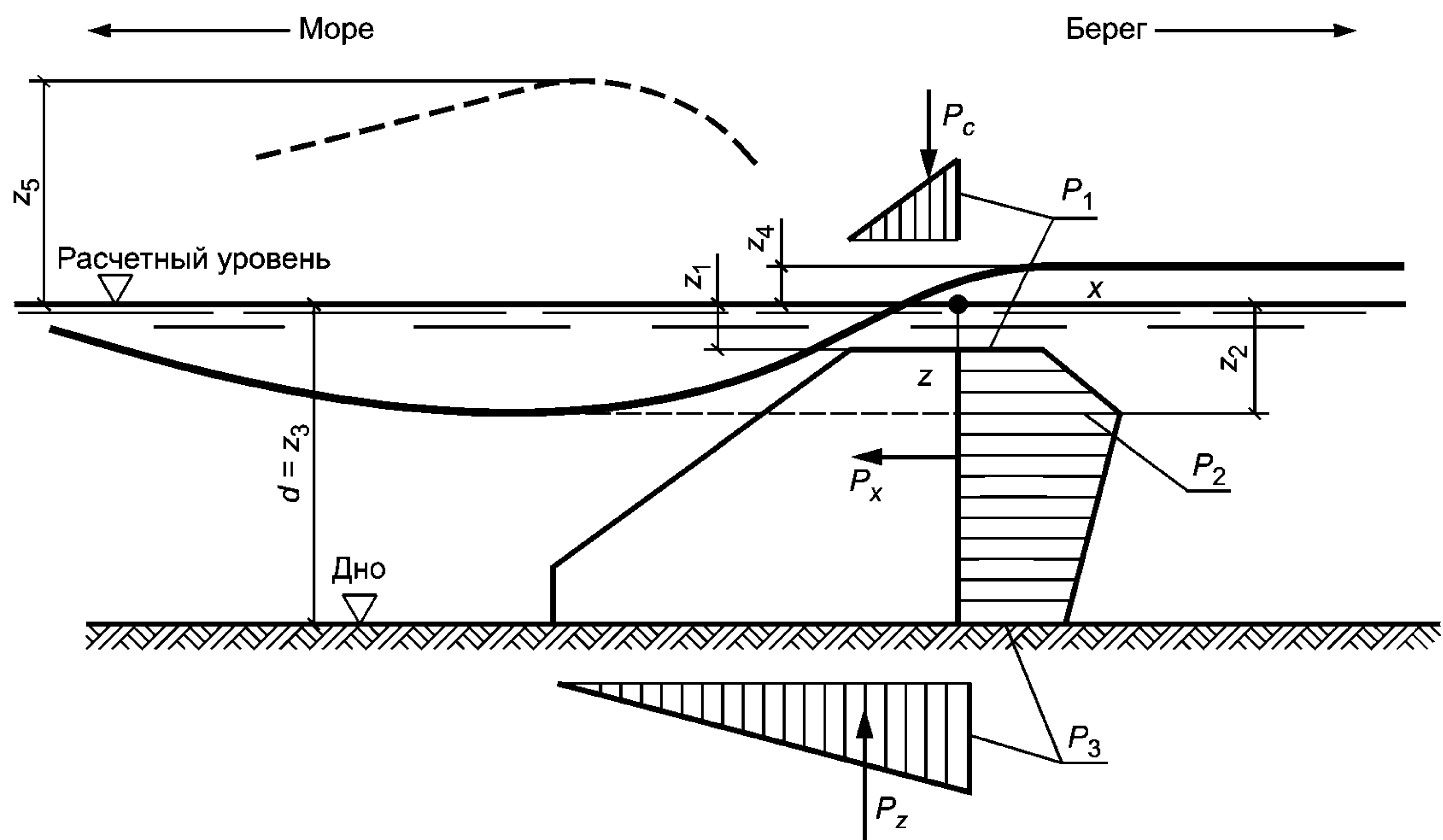
Рисунок 26 — Эпюры волнового давления на подводный волнолом
