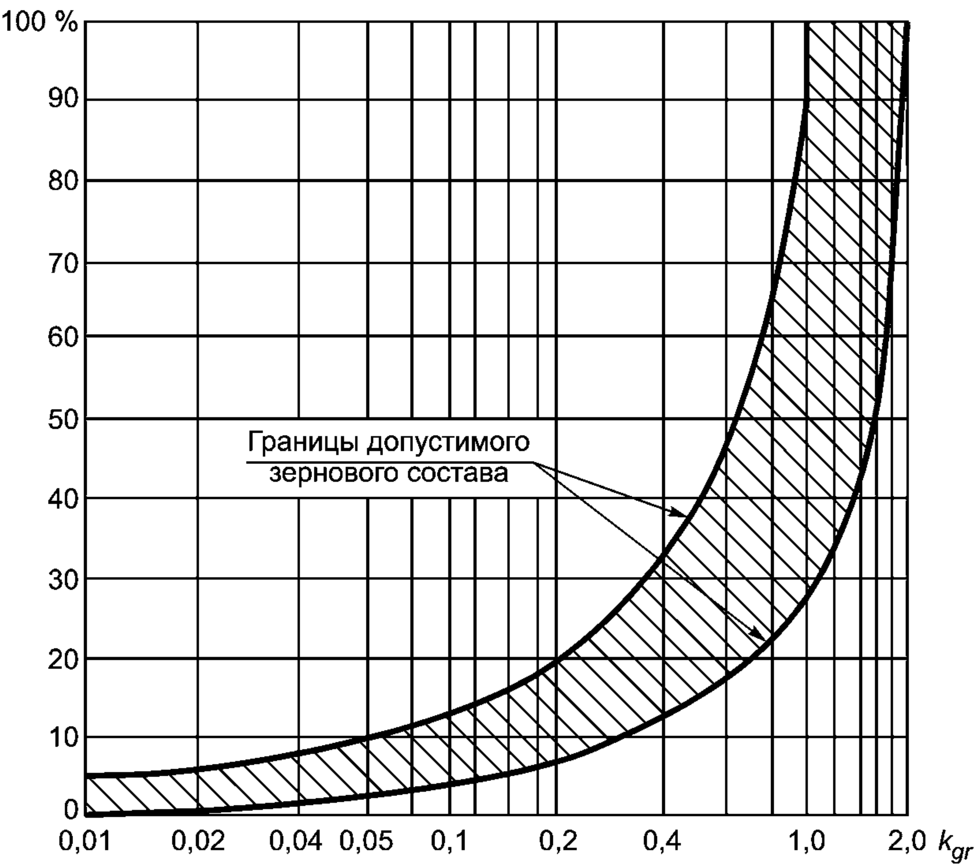
Рисунок 13 — График для определения допустимого зернового состава несортированной каменной наброски для крепления откосов
