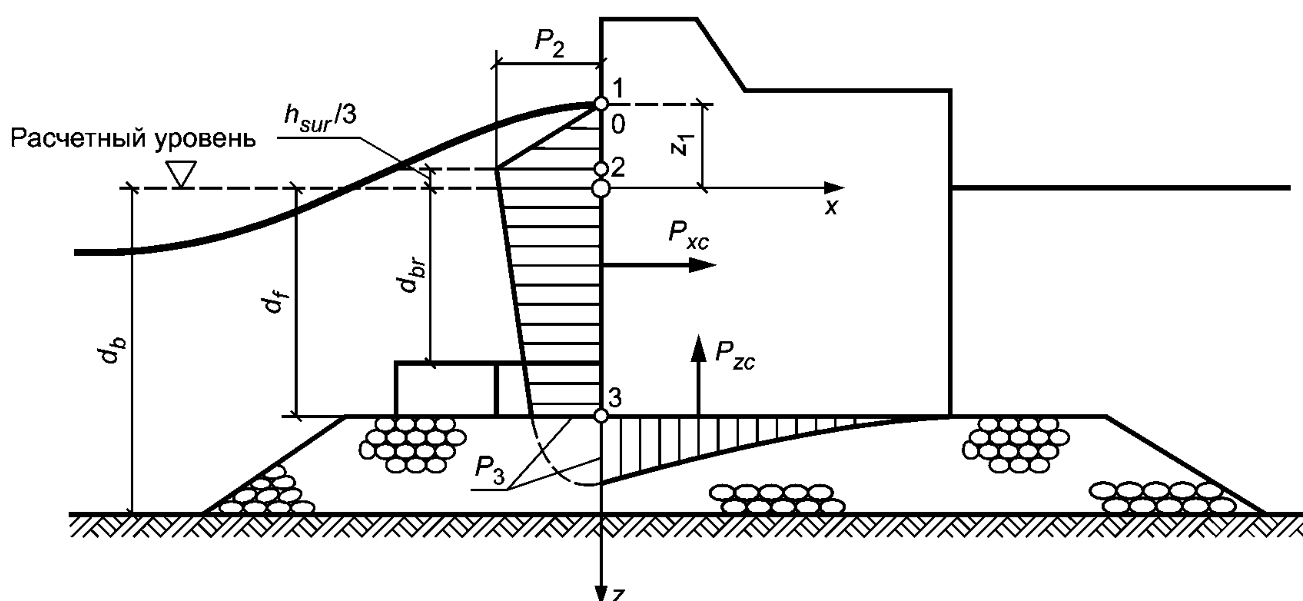
Рисунок 8 — Эпюры давления разбивающихся волн на вертикальную стену
