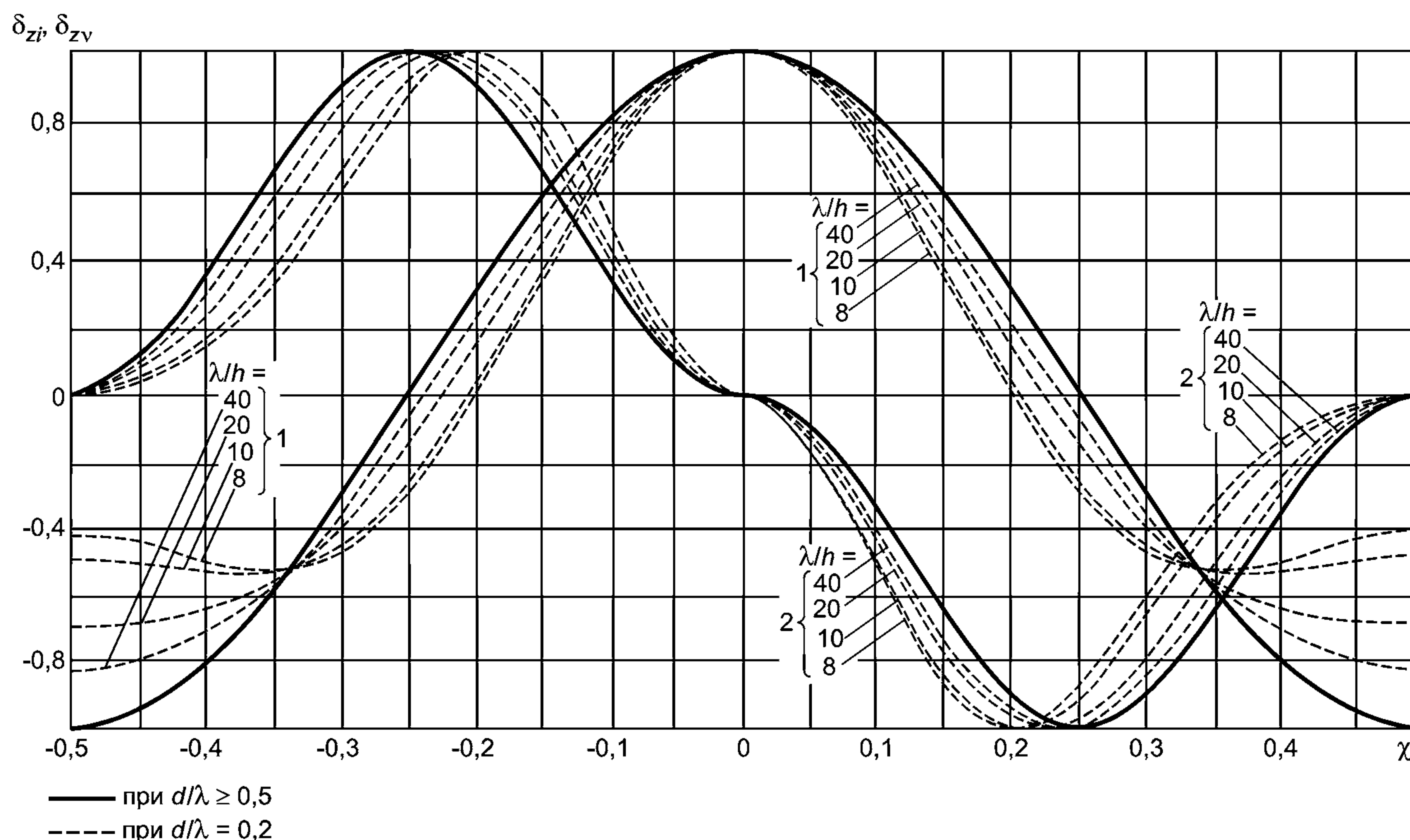
Рисунок 23 — Графики значений коэффициентов сочетания \delta_{zi} инерционного (график 1) и \delta_{zv} — скоростного (график 2) компонентов вертикальной линейной нагрузки от волн
