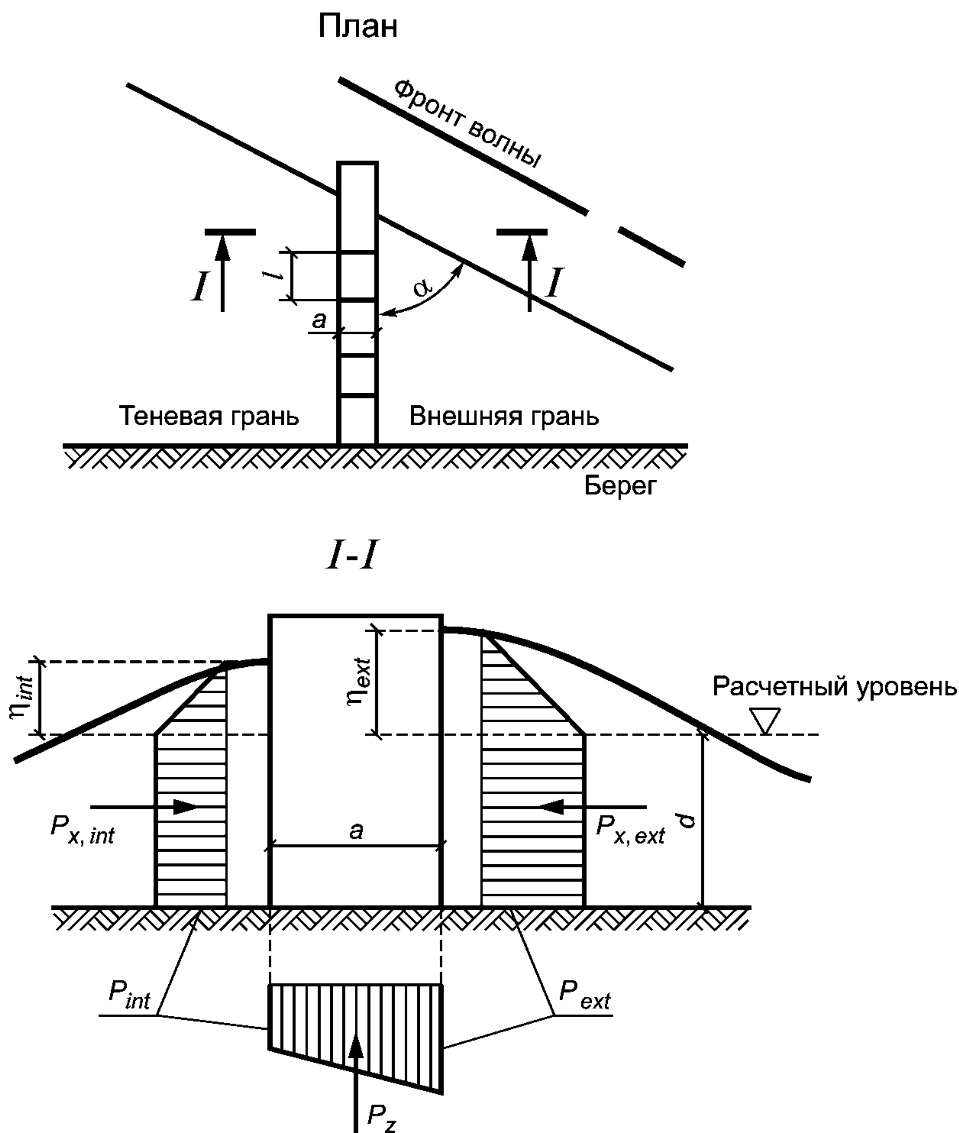
Рисунок 30 — Эпюры волнового давления на буну
