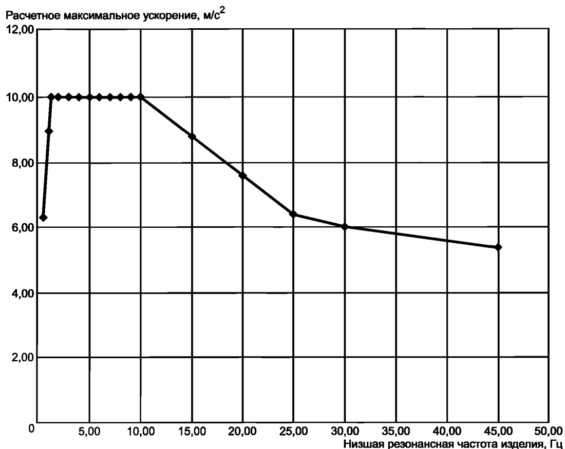
Рисунок 2 — Обобщенный спектр ответа для расчетных оценок сейсмостойкости с использованием ЛСТ (горизонтальное направление, 9 баллов по MSK-64)
