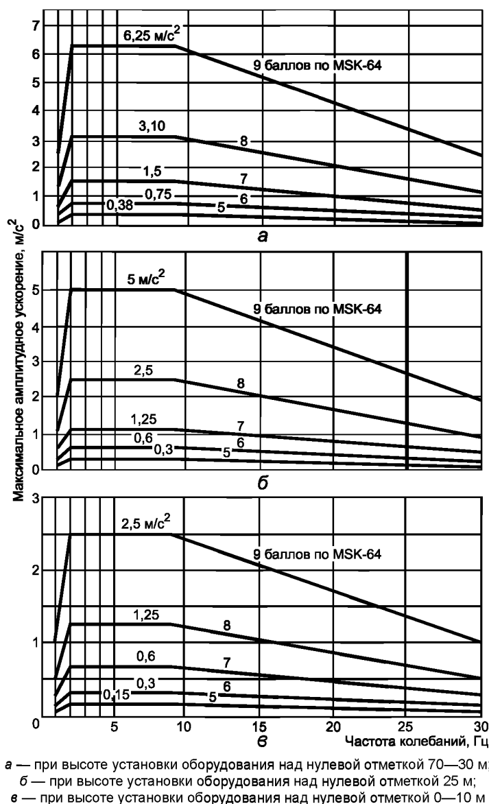
Рисунок 1 — Зависимость между максимальной амплитудой ускорения и частотой синусоидальной вибрации (горизонтальное направление)
