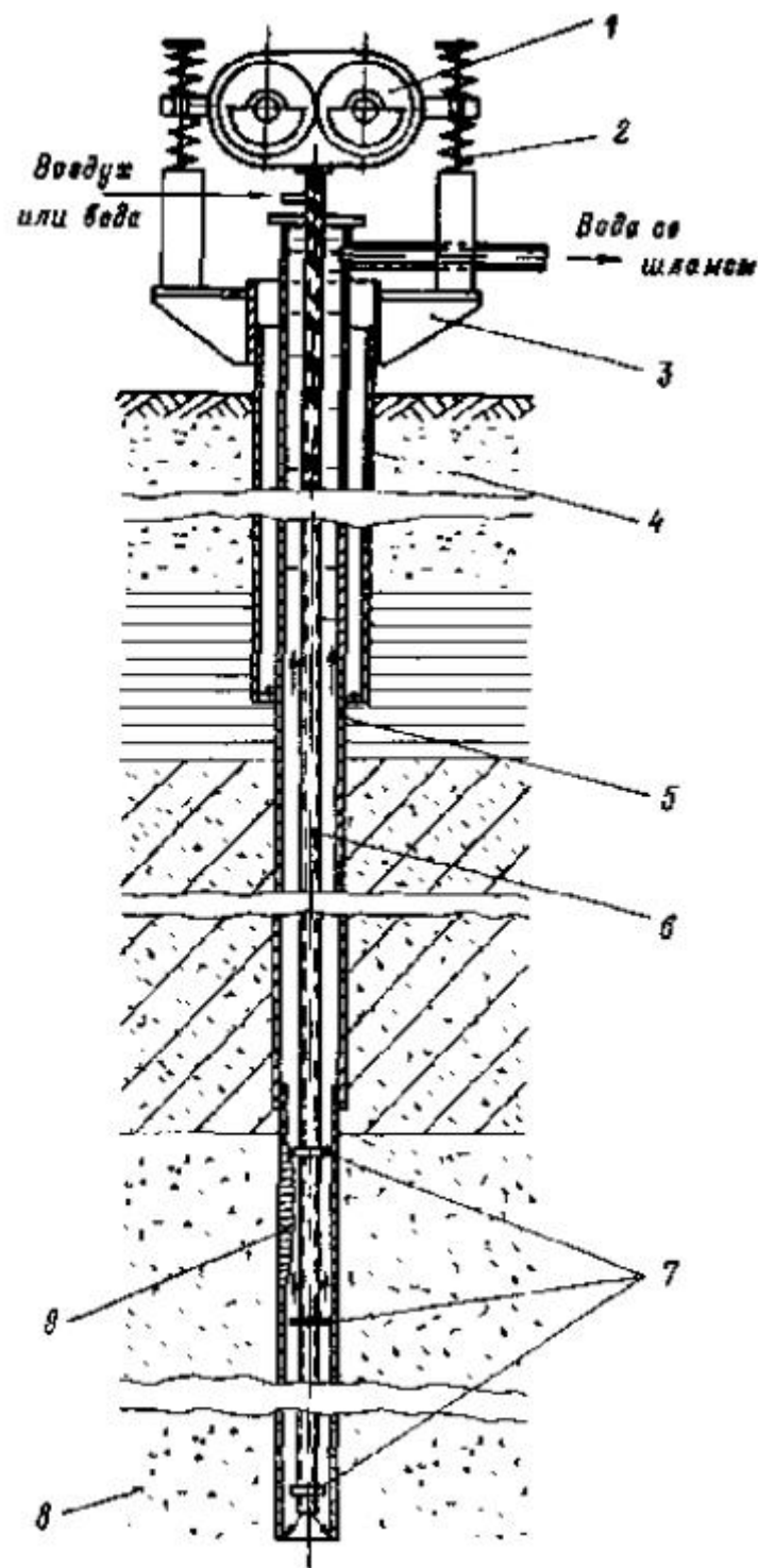
Рис. 6. Схема вибрационной гидродинамической обработки скважин на воду при их разглинizations:
