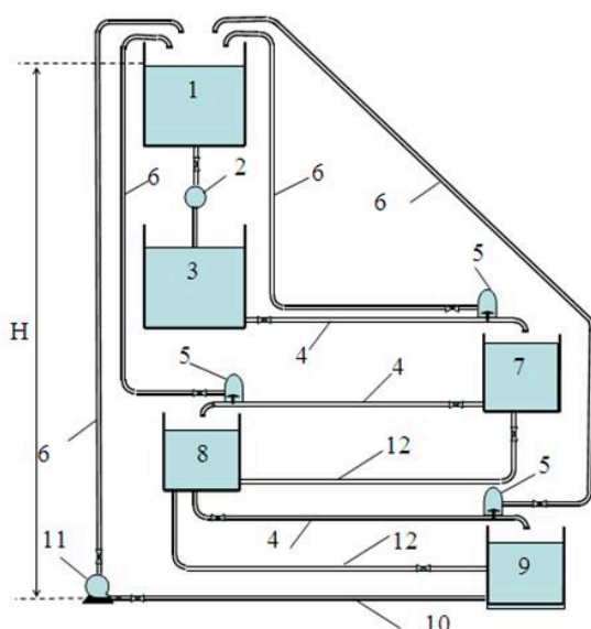
Рис. 14. Схема ГАЭУ с гидравлическими таранами
