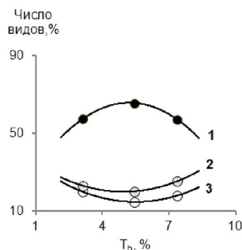
Рис. 6. Полиномиальные тренды по данным 1990–2000 гг.: 1 – H ; 2 – ( T + T h ); 3 – T
