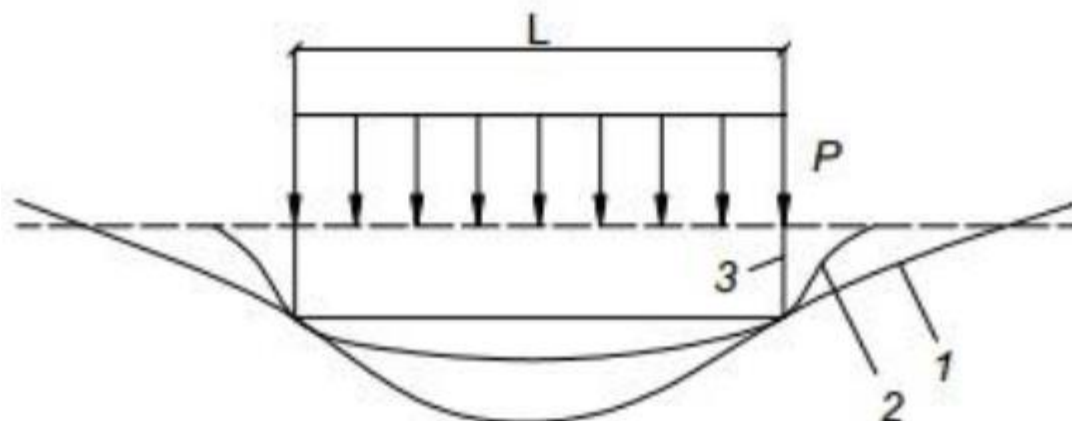
Рис.2. Характер прогиба поверхности грунта при действии полосовой нагрузки. 1- упругое полупространство; 2- нелинейно-деформируемое полупространство; 3- модель местных упругих деформаций.
