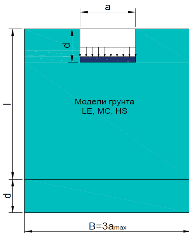
Рис. 1. Расчетная схема для моделей грунта
