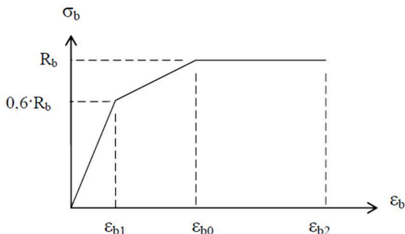
Рис. 4. Трехлинейная диаграмма « \sigma_b – \epsilon_b » по СП [40, 34].
