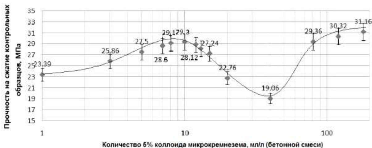
Рис. 4 - Влияние микроколичеств высокодиспергированного микрокремнезема на прочность при сжатие контрольных образцов мелкозернистого бетона при В/Ц=0,4 (без пластифицирующих добавок)
