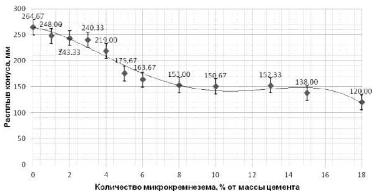
Рис.1 - Влияние микрокремнезема на расплыв конуса на встряхивающем столике ( V/C=0,4 ).
