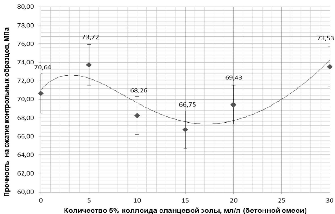
Рис. 3.8 – График зависимости прочности контрольных образцов от количества 5% коллоида сланцевой золы.
