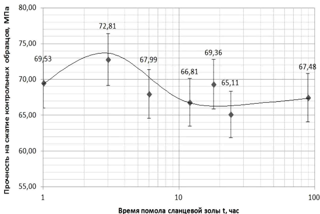
Рис. 6 – График зависимости прочности контрольных образцов от времени помола сланцевой золы
