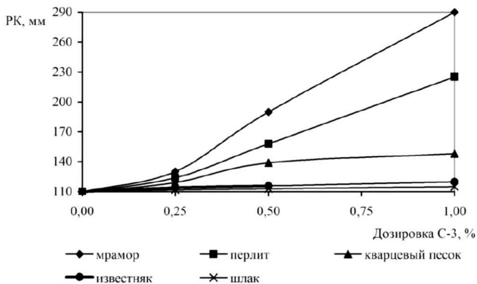
Рисунок 1. - Влияние вида заполнителя на разжижающую способность суперпластификатора С-3
