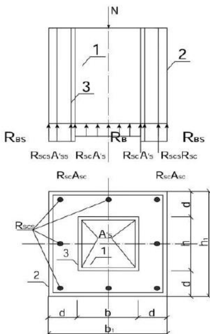
Рис.3.1. Схема центрально сжатого железобетонного элемента, усиленного железобетонной облоймой 1 – усиливаемый железобетонный элемент; 2 – железобетонная облойма; 3 – поверхность сцепления нового бетона со старым (зачистка, насечка, адгезионная обмазка);
