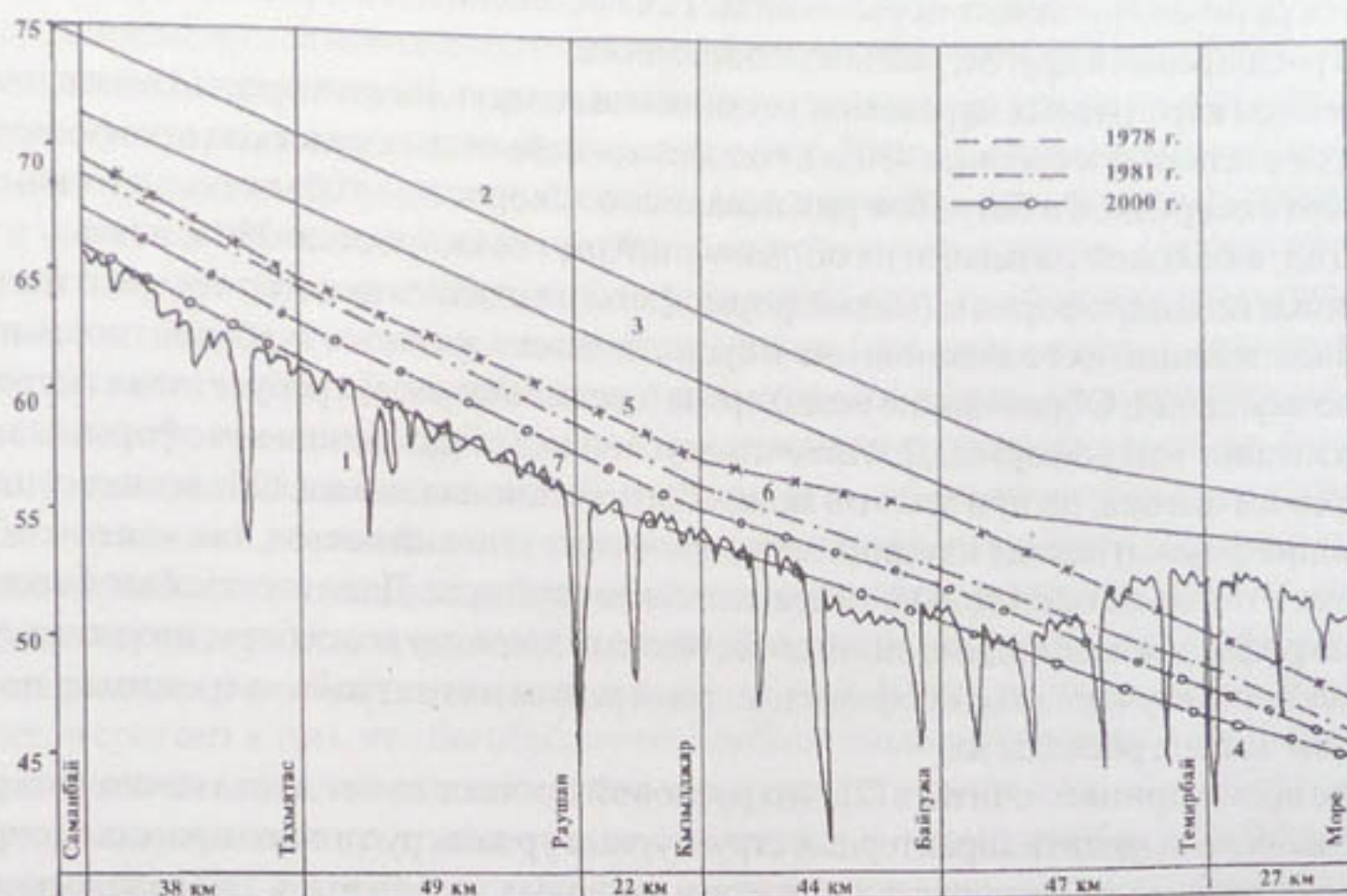
Рис. 2. Изменение вдоль нижнего течения р. Амударья отметок дна (1) и водной поверхности в половодье (2) и меле (3) при бытовом состоянии, а также отметок дна (4) и водной поверхности (5, 6, 7) при зарегулированном стоке.
