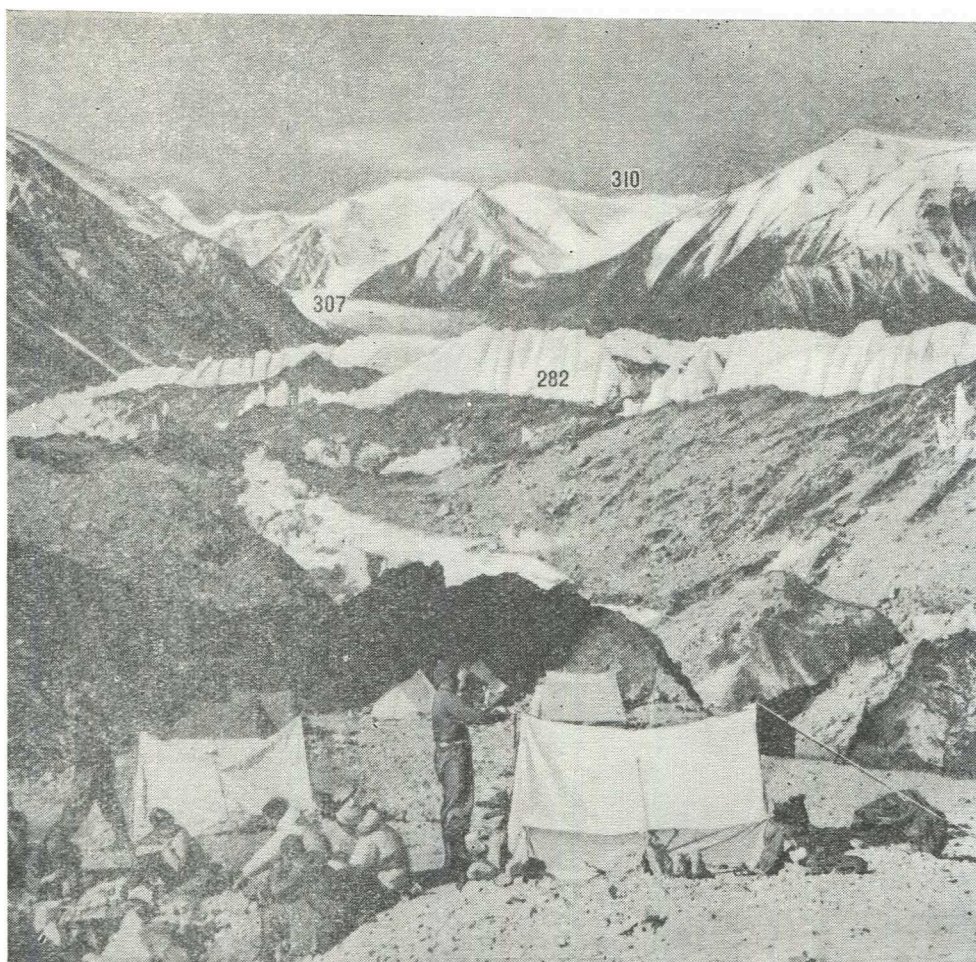
Рис. 10. Оледенение верховьев р. Сауксай. На переднем плане язык ледника Большой Саукдара (№ 282), на заднем — ледник Северный Зулумарт (№ 307). Фото В. И. Рацика.
