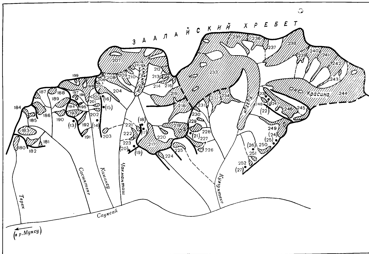
Рис. 19. Схема расположения ледников в бассейнах рек Терек, Сасыктеке, Камансу, Чакманташ и Кузгунтеке. Усл. обозначения см. на рис. 18.
