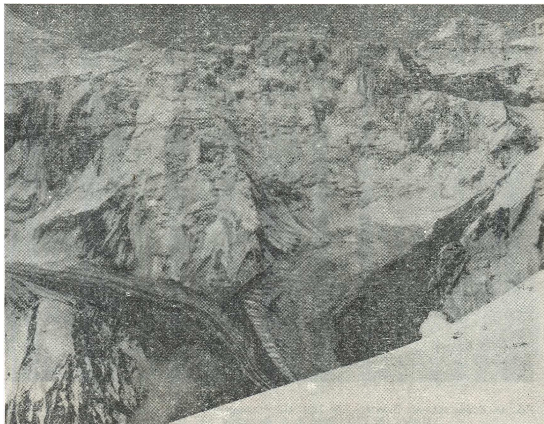
Рис. 45. Слияние ледников Вальтера (№ 730) и Москвина. Фото Г. В. Калинина.
