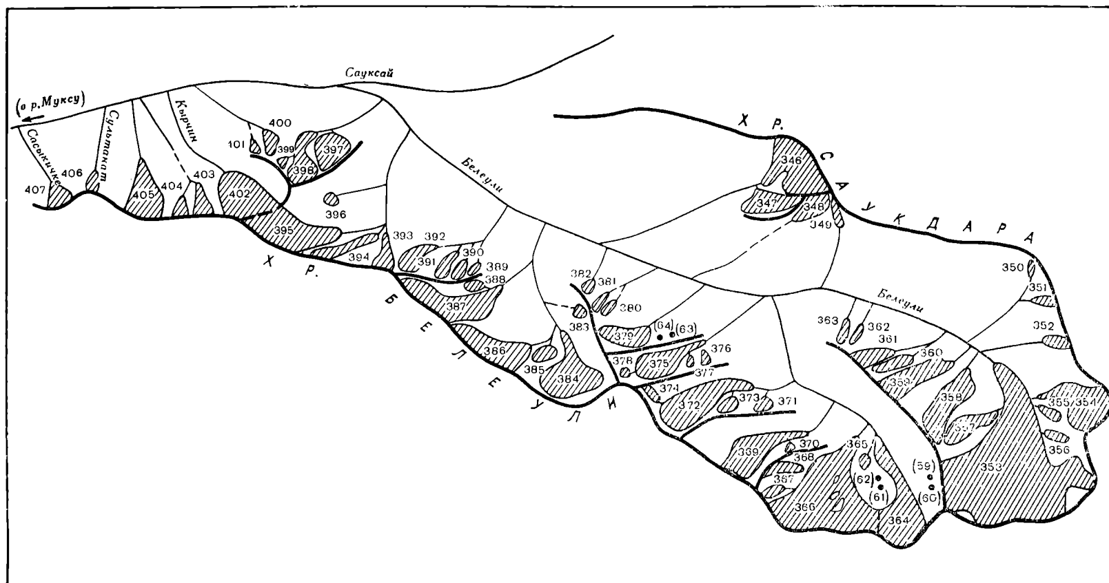
Рис. 22. Схема расположения ледников в бассейнах р. Белеули и левых притоков р. Сауксай. Усл. обозначения см. на рис. 18.
