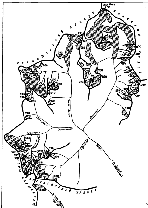
Рис. 34. Схема расположения ледников в бассейне реки Ясмай и в верховьях р. Ярхыч. Усл. обозн. см. на рис. 30.
