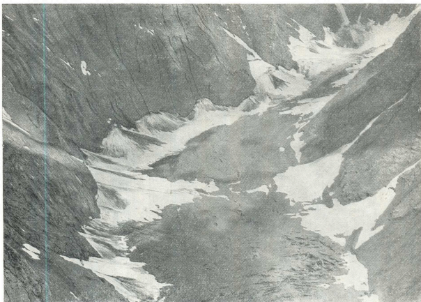
Рис. 19. Долинный ледник туркестанского типа (№ 276).
