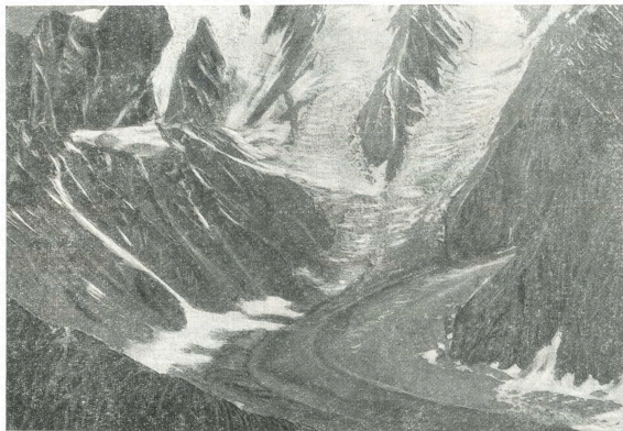
Рис. 23. Ледниковые притоки правой составляющей дендритового ледника Иштансалды (№ 392).
