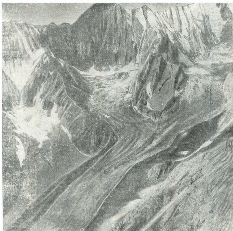
Рис. 21. Сложный долинный ледник Дыдадь (№ 513) на северном склоне хр. Петра Первого.
