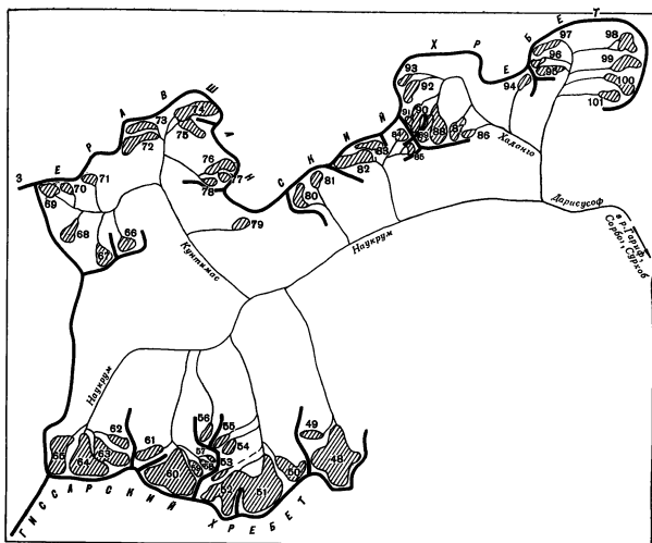
Рис. 31. Схема расположения ледников в бассейне р. Наурум.
