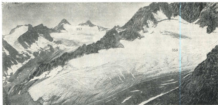
Рис. 14. Долинный ледник № 359 с простым однокамерным бассейном питания и долинный ледник № 357 с расширенным бассейном питания.
