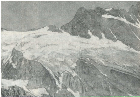
Рис. 48. Склоновый ледник № 223 с ровной, широкой областью аккумуляции. (Большая часть области абляции находится на левом, пологом языке ледника.)
