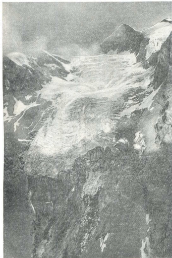
Рис. 18. Висячий долинный ледник № 451.
