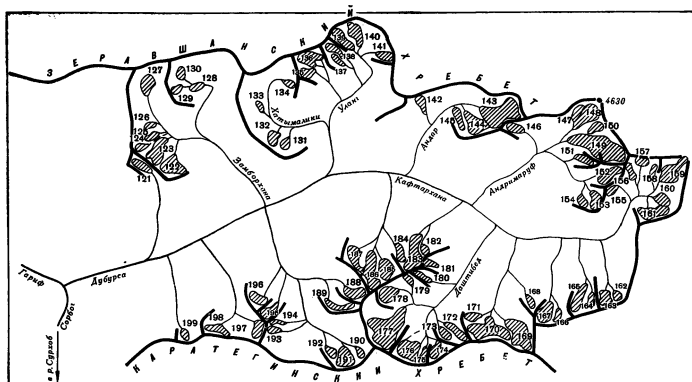
Рис. 32. Схема расположения ледников в бассейне р. Дубурса.
