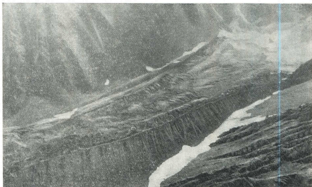
Рис. 22. Язык долинного ледника № 503, заваленный мореной (северный склон хр. Петра Первого).
