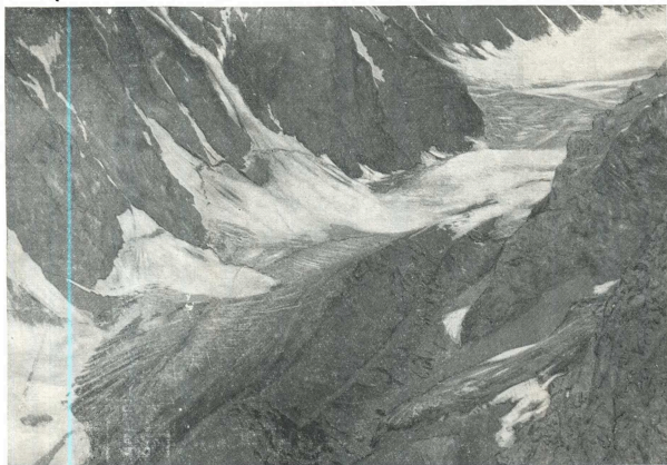
Рис. 45. Лавинный снег — дополнительное питание долинного ледника Чайнак (№ 407), бассейн р. Агуюрма.
