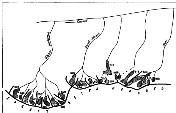
Рис. 39. Схема расположения ледников в бассейнах нижних левых притоков р. Сурхоб.
