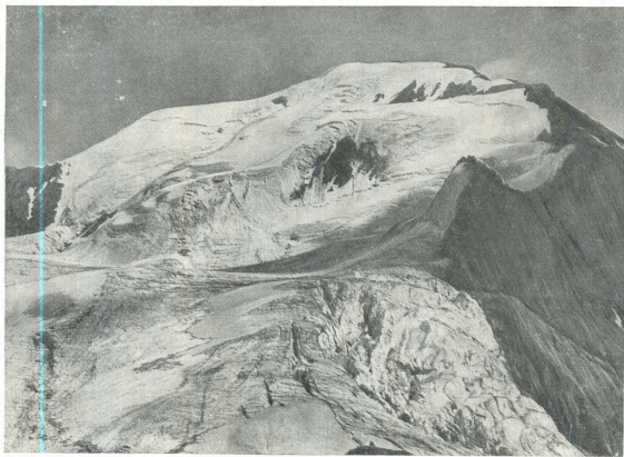
Рис. 46. Складной ледник № 420 покрывает сверху донизу северо-западный склон массива, возвышающегося слева над языком ледника Янгидаван. На снимке не виден лишь узкий тонкий язык ледника — приток ледника Янгидаван.
