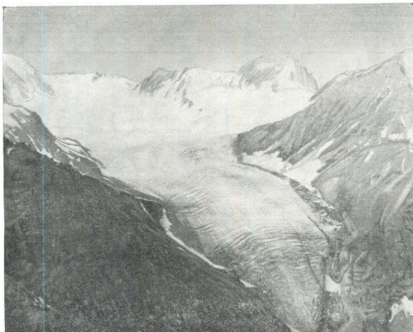
Рис. 13. Долинный ледник № 48.
