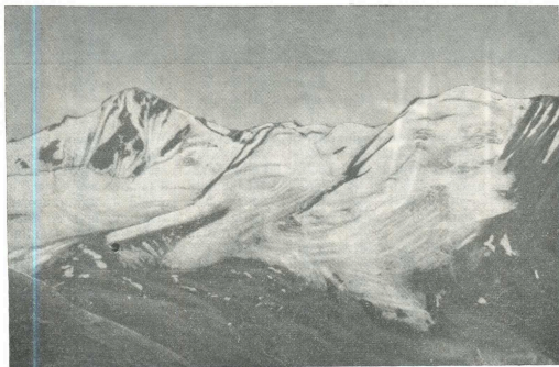
Рис. 27. Склоновый ледник № 480.
