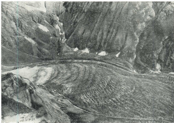
Рис. 16. Поверхность языка ледника № 108 в средней его части.
