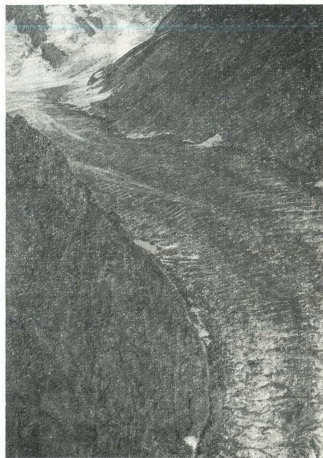
Рис. 24. Средняя часть языка сложного долинного ледника Тамдыкуль (№ 388).
