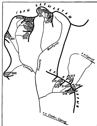
Рис. 33. Схема расположения ледников в бассейне р. Комару. Усл. обозн. см. на рис. 30.
