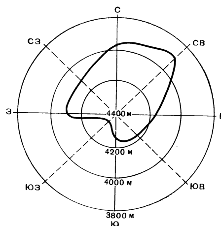
Рис. 4. Высотное положение фирновой линии на ледниках различной экспозиции.
