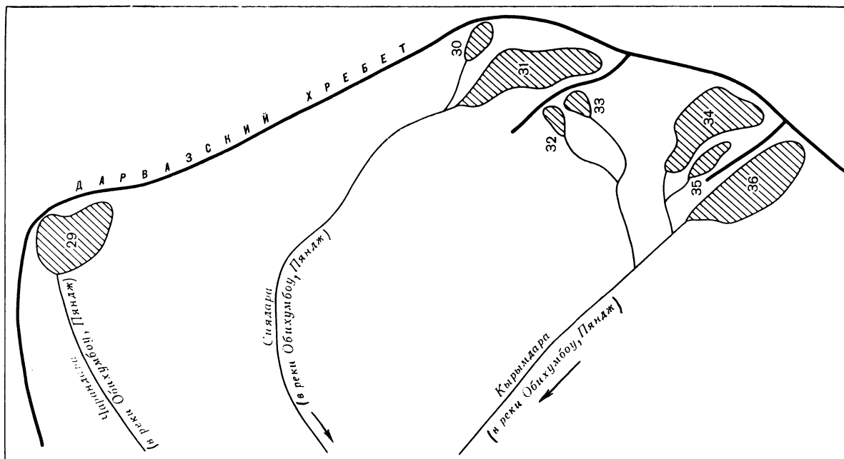
Рис. 8. Схема расположения ледников в бассейне р. Обихумбоу. Усл. обозначения см. на рис. 6.
