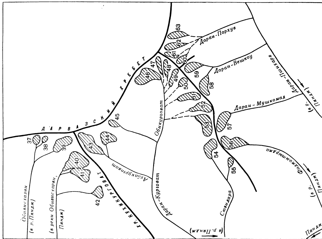
Рис. 9. Схема расположения ледников в бассейнах рек Обивисхарви, Даран-Курговат, Филджомтырджы и Даран-Пшихарв. Усл. обозначения см. на рис. 6.
