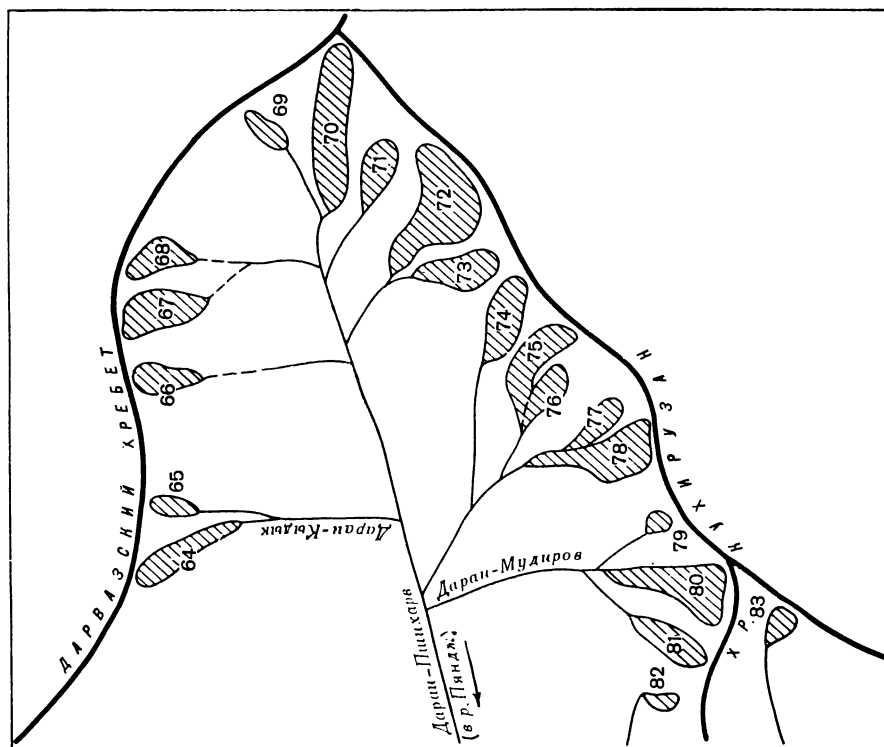
Рис. 10. Схема расположения ледников в бассейнах рек Даран-Пшихарв и Даран-Вурауз. Усл. обозначения см. на рис. 6.
