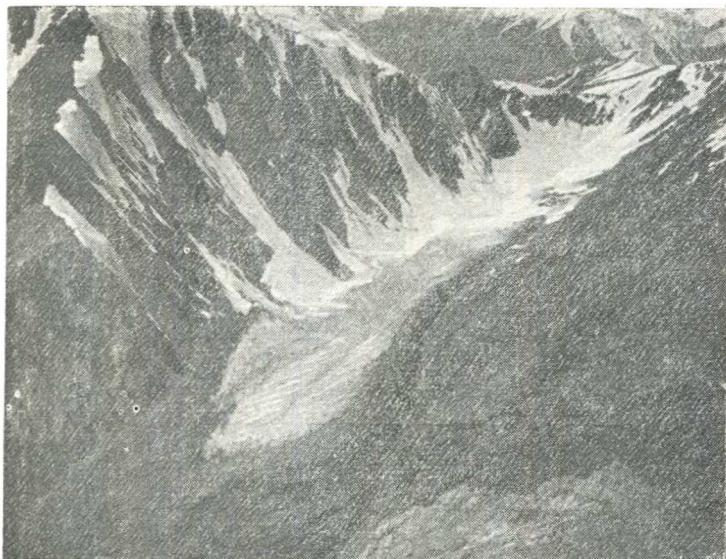
Рис. 18. Долинный ледник № 268 с преимущественно лавинным питанием.
