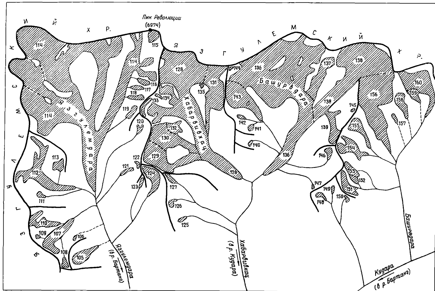
Рис. 15. Схема расположения ледников в верховьях рек Язгулемдара, Хабарвинхац и Башурвдара. Усл. обозначения см. на рис. 11.
