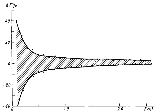
Рис. 1. Зависимость максимальной ошибки округления площади до 0,1 км² ( \Delta F\% ) от площади ледника F .
