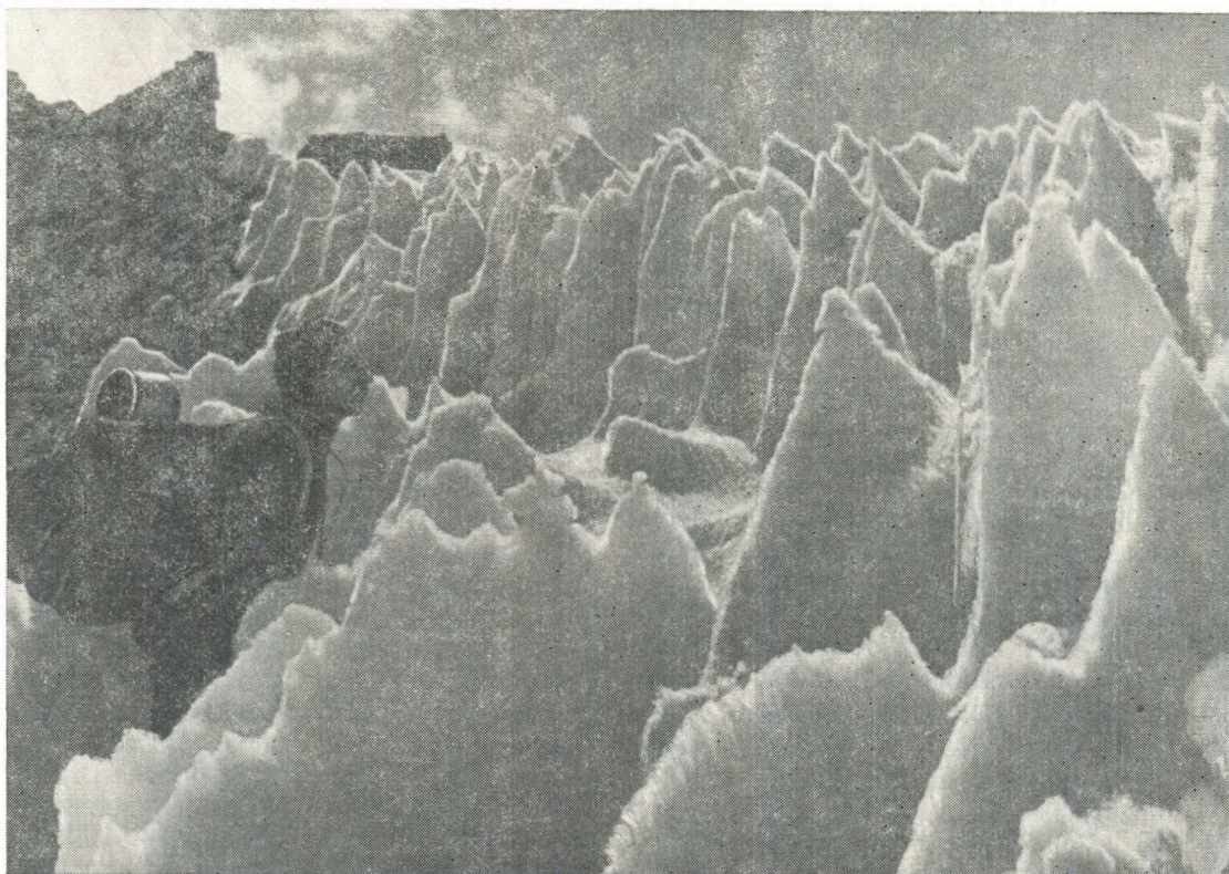
Рис. 6. Кальгаспоры на леднике Северный Танимас. Фото В. К. Ноздрихина.
