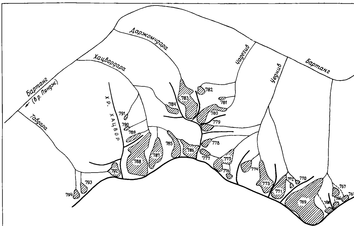
Рис. 31. Схема расположения ледников в бассейнах рек Уеднив, Чадегив, Даржомчдара, Хацвора и Тавдара. Усл. обозначения см. на рис. 11.
