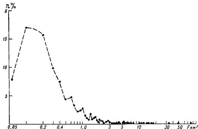
Рис. 4. Распределение числа ледников (n%) по величине их площади (F км²).
