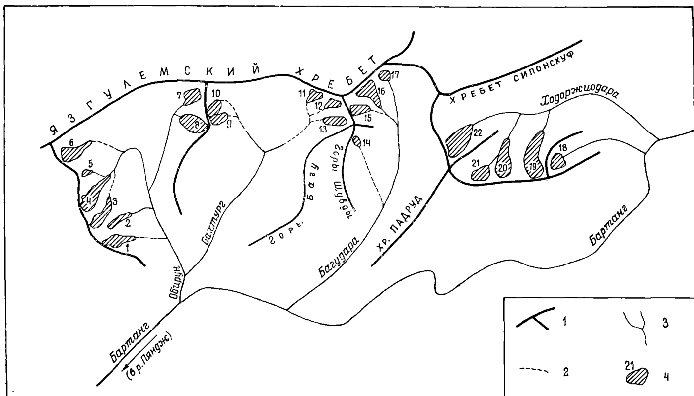
Рис. 11. Схема расположения ледников в бассейнах рек Обирун, Багудара и Ходоржиодара. 1 — водораздел, 2 — ледораздел, 3 — река, 4 — ледник и его номер по табл. 1.
