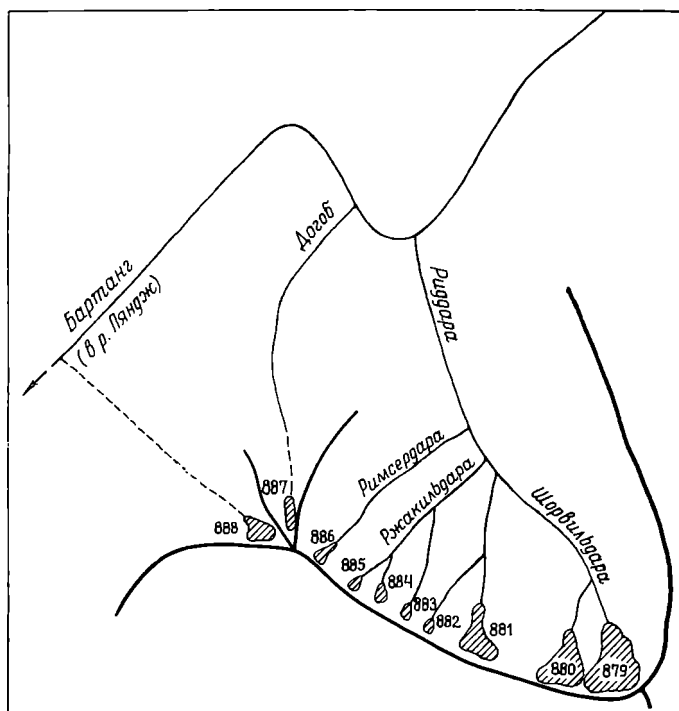
Рис. 34. Схема расположения ледников в бассейнах рек Риддара и Догоб. Усл. обозначения см. на рис. 11.
