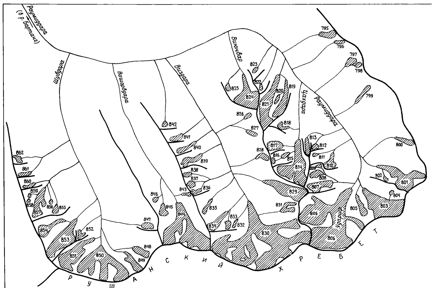
Рис. 32. Схема расположения ледников в бассейне р. Раумиддара. Усл. обозначения см. на рис. 11.
