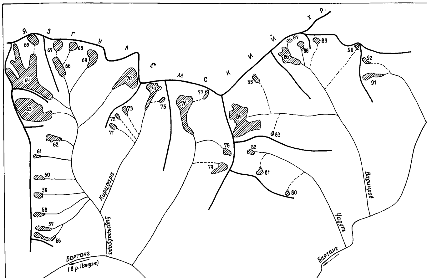
Рис. 13. Схема расположения ледников в бассейнах рек Биджравдара, Чадут, Вадинров и безымянных притоков р. Бартага. Усл. обозначения см. на рис. 11.
