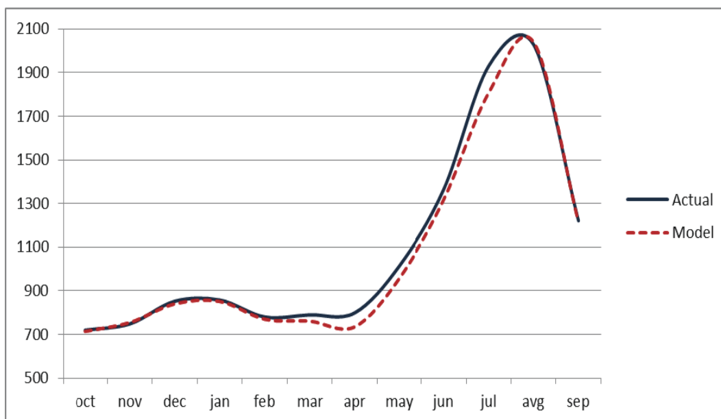
Рис. 13. Выработка электроэнергии на Нуρεкской ГЭС, в среднем за 2010-2016 гг.: сравнение фактических значений с расчетными, полученными с помощью модели
