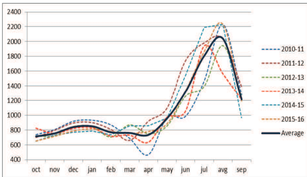
Рис. 12. Выработка электроэнергии на Нуρεкской ГЭС за 2010-2016 гг результаты расчетов на модели
