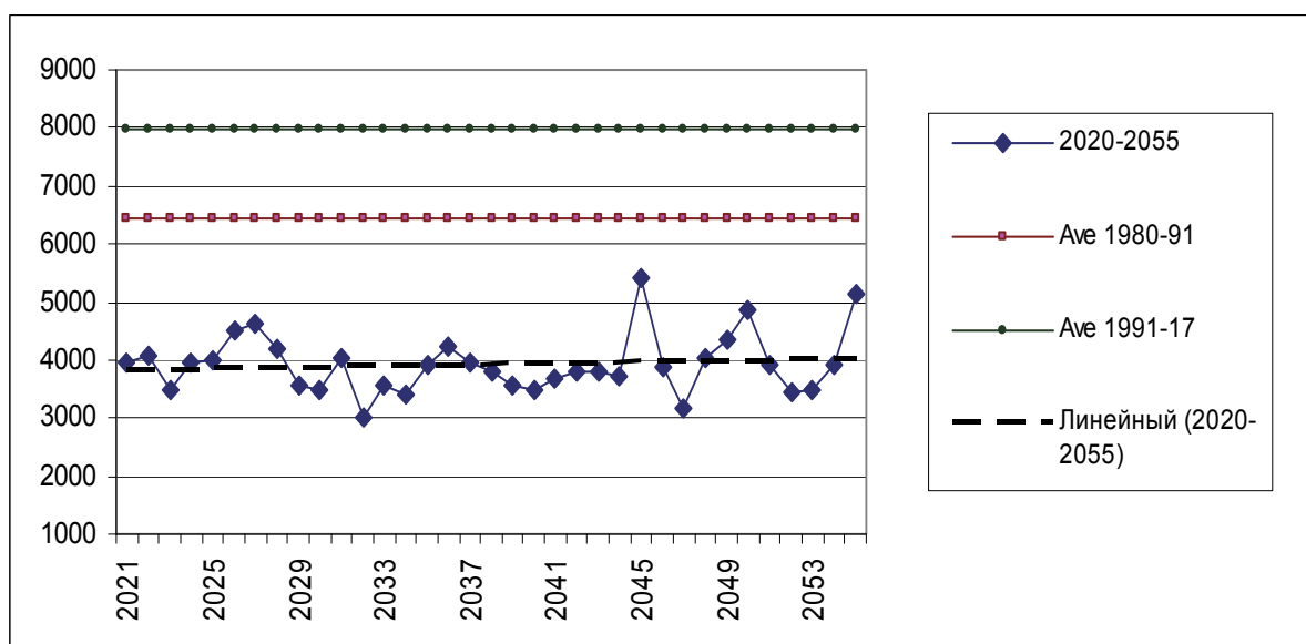
Рис. 103 Межвегетационные попуски из Нурекского г/у (октябрь-март), млн.м³: результаты расчетов на GAMS-модели (2020-2055 гг), в сравнении со средними попусками за 1980-1991 и 1991-2017 гг. Вариант 2. Энерго-ирригационный режим
