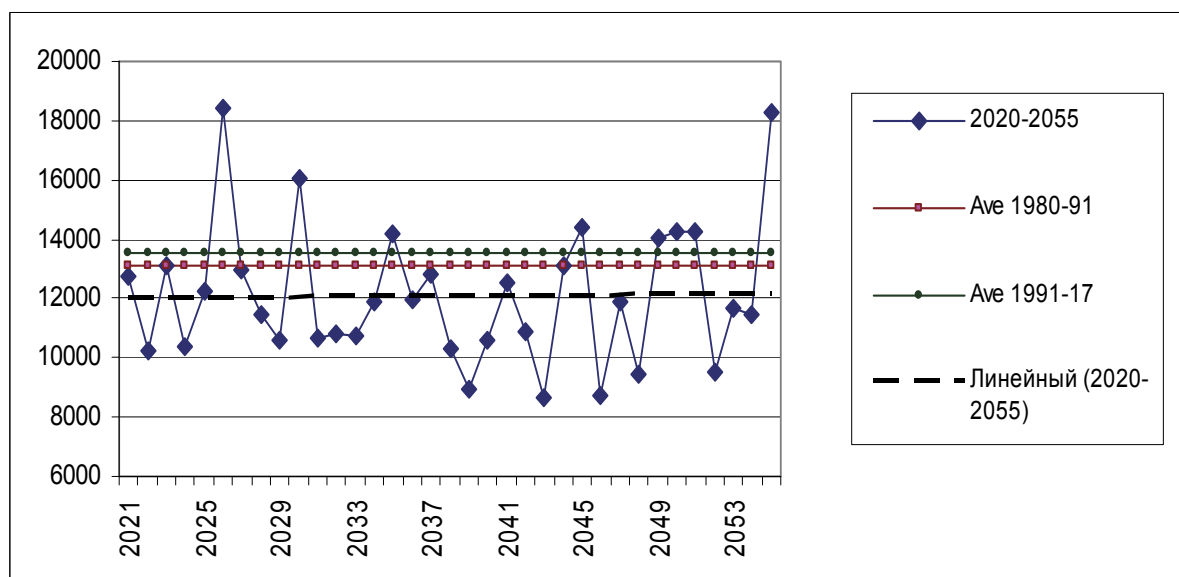
Рис. 101 Вегетационные попуски из Нурекского г/у (апрель-сентябрь), млн.м 3 : результаты расчетов на GAMS-модели (2020-2055 гг), в сравнении со средними попусками за 1980-1991 и 1991-2017 гг. Вариант 1. Энергетический режим
