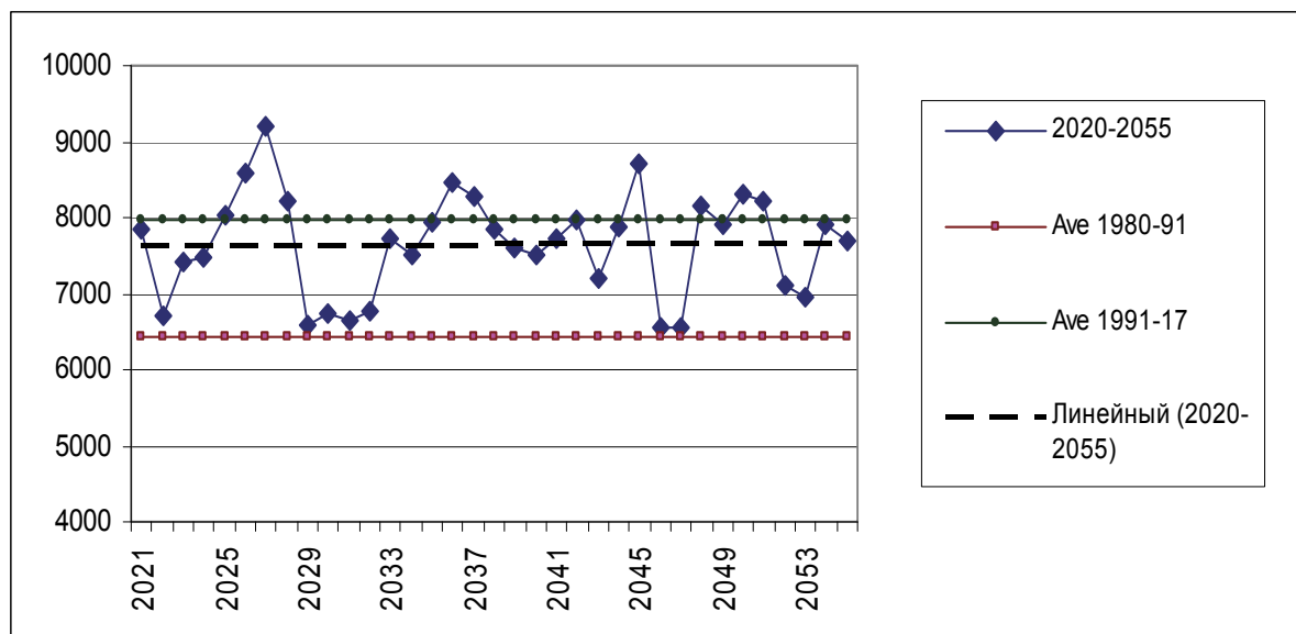
Рис. 100 Межвегетационные попуски из Нурекского г/у (октябрь-март), млн.м 3 : результаты расчетов на GAMS-модели (2020-2055 гг), в сравнении со средними попусками за 1980-1991 и 1991-2017 гг. Вариант 1. Энергетический режим
