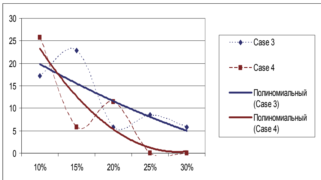
Рис 53 Зависимость глубины дефицита (D, %) от количества случаев их появления
