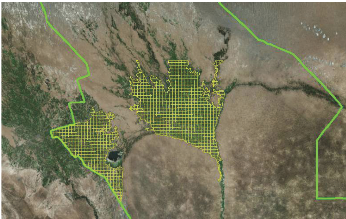
Рис. 65. Пример нанесения расчетной сетки на спутниковый снимок
