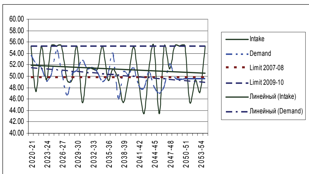
Рис. 61 Динамика требуемого водопотребления и водозабор в бассейне Амударьи на 2020-2055 гг. (км³); сочетание сценариев: ESA + Case 3
