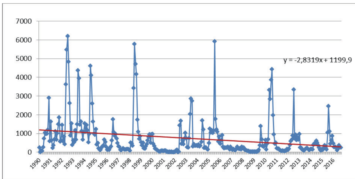
Рис. 38. Динамика притока воды в Аральское море, млн. \text{м}^3/\text{мес}
