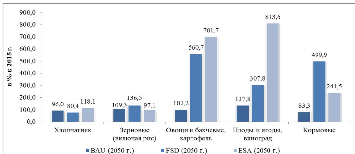
Рис. 74. Прогноз изменения роста производства основных видов сельхозкультур до 2050 г. в туркменской части бассейна Амударьи
