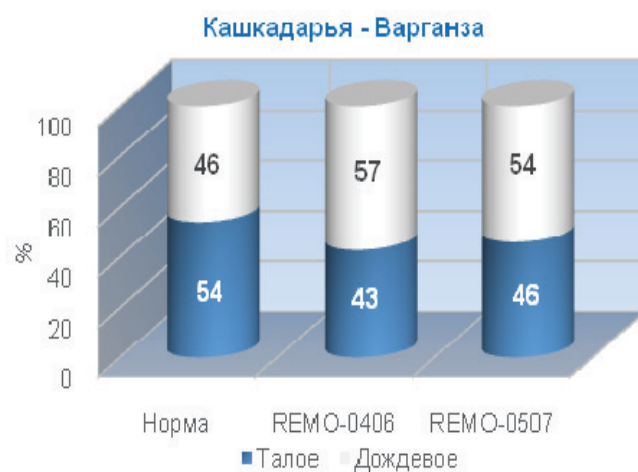
Рис. 67. Соотношение поступлений на водосбор реки Кашкадарья за апрель-сентябрь по климатическим сценариям REMO на 2050 год
