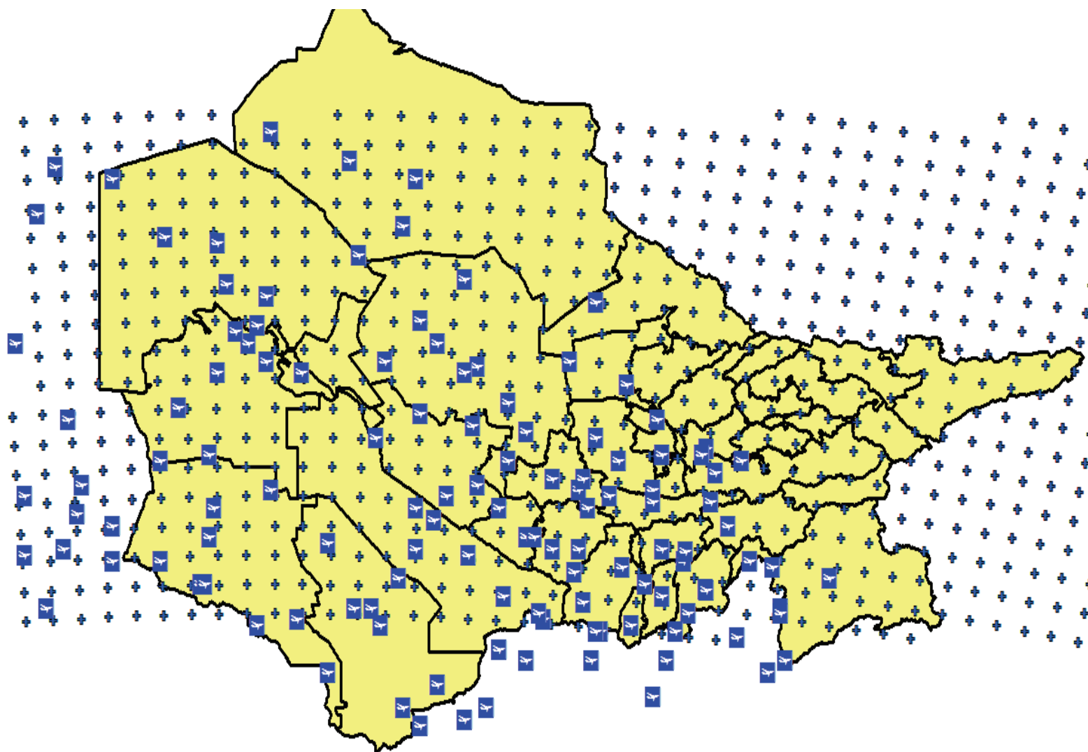
Рис. 64. Пример применения расчетной сетки для ЗП Мары с нанесением авиационных метеостанций
