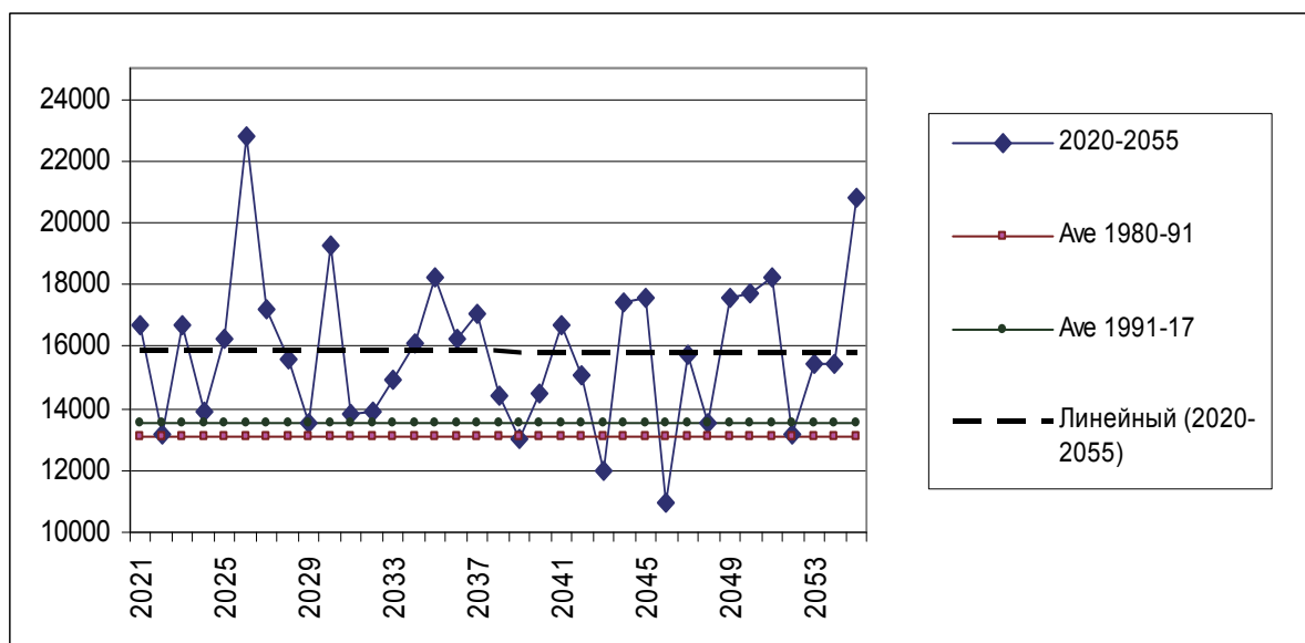
Рис. 102 Вегетационные попуски из Нурекского г/у (апрель-сентябрь), млн.м³: результаты расчетов на GAMS-модели (2020-2055 гг), в сравнении со средними попусками за 1980-1991 и 1991-2017 гг. Вариант 2. Энерго-ирригационный режим
