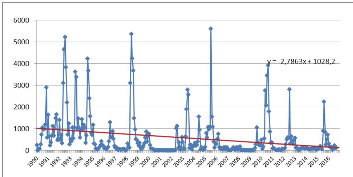
Рис 37 Динамика стока реки Амударья в г/п Саманбай, млн. \text{м}^3/\text{мес}
