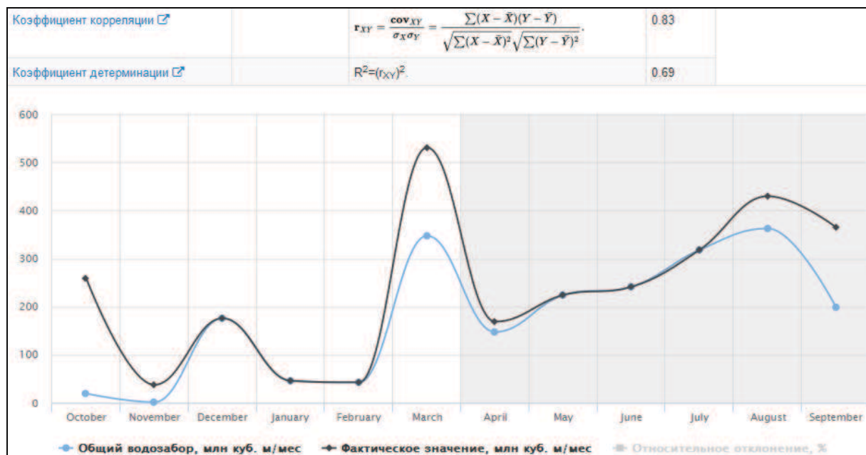
Рис. 10 Сравнение графиков расчетного и фактического водозабора после корректировки исходных данных (калибровки) для Хорезмской ЗП, 2011 год
