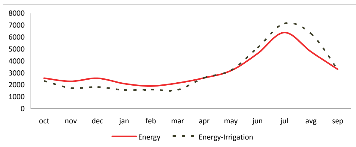
Рис. 44. Гидрограф стока реки Амударья в створе выше водозабора в Гарагумдарью (г/п Келиф) для особо маловодного года (2042-2043 г) для вариантов: case 1 (энергетический) и case 2 (энерго-ирригационный), млн.м³/мес
