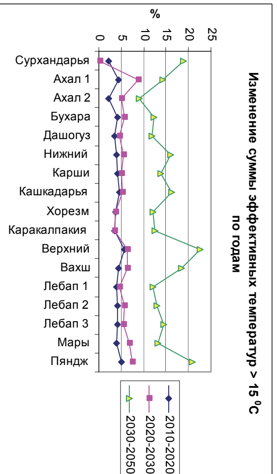
Рис. 111. Изменение термического потенциала в бассейне р. Амударья
