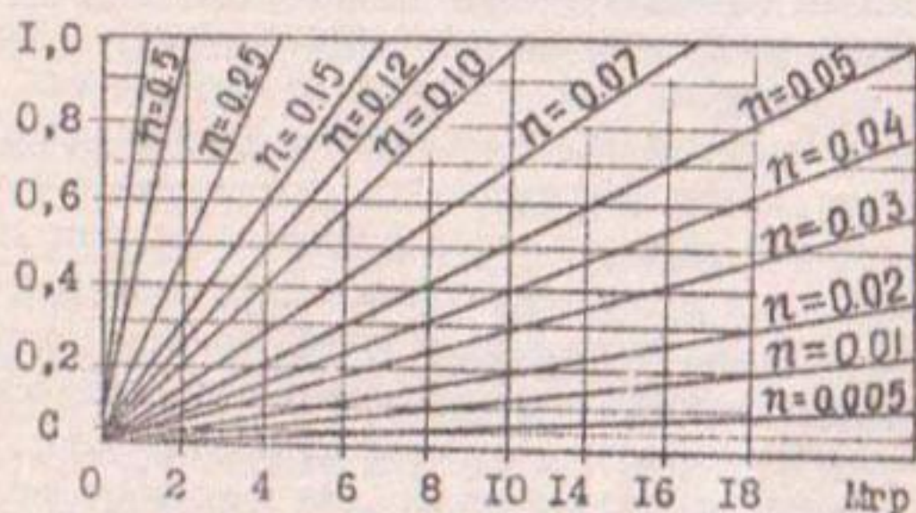
Рис. 2. Графики отношения ( ) засоления почвогрунтов ( C, \% ) к минерализации грунтовых вод ( M_{гр}, г/л )
