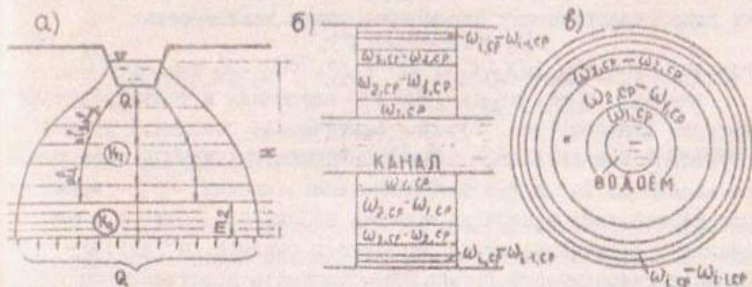
Рис. I. Расчетные схемы для определения параметров по фактической форме водяного "бутора" возле каналов (а, б) и водоемов (а, в): а — разрез; б, в — план
