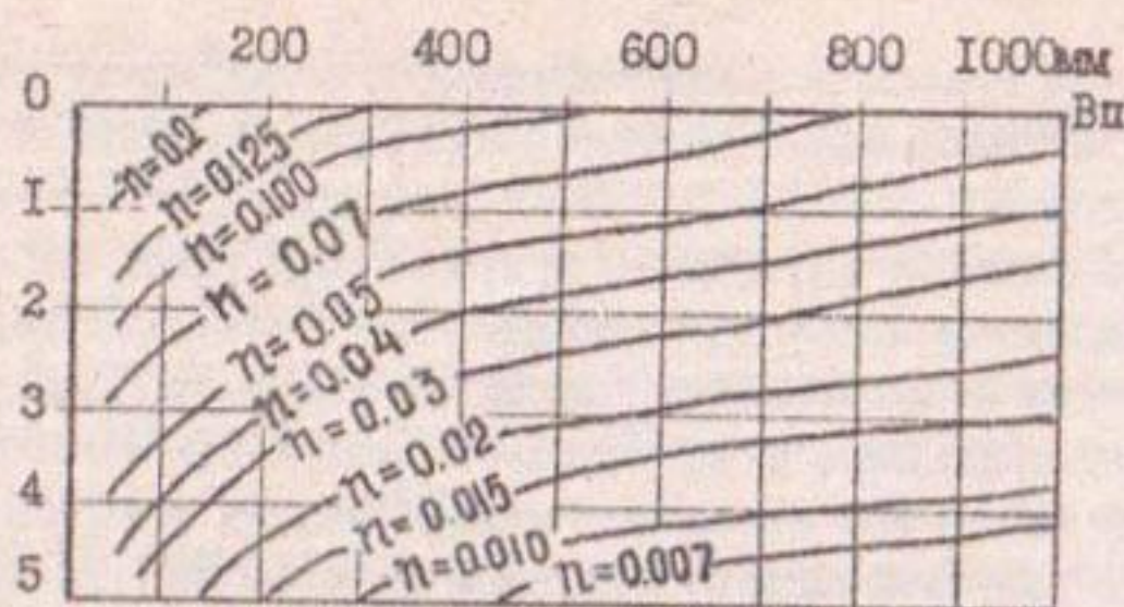
Рис. 1. Графики взаимосвязи между содержанием солей в грунтах, грунтовых водах, глубиной до уровня грунтовых вод и водопоступлением за год ( B_{п} )
