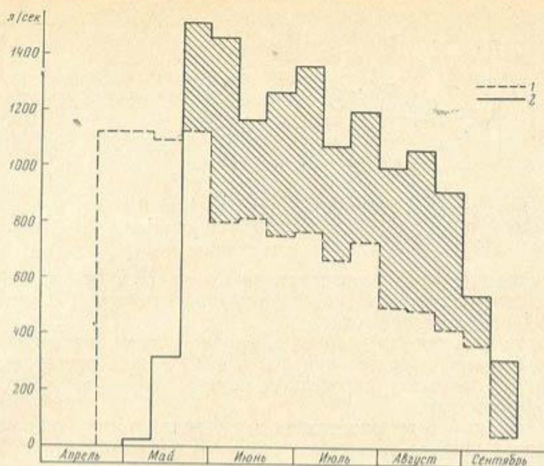
Рис. 1. Плановый (1) и фактический (2) расход воды по каналу Ш-1 в 1950 г.
