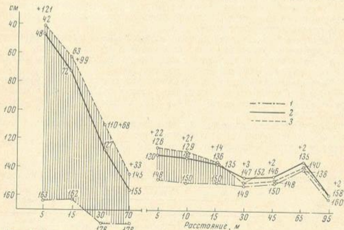
Рис. 6. Перехватывающее влияние дренажа, ограничивающей рисовый участок (Золотая Орда)
