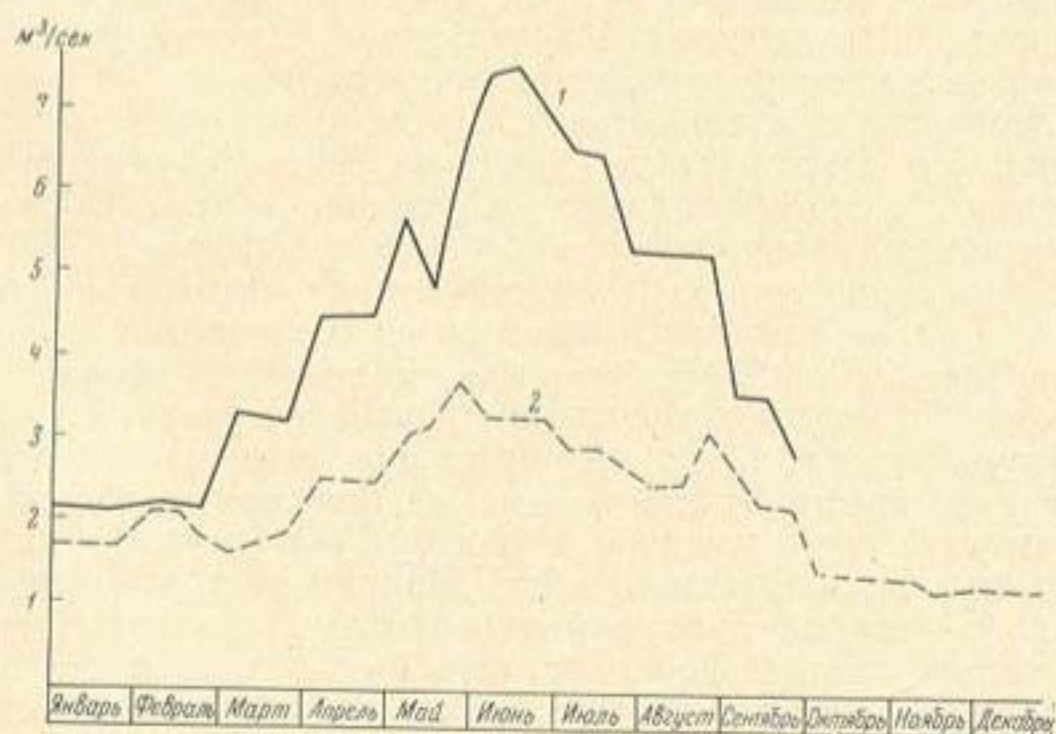
Рис. 3. Расход воды по коллектору Шурузяк.
