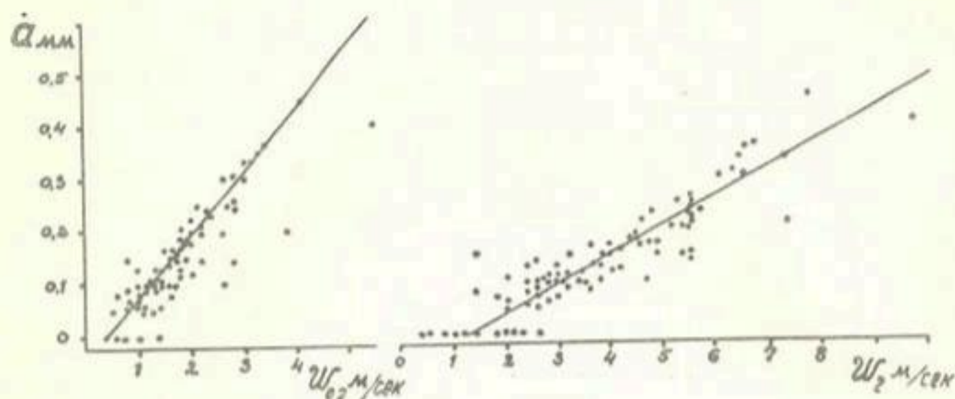
Рис.2. График связи между скоростью ветра ( W ) и амплитудой вертикальных перемещений плавающей системы ГПИ ( a )
