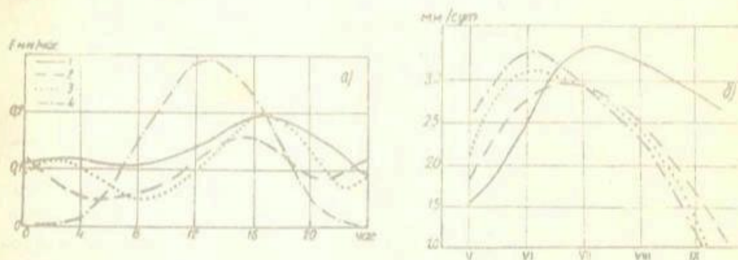
Рис. 1. Суточный (а) и сезонный (б) ход испарения с водной поверхности. 1 — озеро; 2 — бассейн площадью 20 м 2 ; 3 — испаритель ГГИ-3000; 4 — луг.
