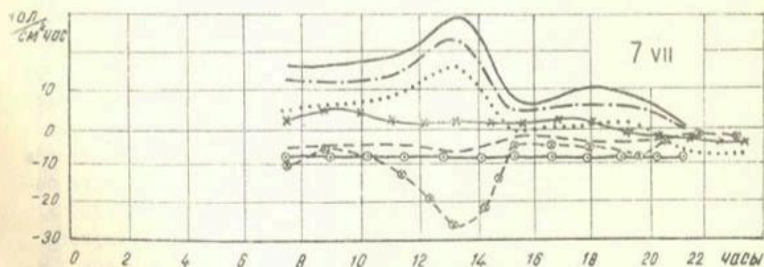
Рис. I. Суточный ход элементов теплового баланса. 1 - суммарная радиация ( S + D ), 2 - отраженная радиация R , 3 - баланс коротковолновой радиации Q_k , 4 - радиационный баланс Q_\delta , 5 - эффективное излучение E_{эф} , 6 - поток тепла в почву Q_n , 7 - суммарное испарение E .
