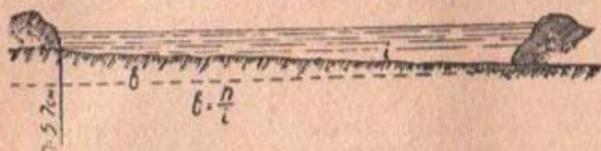
Рис. 23. Зависимость ширины промывной делянки от уклона местности.
