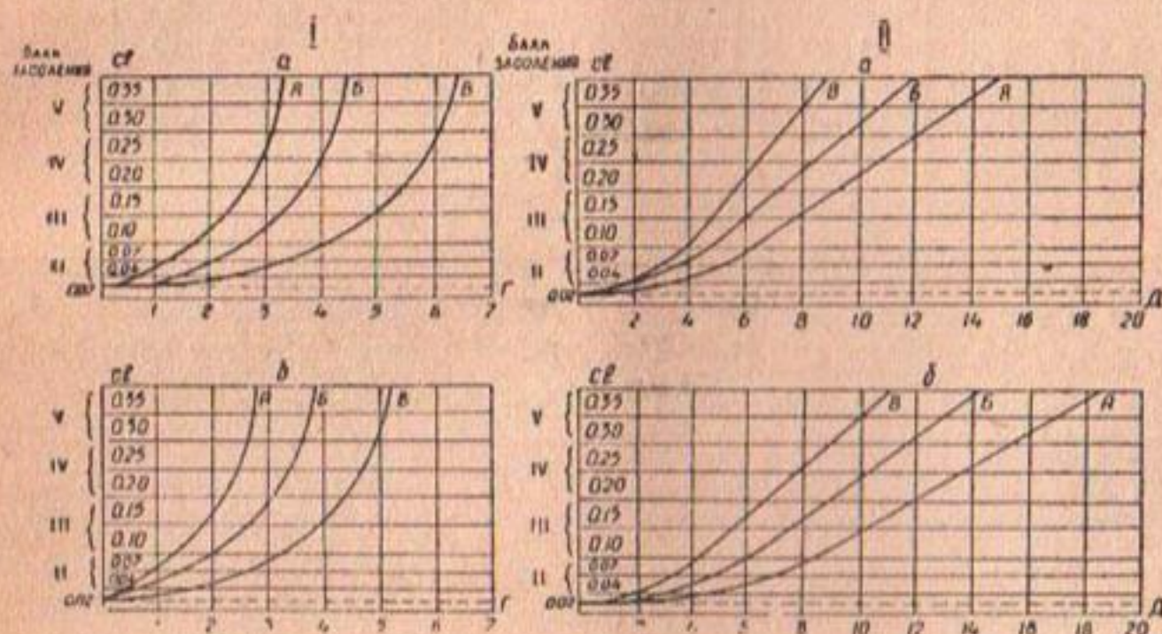
Рис. 17. Коэффициенты K и затраты воды ( \text{м}^3/\text{га} ), необходимые для опреснения земель в бездренажных условиях в зависимости от степени засоления почвы и исходной глубины залегания уровня грунтовых вод. Шкала — содержание хлора до промывки.
