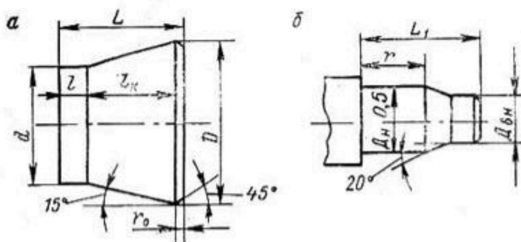
Рис. 7. Формовочные оправки для стыковки пластмассовых коллекторных труб:
