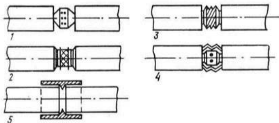
Рис. 2. Образцы пластмассовых соединительных муфт для керамического дренажа:
