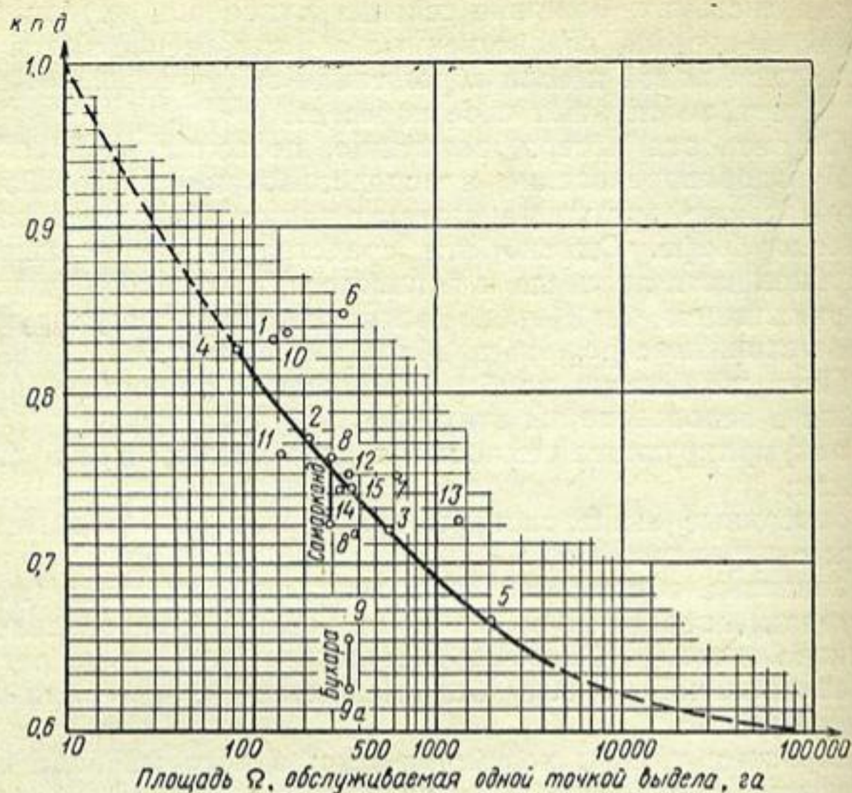
Рис. 28. Приближенная зависимость к.п.д. = f(\Omega) внутрихозяйственной сети из земляных каналов.
