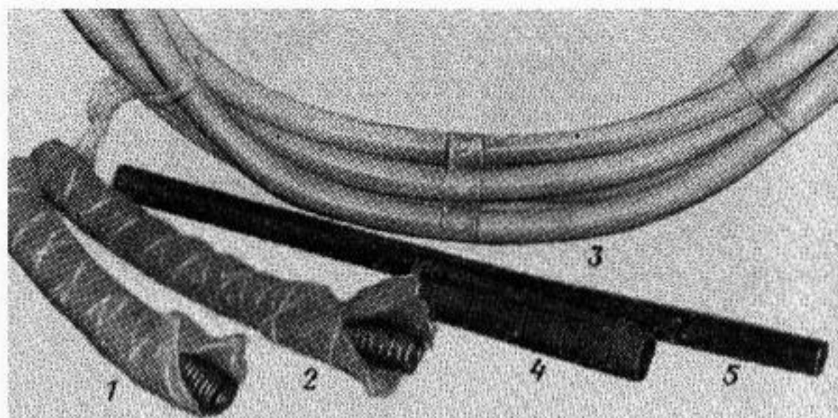
Рис. 5. Конструкции пластмассовых дренажных труб: 1, 2 — гофрированные трубы с оберткой рулонным ЗФМ; 3 — спиральнонавивные трубы ТДСВ; 4 — гофрированные трубы с перфорацией 1—1,5 мм; 5 — труба с мелкими гофрами
