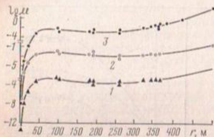
Рис. 6.7. Характер изменения логарифма коэффициента емкости (упругой водоотдачи) по радиусу депрессионной воронки в процессе опытных откачек из дренажной скв. 1 с дебитам 102 (1), 134 (2) и 164 м 3 /ч (3). Опыты 69—71
