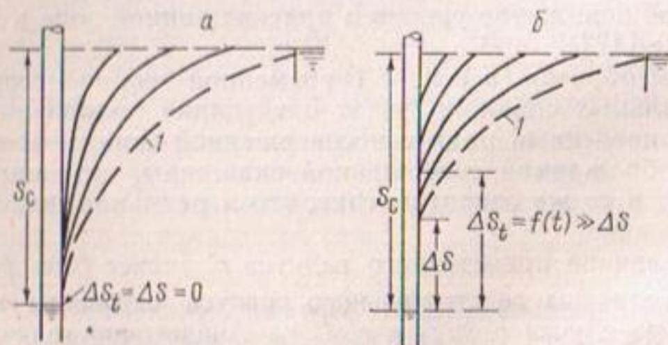
Рис. 2.1. Характер распространения воронки депрессии вблизи возмущающей скважины, пущенной в эксплуатацию с постоянным забойным давлением S_c = \text{const} : а — по В. Н. Щелкачеву; б — по автору; l — положение пьезометрической поверхности при стационарном режиме фильтрации
