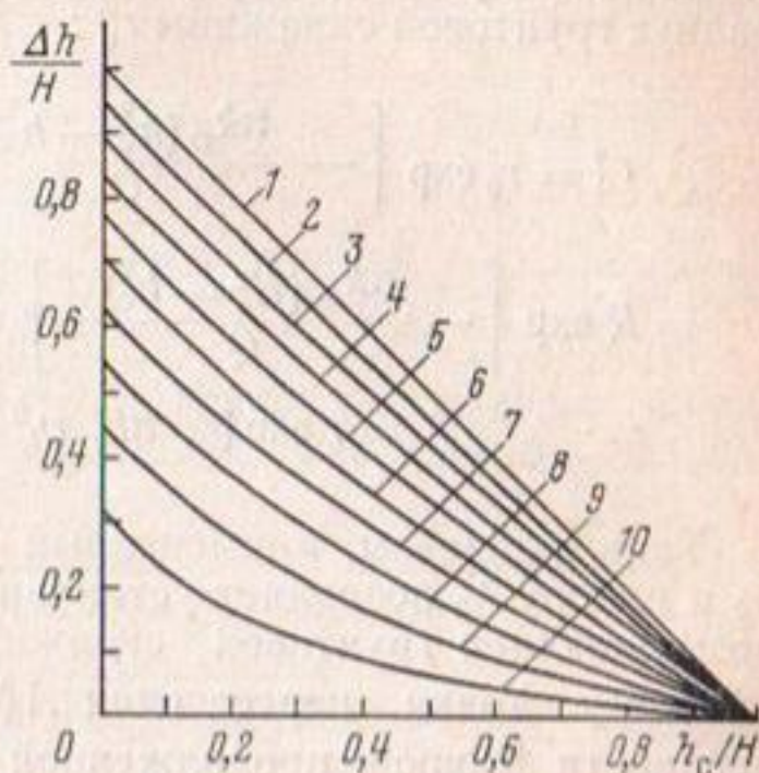
Рис. 2.9. Функция \Delta h/H = f(h_c/H) для значений \tau^* = 0 (1), 0,1 (2), 0,2 (3), 0,3 (4), 0,4 (5), 0,5 (6), 0,6 (7), 0,7 (8), 0,8 (9), 0,9 (10)
