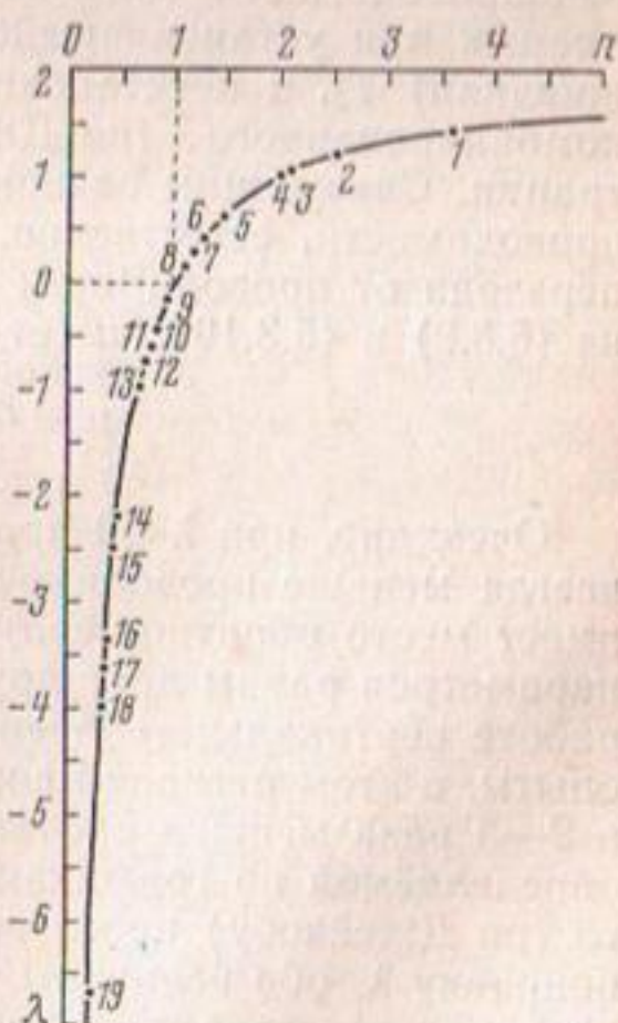
Рис. 5.21. Функция \lambda = 2(1 - 1/n) с экспериментальными значениями n и \lambda различных исследователей: 1 — [13]; 2 — откачка вблизи Элмвейла [138]; 3 — [27]; 4 — [14]; 5 — скв. 2 ц, Q = 180 \text{ м}^3/\text{сут} [82]; 6 — то же, Q = 134 \text{ м}^3/\text{сут} [82]; 7 — то же, Q = 240 \text{ м}^3/\text{сут} [82]; 8 — [107]; 9 — [110]; 10 — [114]; 11 — [8]; 12 — откачка вблизи Гранд Айслэнда [139]; 13 — скв. 3 ц, Q = 288 \text{ м}^3/\text{сут} [53, 57]; 14 — откачка вблизи Брэдфорда, Q = 55 \text{ фут}^3/\text{мин} [138]; 15 — откачка вблизи Скоттсблаффа (табл. 5.3); 16 — [119]; 17 — [18]; 18 — откачка в долине р. Арканзас, Q = 93 \text{ фут}^3/\text{мин} [135]; 19 — откачка на ферме Вортман, Q = 72 \text{ фут}^3/\text{мин} [136]
