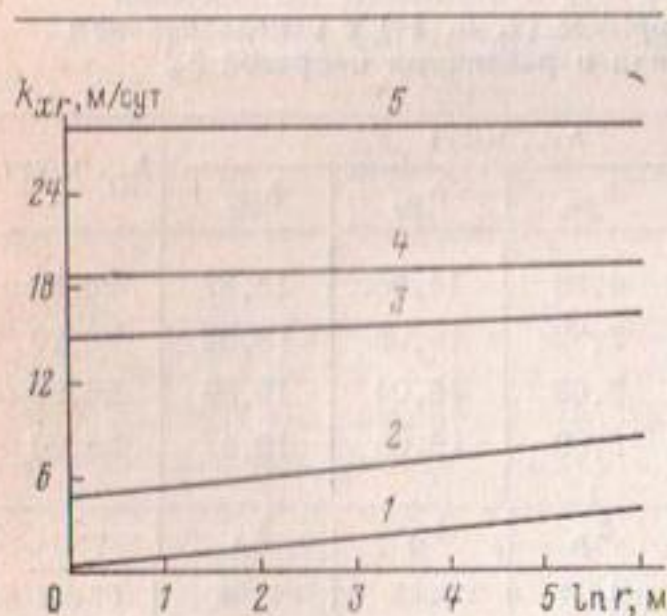
Рис. 2.7. Кривые k_{xr} = f(\ln r) для различных поправок (на несовершенство возмущающей скважины) к формуле Дюпюи \xi_x (построены по данным В. Н. Эмиха): 1 — k_{kr} , \xi_x = 0 ; 2 — k_{Br} , \xi_x = 10 ; 3 — k_{Яr} , \xi_x = 27,65 ; 4 — k_{Ar} , \xi_x = 35 ; 5 — k_D , \xi_x = 55,3 = \xi
