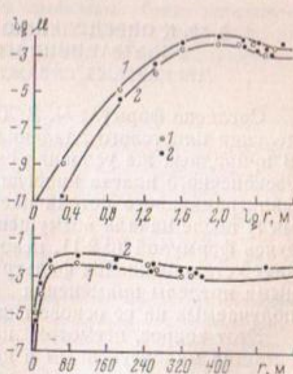
Рис. 6.11. Функции \lg \mu = f(r, \lg r) при восстановлении УГВ после остановок дренажной скв. 1, работавшей до остановок с дебитами 61 (1) и 164 м 3 /ч (2). Опыты 67 и 71
