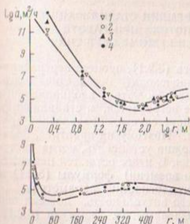
Рис. 6.10. Характер кривых \lg a = f(r, \lg r) при восстановлении УГВ после остановок дренажной скв. 1, работавшей до остановок с дебитами 32 (1), 61 (2), 102 (3) и 164 м 3 /ч (4). Опыты 66, 67, 69 и 71
