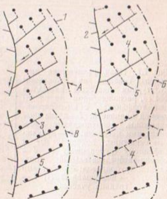
Рис. 7.6. Схемы крупных СВД: 1 — граница осушаемого массива; 2 — водоприемник; 3 — мелкие каналы сбросной сети; 4 — подземные трубопроводы проводящей сети; 5 — дренажные скважины
