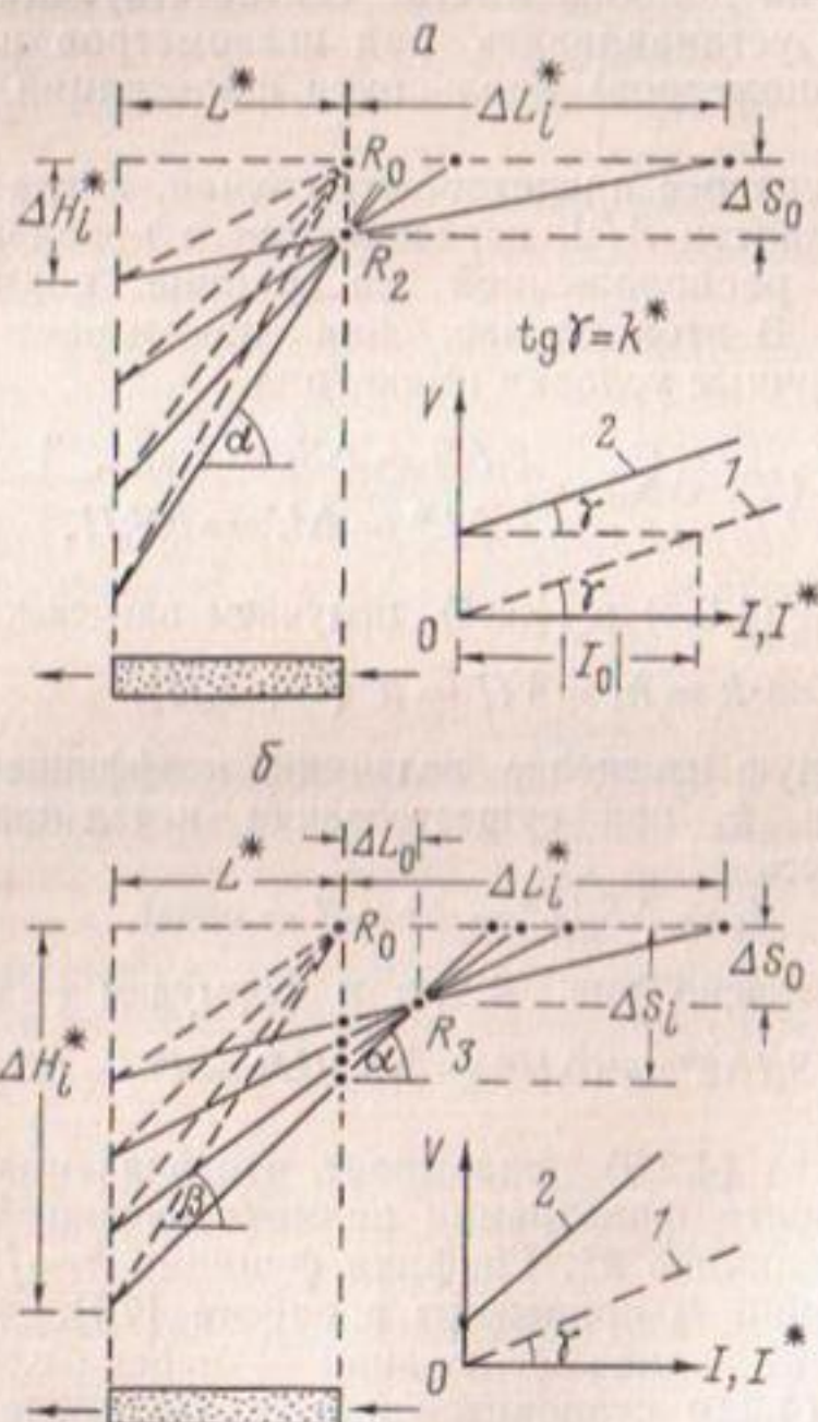
Рис. 4.4. Изображение устойчивых граничных условий R_0 и R_2 и соответствующих им кривых (а); то же для граничных условий R_0 и R_3 (б): 1 — V = f(I^*) ; 2 — V = f(I)
