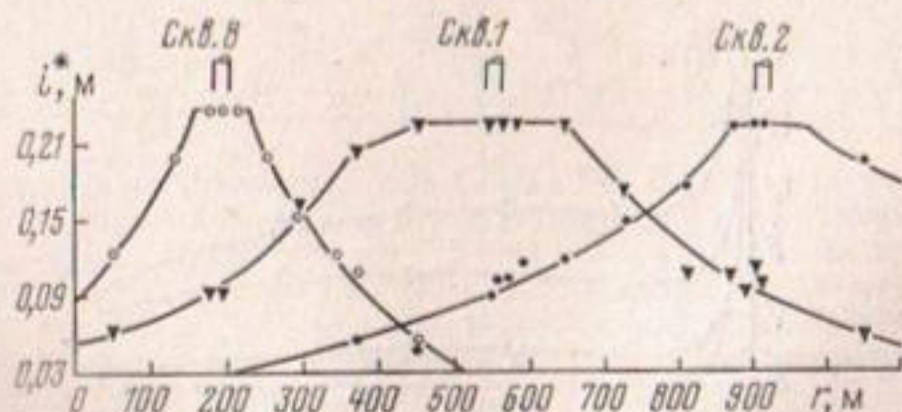
Рис. 6.2. Характер изменения параметра i^* = 0,183 Q/T по диаметру депрессионных воронок при опытных откачках из дренажных скв. 8, 1, 2, работавших с дебитами соответственно 105, 134 и 132 м 3 /ч (опыты 64, 70, 76)
