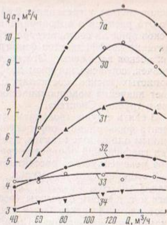
Рис. 1.13. Характер зависимости логарифма коэффициента уровне-проводности от дебита при опытных откачках из дренажной скв. 7. Цифры у кривых означают номера наблюдательных скважин
