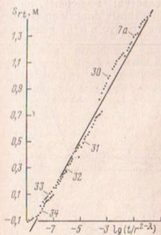
Рис. 7.9. Комбинированное (по автору) прослеживание снижения УГВ в наблюдательных скв. 7а—34 при пуске дренажной скв. 7 в работу с дебитом 60 \text{ м}^3/\text{ч} (опыт 45, \lambda = -1,6 )
