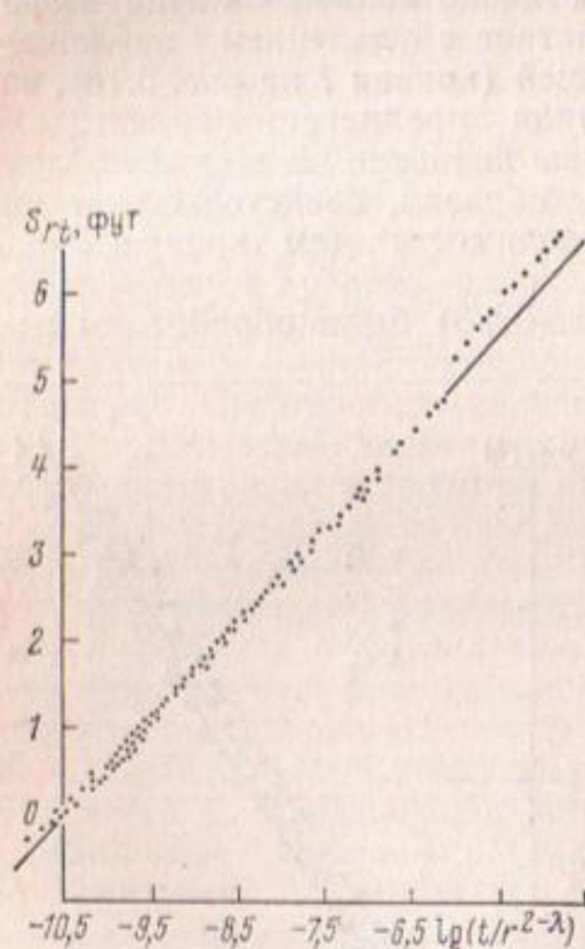
Рис. 5.26. Комбинированное (по автору) прослеживание снижения УГВ в различных наблюдательных скважинах при опытной откачке вблизи Скоттсблаффа (по данным Л. К. Венцеля [139]); \lambda = -2,5
