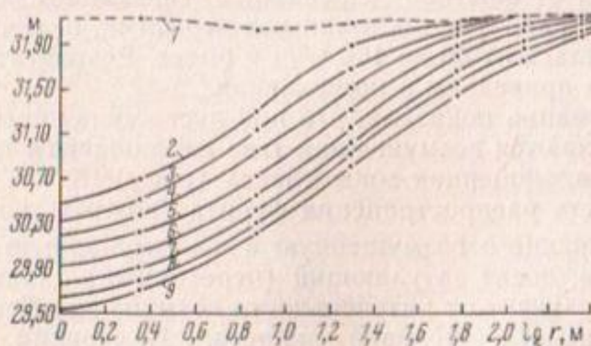
Рис. 5.1. Положение неустановившейся депрессионной поверхности грунтовых вод в координатах S_{rt} — \lg r на различные моменты времени после пуска дренажной скв. 7 в работу с дебитом 125 м 3 /ч (опыт 22): положение статического уровня (1) и депрессионной поверхности спустя 1 (2), 2 (3), 4 (4), 10 (5), 20 (6), 60 (7), 180 (8) и 600 мин (9) после включения насоса в работу
