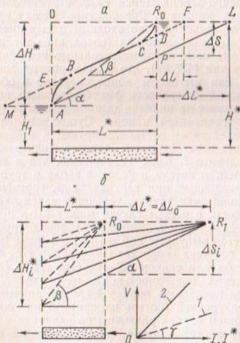
Рис. 4.2. Схема к расчету внутреннего ( I = \operatorname{tg} \alpha ) и внешнего ( I^* = \operatorname{tg} \beta ) градиентов давления при движении ньютоновских и аномальных жидкостей в приборе Дарси (а) и изображение устойчивых граничных условий R_0 и R_1 и соответствующих им законов Дарси (б): 1 — V = f(I^*) ; 2 — V = f(I)
