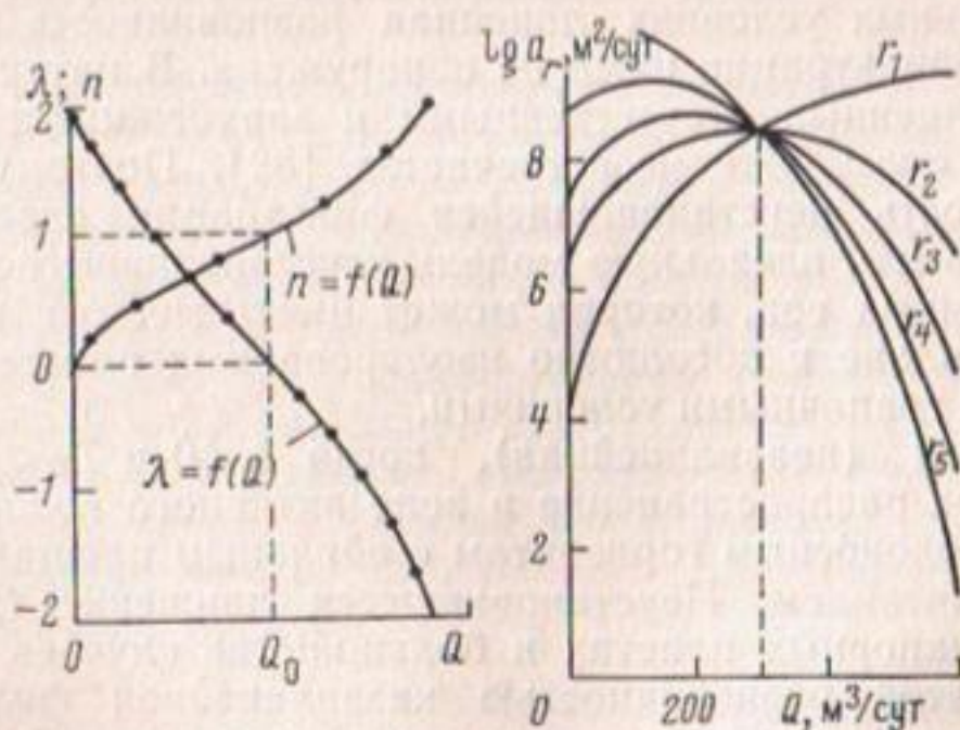
Рис. 5.14. Влияние интенсивности возмущения на изменение параметров \lambda , n , \lg a_r при режимах питания и разгрузки пласта, являющихся функцией интенсивности возмущения (по данным табл. 1 из [67, 76])
