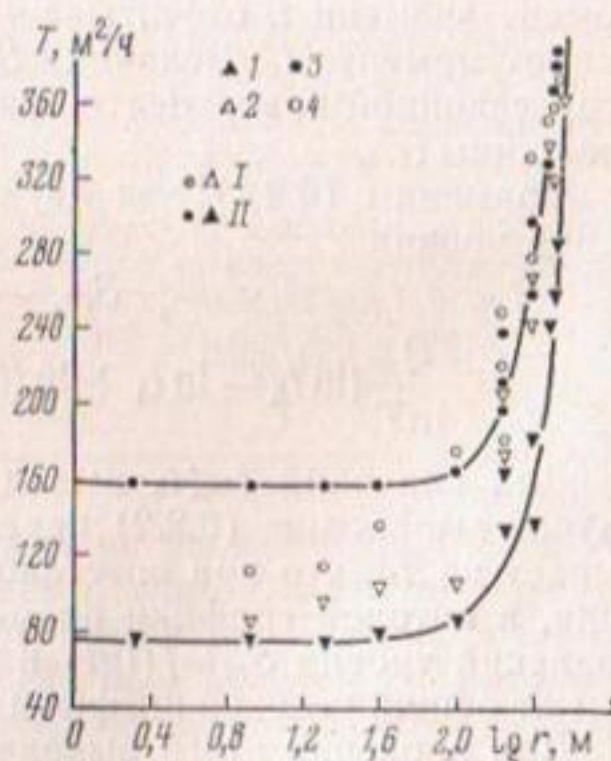
Рис. 6.9. Характер изменения по радиусу депрессионной воронки коэффициента водопроводимости при снижении (I) и восстановлении (II) уровня в процессе откачек из дренажной скв. 1 с дебитами 80 (1, 2) и 164 м³/ч (3, 4). Опыты 68, 71
