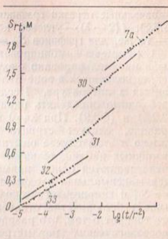
Рис. 5.24. Комбинированное (по Джейкобу) прослеживание восстановления УГВ после прекращения откачки из скв. 7, работавшей до остановки 24 ч с постоянным дебитом 125 м³/ч (опыт 22). Цифры у кривых означают номера наблюдательных скважин
