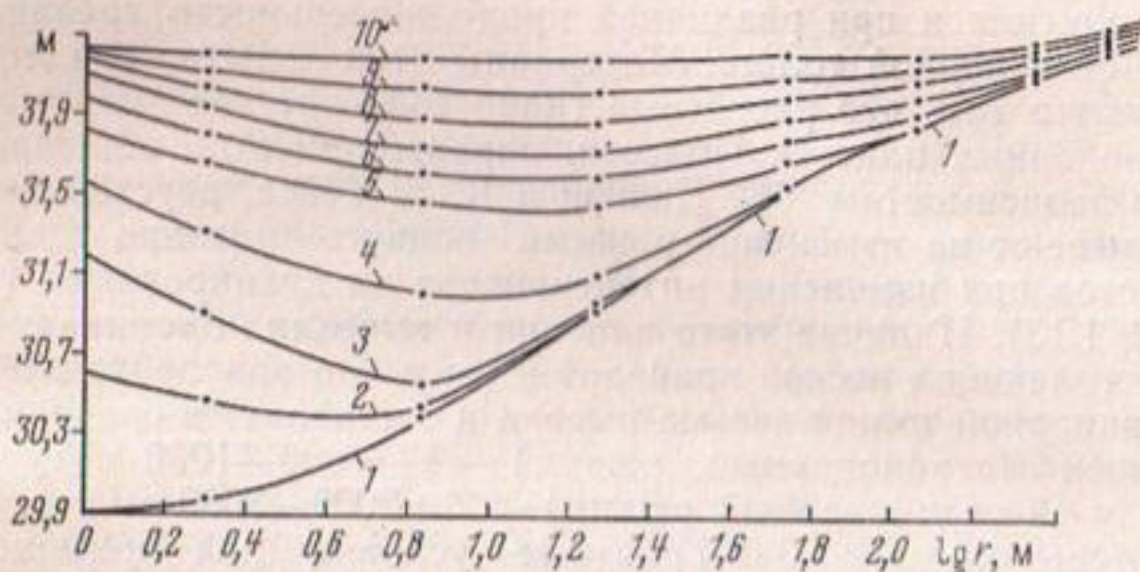
Рис. 1.3. Характер восстановления депрессионной поверхности в координатах S_{rt}-\lg r на различные моменты времени после прекращения откачки из скв. 7, работавшей до остановки 24 ч с дебитом 110 \text{ м}^3/\text{ч} (опыт 20). Положение кривой депрессии в момент остановки (1) и через 1/6 (2), 1/3 (3), 1 (4), 6 (5), 20 (6), 60 (7), 180 (8), 420 (9) и 1200 мин (10) после остановки скв. 7
