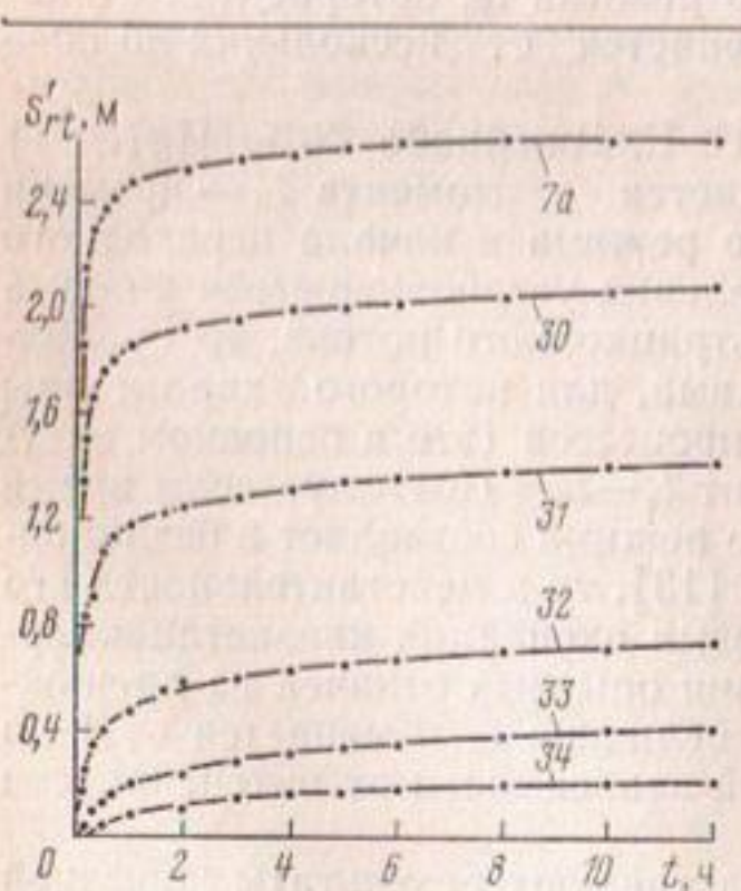
Рис. 5.20. Характер снижения УГВ во времени в различных наблюдательных скважинах при опытной откачке из дренажной скв. 7, пущенной в работу с дебитом 145 м 3 /ч (опыт 23). Цифры у кривых означают номера наблюдательных скважин
