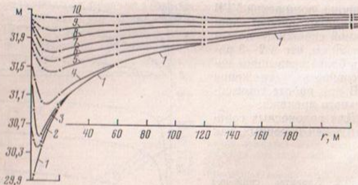
Рис. 1.4. Положение неустановившейся депрессионной поверхности в координатах S_{rt}-r на различные моменты времени после прекращения откачки из скв. 7, работавшей до остановки 24 ч с дебитом 110 \text{ м}^3/\text{ч} (опыт 20). Положение кривой депрессии в момент остановки (1) и через 1/6 (2), 1/3 (3), 1 (4), 6 (5), 20 (6), 60 (7), 180 (8), 420 (9) и 1200 мин (10) после остановки скв. 7
