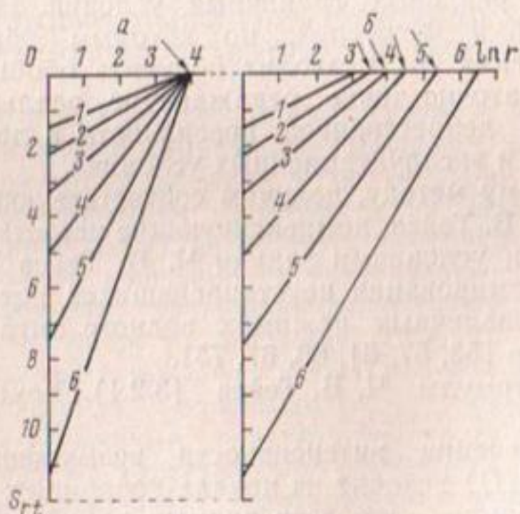
Рис. 5.9. Расположение не установившихся депрессионных поверхностей S_{r,t} = f(\ln r) на один и тот же момент времени: a — согласно формуле (3.2.1), \lambda_{1-6} = 0 , R_t = \text{const} \neq f(Q) ; b — согласно обобщенной формуле (5.3.17), учитывающей водобалансовую поправку \lambda : \lambda_{1-2} < 0 ; \lambda_3 = 0 ; \lambda_{4-6} > 0 ; R_t = f(Q) . Номера депрессионных поверхностей 1, 2, 3... соответствуют величинам дебита соответственно Q_1 , Q_2 = 1,5 Q_1 , Q_3 = 1,5 Q_2 и т. д.
