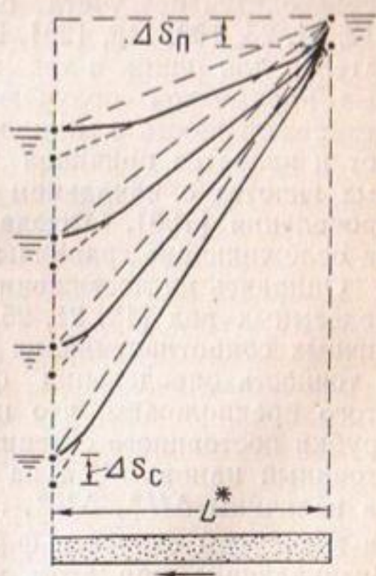
Рис. 4.1. Характер установившихся пьезометрических поверхностей (сплошные линии), формирующихся в пермеаметре при граничном условии R_0 , когда величина потерь напора на входе в трубку равна величине восстановления напора на выходе из трубки: I^*=I , |\Delta S_c| = |\Delta S_\pi|
