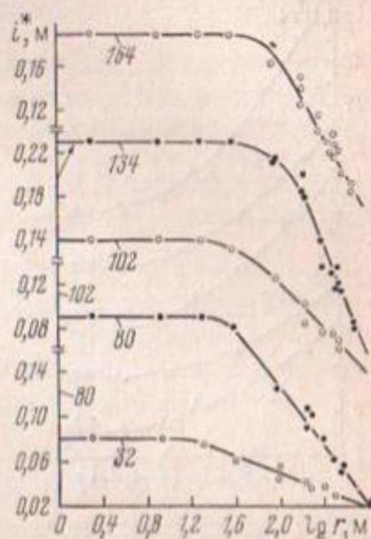
Рис. 6.1. Характер изменения параметра i^* = 0,183 Q/T по радиусу депрессионной воронки при откачках из дренажной скв. 1. Цифры у кривых означают дебит скважины в м 3 /ч
