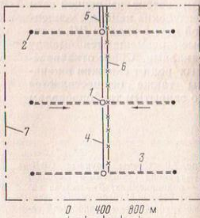
Рис. 7.7. План размещения дренажных скважин на орошаемом культурном пастбище площадью 484 га, расположенном на низинных торфяниках с высокопроницаемой подпочвой: 1 — дренажные скважины, оборудованные артезианскими насосами; 2 — дренажные скважины, подключаемые к сифонному трубопроводу 3; 4 — сборно-распределительный подземный трубопровод; 5 — сбросный канал; 6 — воздушная ЛЭП; 7 — граница участка
