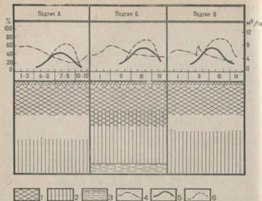
Рис. 13. I тип водного режима почвы: 1 — зона увлажнения осадками и поливами; 2 — зона увлажнения грунтовыми водами; 3 — грунтовые воды; 4 — влажность почвы; 5, 6 — суммарное водопотребление фактическое и расчетное.
