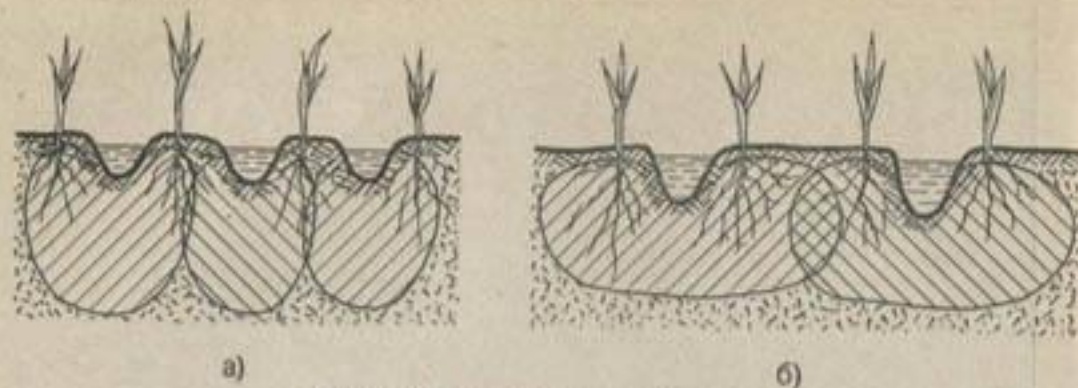
Рис. 8. Контуры увлажнения: а — на легких и б — на тяжелых почвах.
