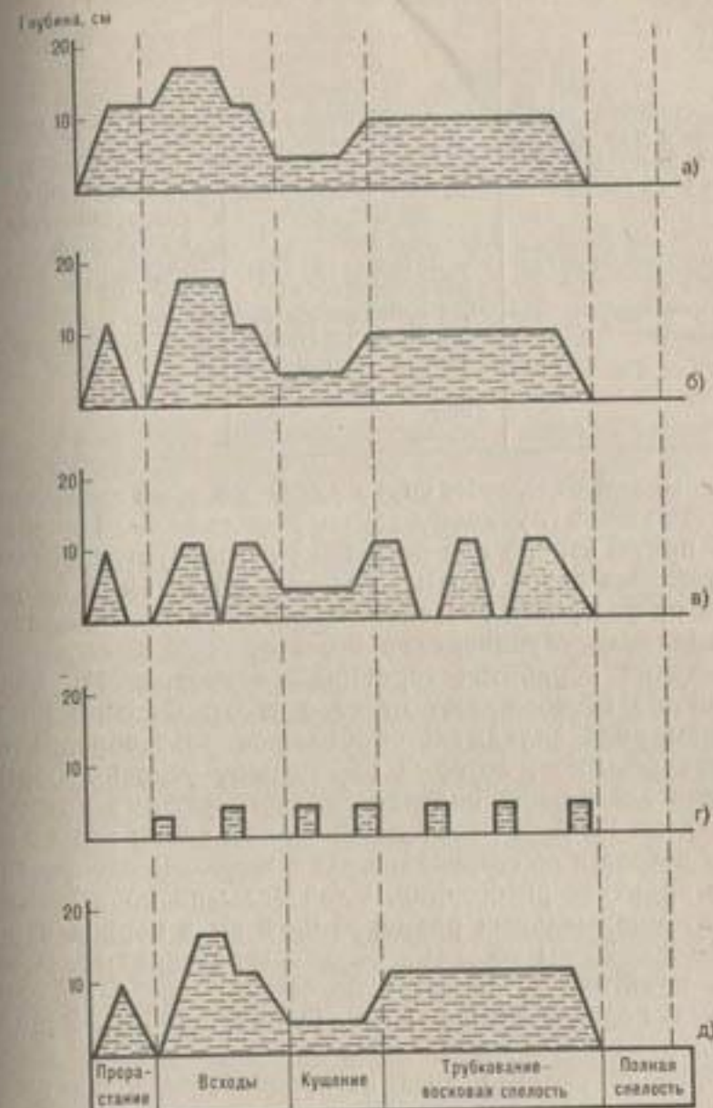
Рис. 14. III тип водного режима почвы:
