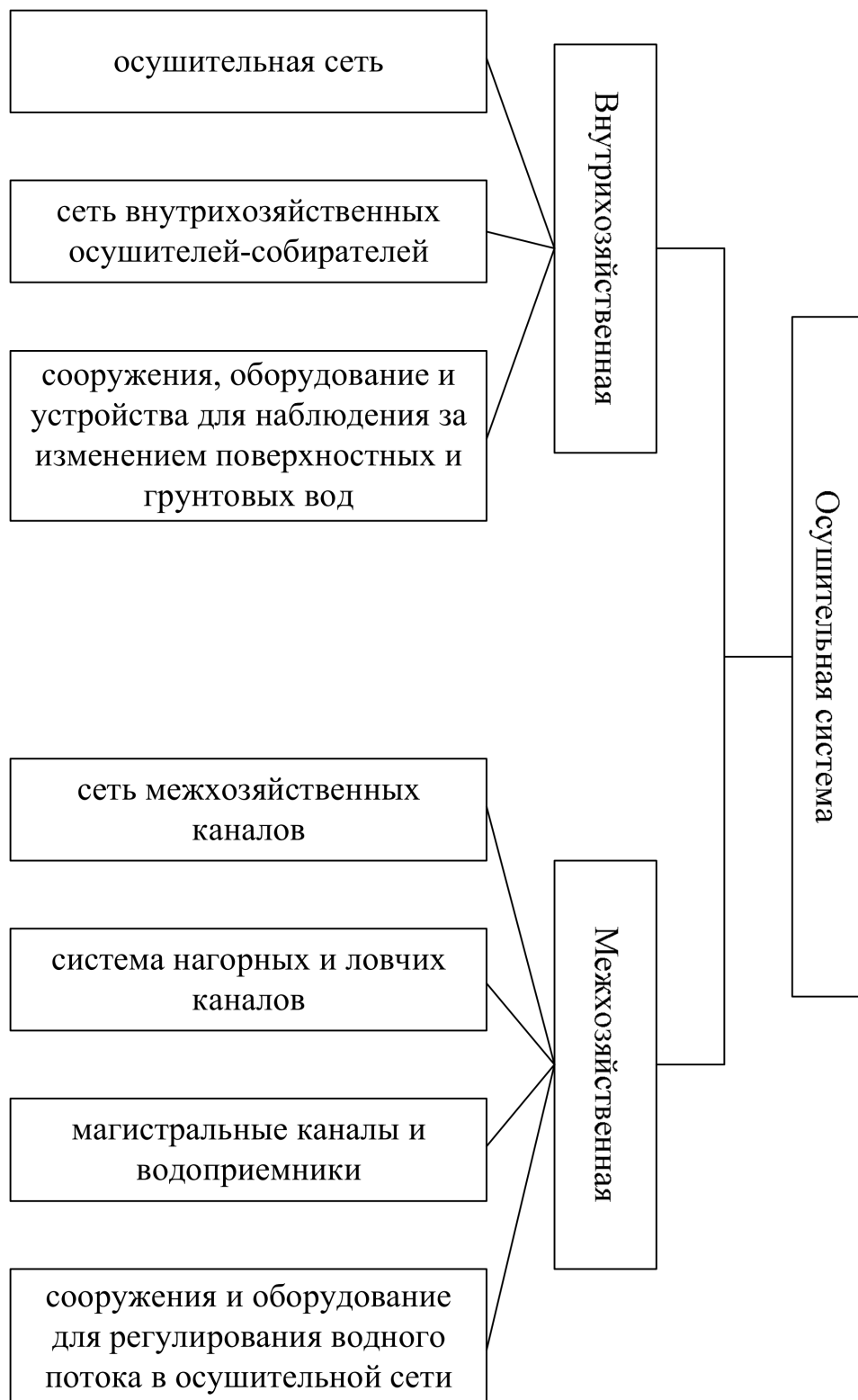
Рисунок 28 – Состав осушительной системы согласно В. А. Шумянцу
