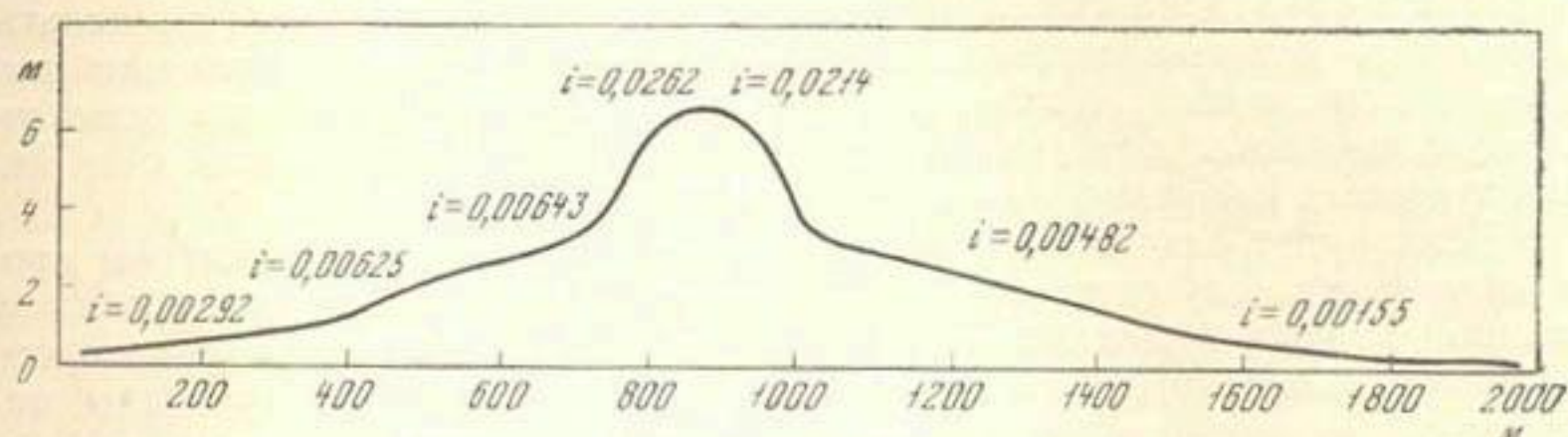
Рис. 22. Поперечный профиль вала в 2,5 км к юго-западу от Мессариана ( i -уклоны поверхности вала, в тысячных)
