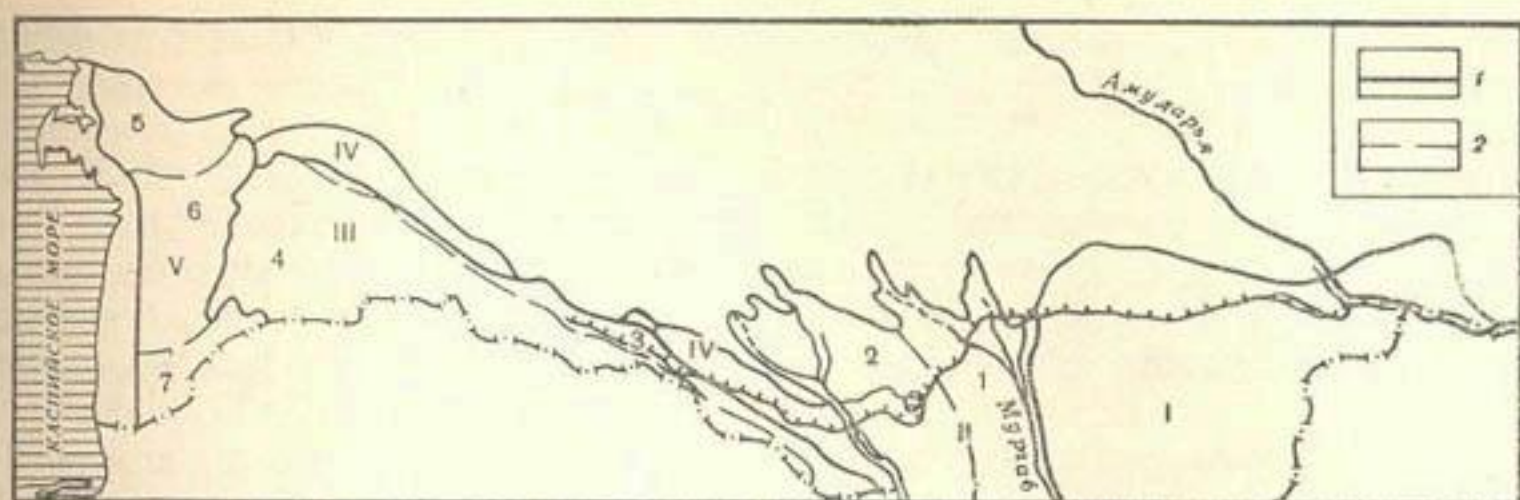
Рис. 9. Агроклиматическое районирование
