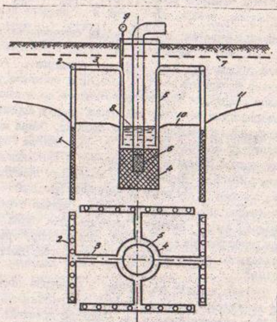
Рис.48. Конструкция вертикальной дрены с сифонными усилителями.
