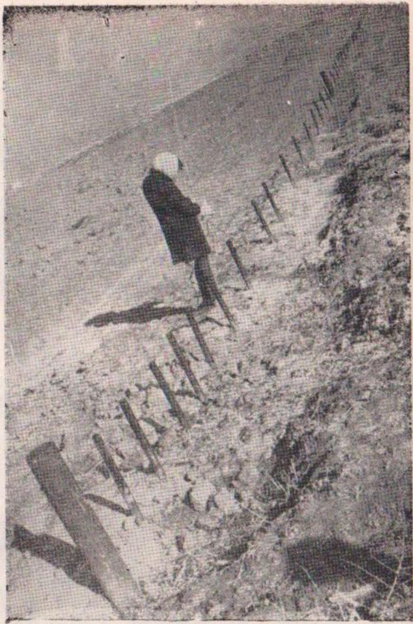
Рис. 11. Створ наблюдательных скважин и пьезометров.
