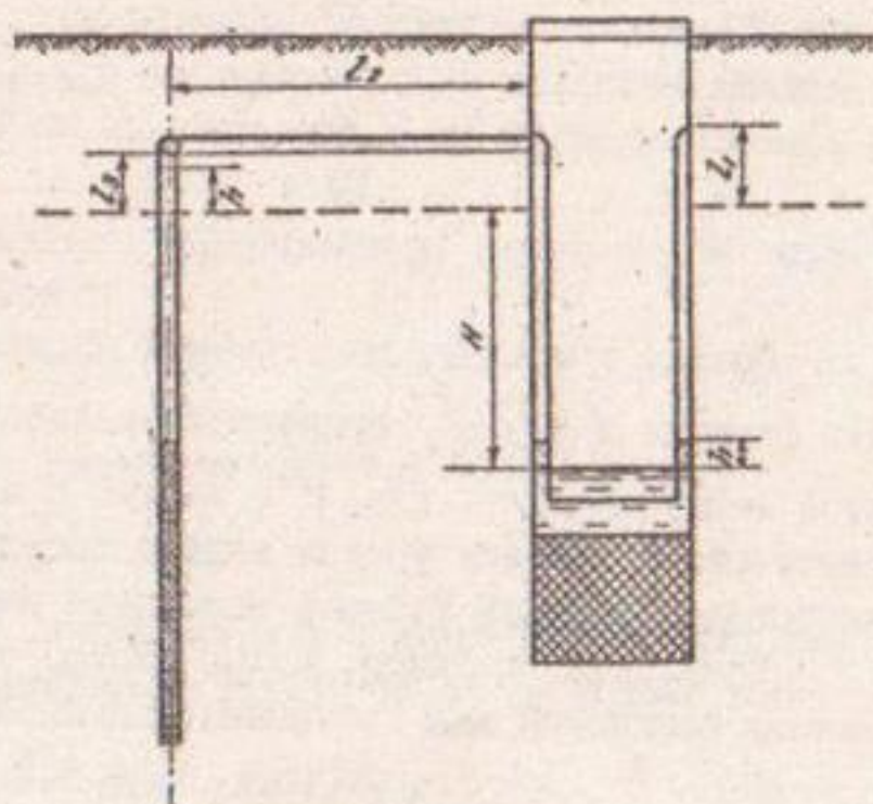
Рис.33. Схема для расчета зарядки сифонной линии.
