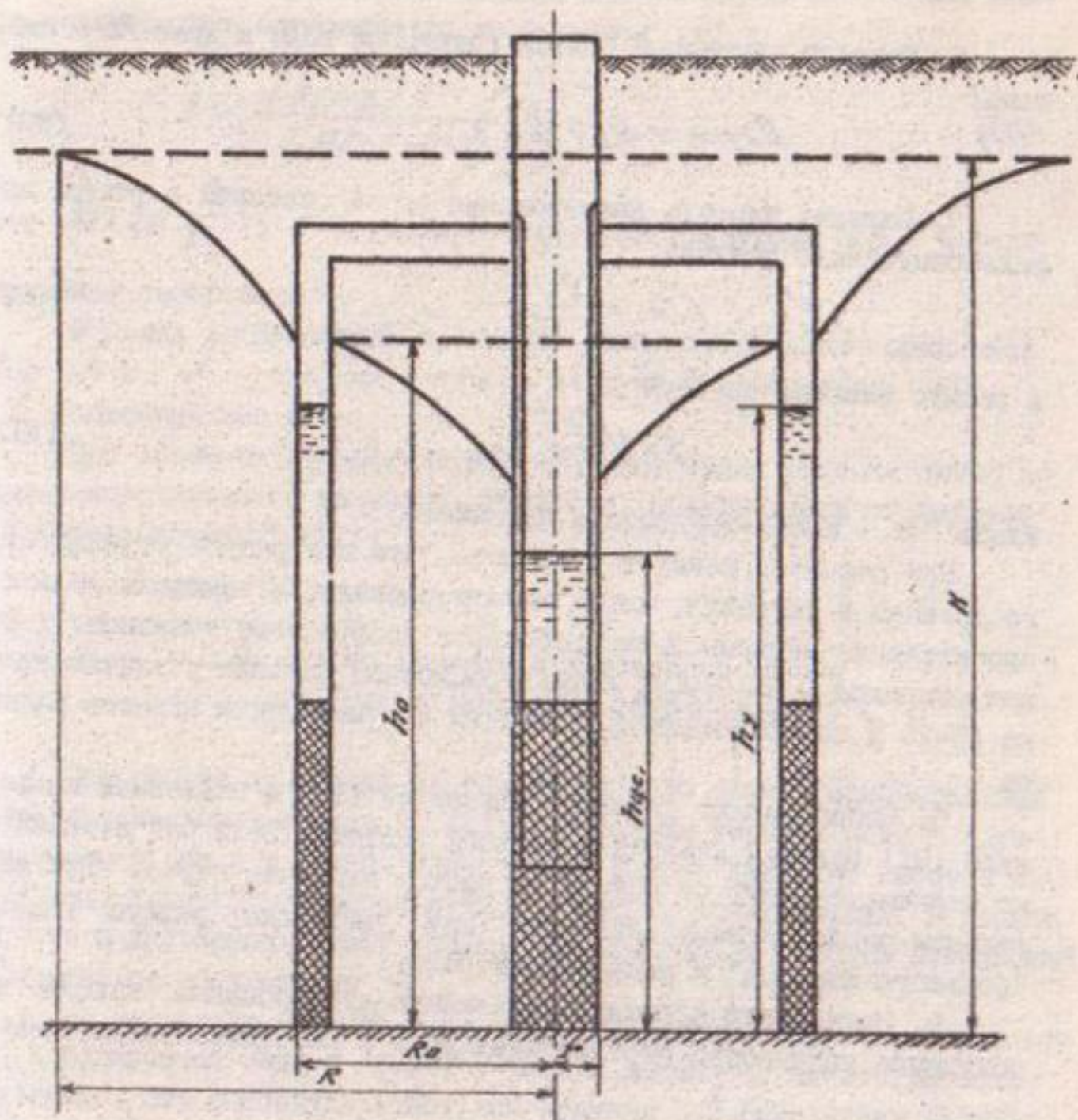
Рис.44. Схема для расчета вертикальной дрени с сифонными усилителями.
