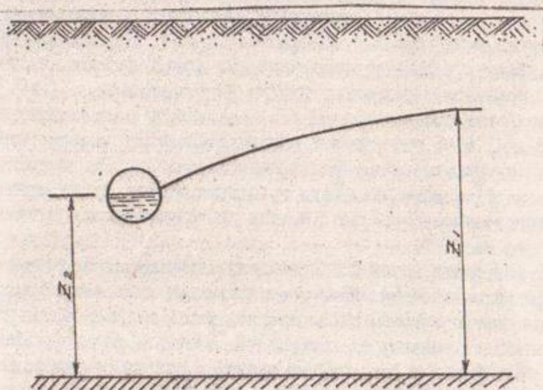
Рис.9. Схема понижения уровня грунтовых вод при работе дренажа.
